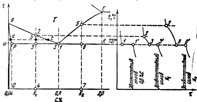
Рис. 140. Часть диаграммы состояния Fe—C. Вторичная кристаллизация сталей
