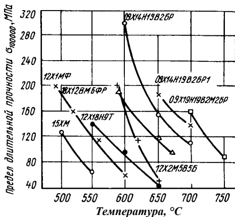
Рис. 335. Зависимость длительной прочности (100 000 ч) котельных сталей от температуры
