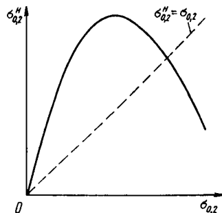
Рис. 58. Предел текучести гладкого ( \sigma_{0.2}^г ) и надрезанного ( \sigma_{0.2}^н ) образцов
