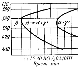
Рис. 426. Диаграмма изотермического распада р-фазы в алюминиевой бронзе
