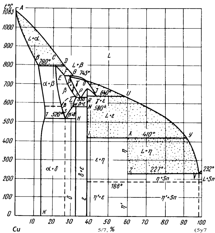
Рис. 421. Диаграмма состояния Си—Бп
