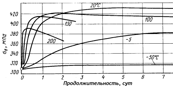
Рис. 396. Кривые старения дюралюминия при различных температурах
