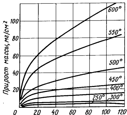
Рис. 365. Окисление титана при различных температурах
