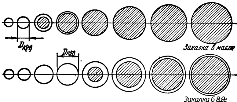
Рис. 234. Прокаливаемость прутков различного размера при закалке в воде и масле (заштрихована незакаленная сердцевина)
