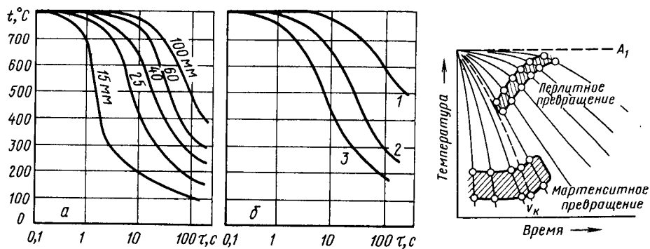
Рис. 194. Кривые охлаждения центра цилиндрических образцов:
