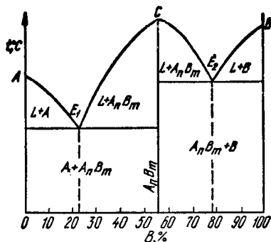
Рис. 101. Диаграмма состояния в устойчивом химическом соединении
