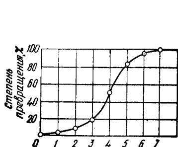
Рис. 29. Кинетическая кривая кристаллизации
