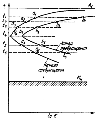
Рис. 186. Диаграмма изотермического превращения аустенита (построена по кривым изотермического превращения на рис. 181))
