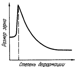
Рис. 75. Размер зерна после кристаллизации в зависимости от степени предшествующей деформации (схема)
