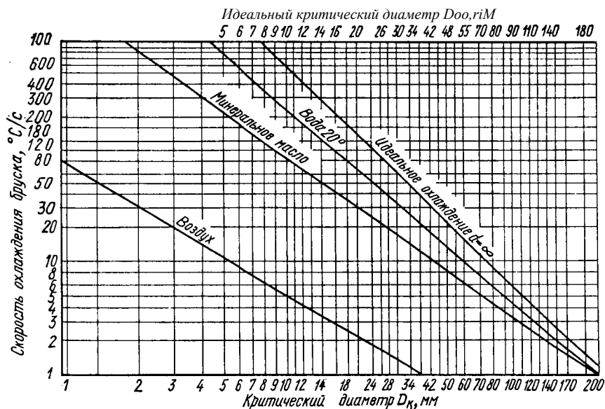
Рис. 235. Номограмма для определения прокаливаемого»
