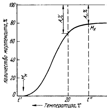
Рис. 199. Мартенситная кривая
