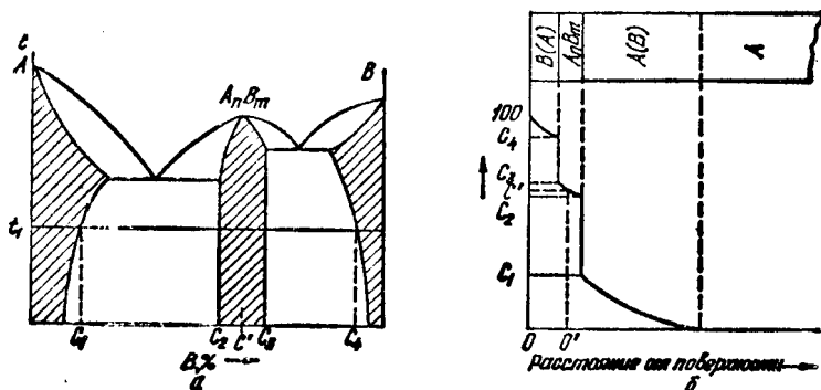
Рис. 266. Система сплавов «ограниченное растворимостью» химическими соединениями:
