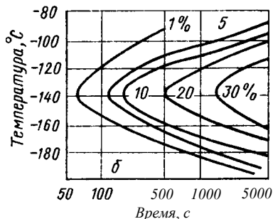
Рис. 212. Изотермическое превращение аустенита в мартенсит (сплав \text{Re}-23\% \text{Ni}-3\% \text{Mn} ) при разных температурах (а) и диаграмма изотермического превращения (б) (цифры у кривых — степень превращения)
