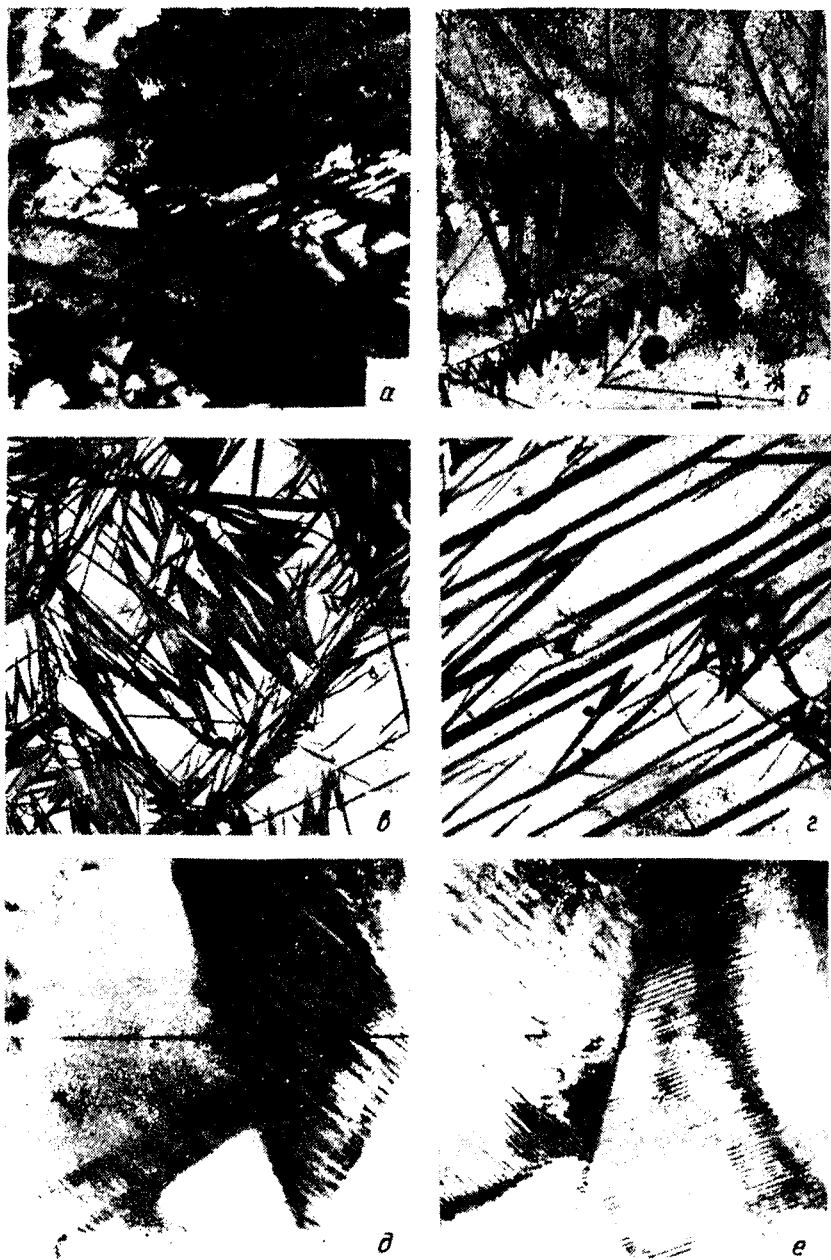
Рис. 204. Структура пластинчатого (двойникового) мартенсита: a — частично двойникованный. X300; б — г — полностью двойникованный, X 400; д , е — полностью двойникованный мартенсит (просвечивающая электронная микро- скопия, X 20 000
