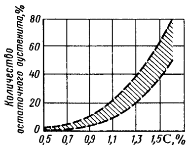
Рис. 201. Зависимость количества остаточного аустенита от содержания углерода (заштрихованная полоса учитывает возможность разных условий охлаждения в интервале M_u - M_s )
