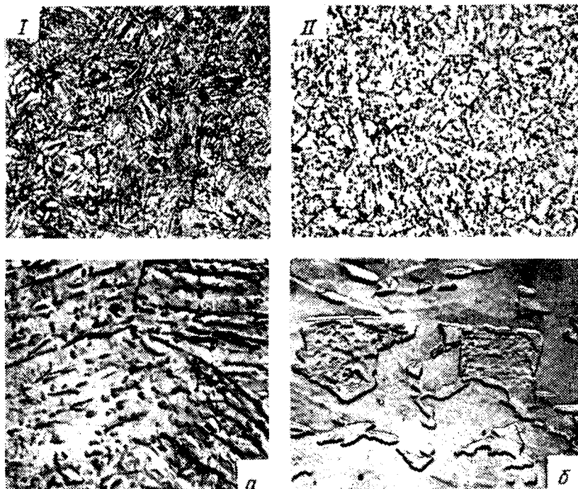
Рис. 217. Структура бейнита (левые фотографии — нижний бейнит, правые — верхний бейнит; верхние фотографии — световая микроскопия, X 500; нижние — электронная микроскопия, X3000)
