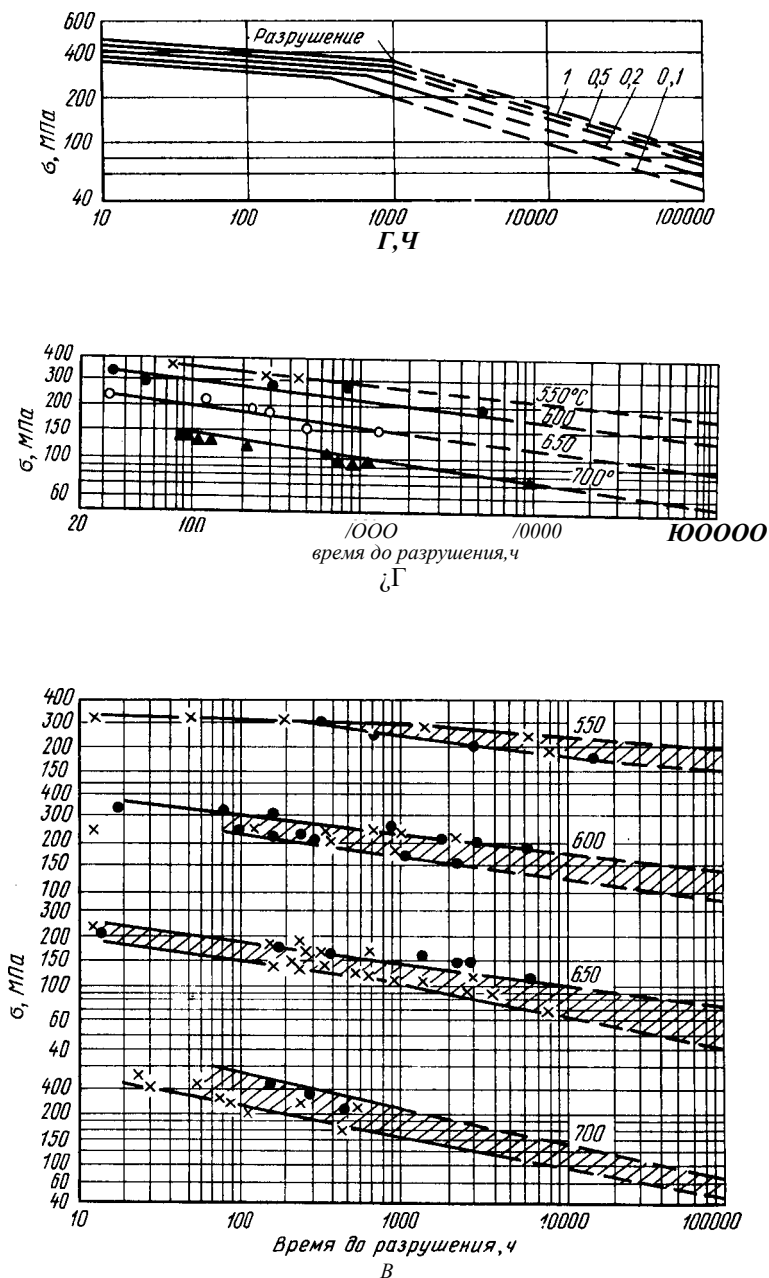
Рис. 331. Графики жаропрочности:
