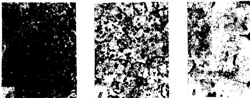
Рис. 405. Микроструктура дюралюминия:
