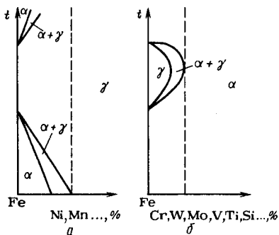
Рис. 272. Диаграммы состояния железо — легирующий элемент
