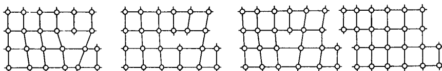
Рис. 14. Схема сдвиговой деформации, осуществляемой скольжением краевой дислокации
