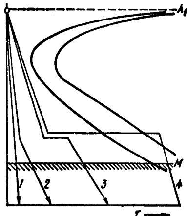
Рис. 242. Влияние температуры и продолжительности отпуска стали с 0,3 % C на остаточные напряжения
