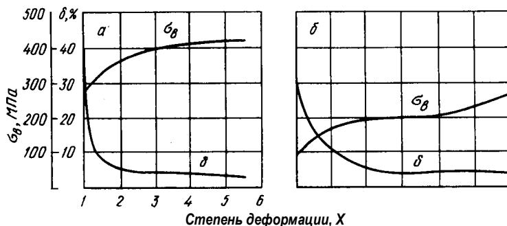
Рис. 66. Изменение механических свойств меди (а) и алюминия (б) в зависимости от степени пластического* деформации
