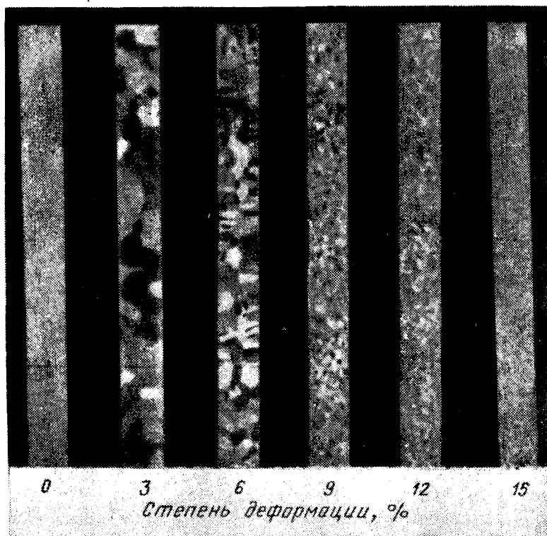
Рис. 76. Макроструктура алюминия после рекристаллизации в зависимости от степени деформации, % (указана у структур)
