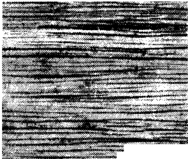
Рис. 370. Микроструктура молибдена в рекристаллизованном состоянии
