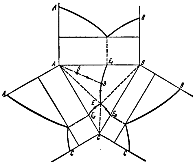
Рис. 120. Диаграмма состояния трехкомпонентной системы. Компоненты нерастворимы в твердом состоянии и образуют тройную эвтектику (развертка)
