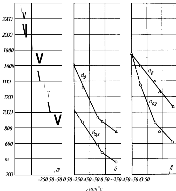
Рис. 354. Пределы прочности и текучести аустенитных сталей (образцы с надрезом) при различных температурах испытаний: а — 12Х18Н10; б — 12Х18Н20; е — 12Х18АГ19
