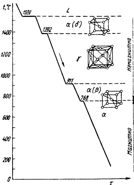
Рис. 39. Кривая охлаждения железа
