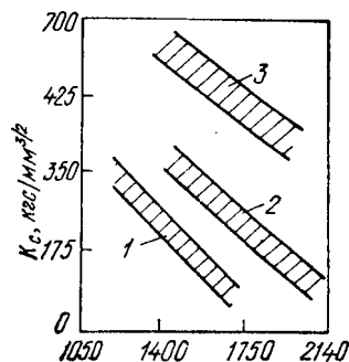
Рис. 297. Вязкость разрушения высокопрочных сталей: 1 — 30XНЗМ; 2 — мартенсит-настающая; 3 — трип-сталь
