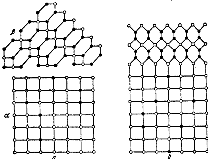
Рис. 111. Схемы сочленения кристаллических решеток: \alpha — несвязанная; \beta — связанная (когерентная)
