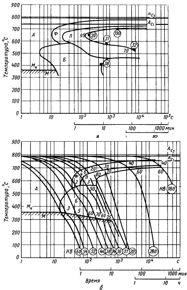
Рис. 196. Диаграмма изотермического (а) и анизотермического (термо-кинетического) (б) превращений аустенита в стали 45Х (Ф. Вефер). Цифры в кружках — твердость продуктов распада (НВС); цифры без кружков — количество структурной составляющей после превращения
