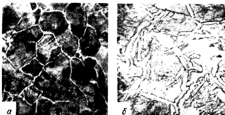
Рис. 260. Микроструктура заэвтектодного слоя, X 600 а — нормальная; б — аномальная
