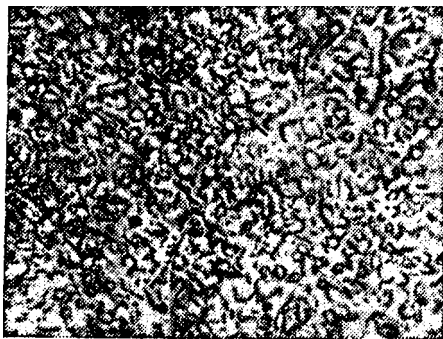
Рис. 302. Структура стали ШХ15 после закалики и отпуска, \times 500
