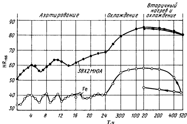
Рис. 267. Изменение твердости железа (Fe) и стали (38Х2МН0А) в процессе насыщения, последующего охлаждения и вторичного нагрева охлаждения
