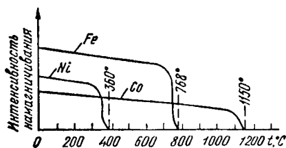
Рис. 40. Изменение магнитных свойств железа, никеля и кобальта в зависимости от температуры
