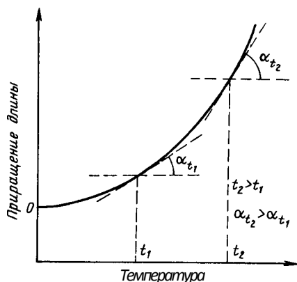
Рис. 378. Кривая расширения сплавов при повышении температуры
