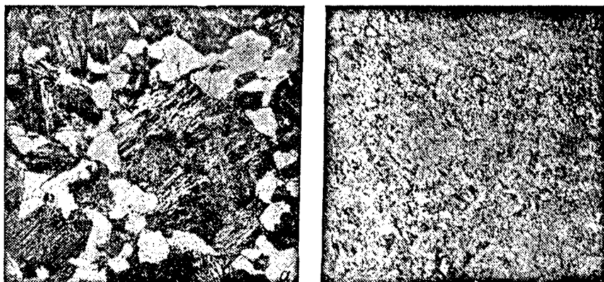
Рис. 293. Структура стали 30ХГСА, \times 500 :
