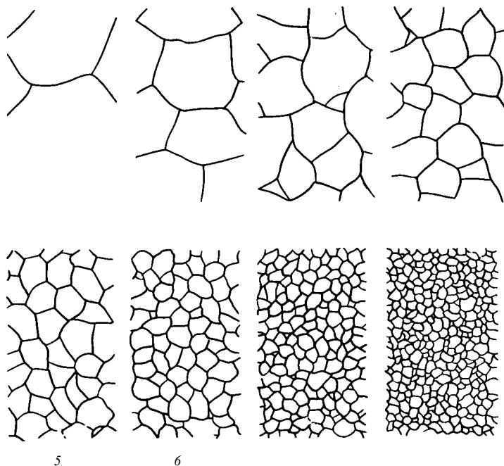
Рис. 180. Шкала размеров зерна, X 100
