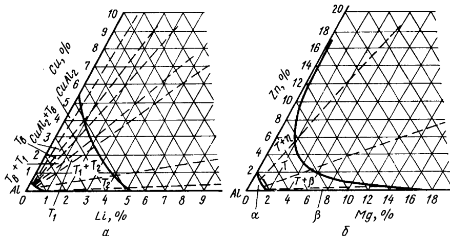
Рис. 402. Алюминиевый угол системы Al — Си—Ы (а) и системы Al— Me (б)
