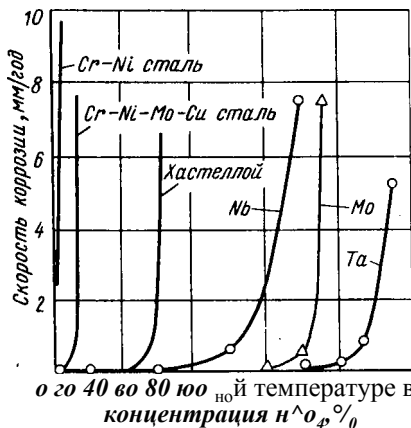
Рис. 353. Скорость коррозии различных металлов в кипящей серной кислоте
