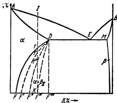
Рис. 110. Кристаллизация из твердого раствора в условиях переохлаждения
