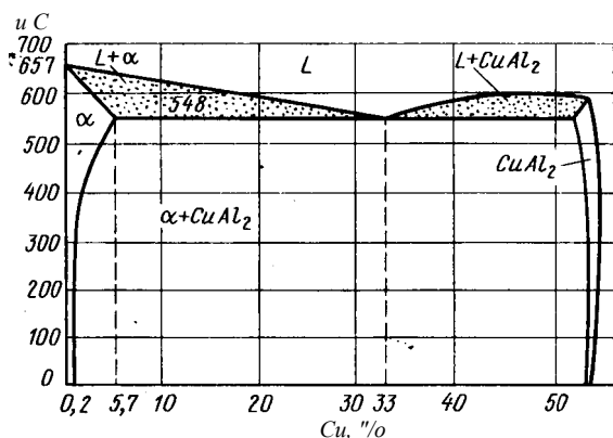
Рис. 392. Диаграмма состояния Al—
