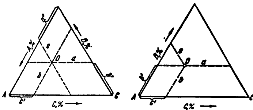
Рис. 116. Определение концентрации сплавов в равностороннем концентрационном треугольнике
