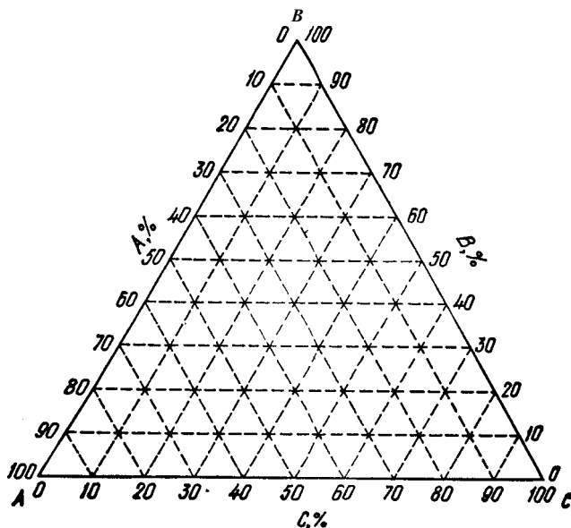
Рис. 114. Концентрационный треугольник (равносторонний)
