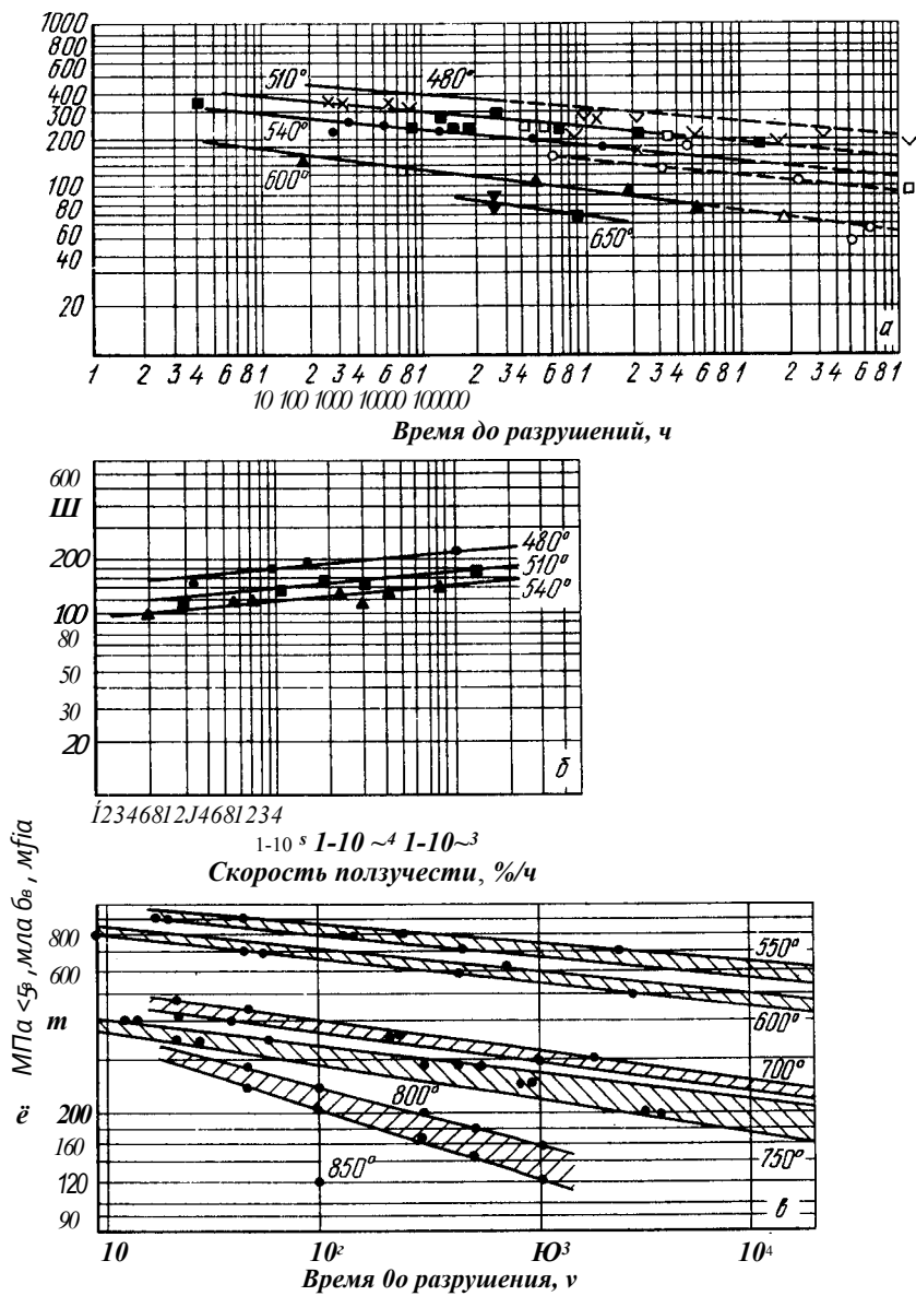
Рис. 334. Жаропрочные свойства стали 12ХМФ (а, б) и стали ХН35ВТЮ (в)
