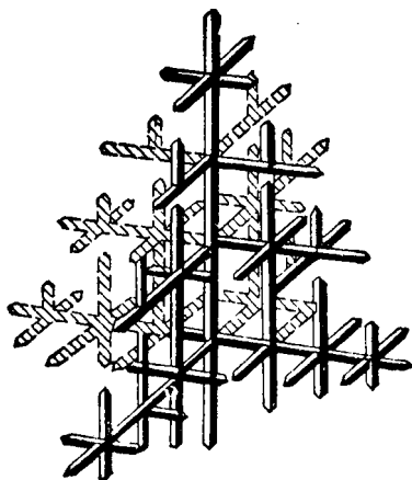
Рис. 32. Схема дендрита
