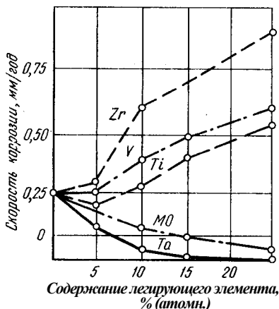
Рис. 377. Влияние легирующих элементов на коррозионную стойкость сплавов ниобия в кипящей 40%-ной H_2SO_4 .
