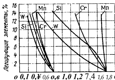
Рис. 288. Влияние легирующих элементов на положение точек S и E ОИДЫ и аучЛспИ!.
