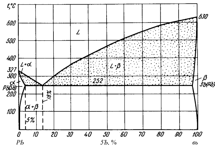
Рис. 431. Диаграмма состояния РЬ—БЬ
