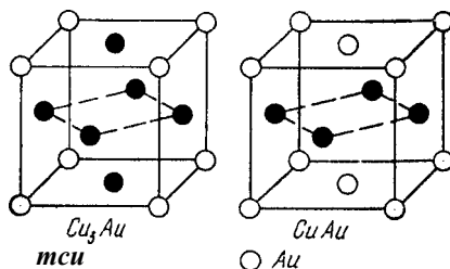
Рис. 88. Кристаллические решетки упорядоченных твердых растворов в системе \text{Cu}-\text{Au}
