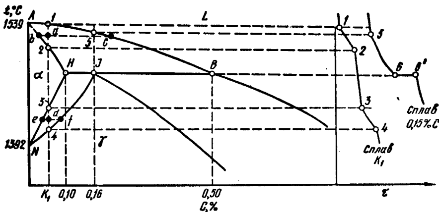
Рис. 138. Часть диаграммы состояния Fe—C. Первичная кристаллизация низкоуглеродистых сплавов
