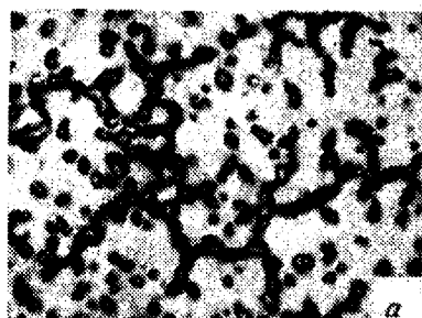
Рис. 412. Микроструктура сплава МЛ6, X 250:
