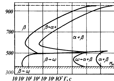
Рис. 364. Диаграмма изотермического превращения 3-фазы в сплавах Ti-J-8% Mo
