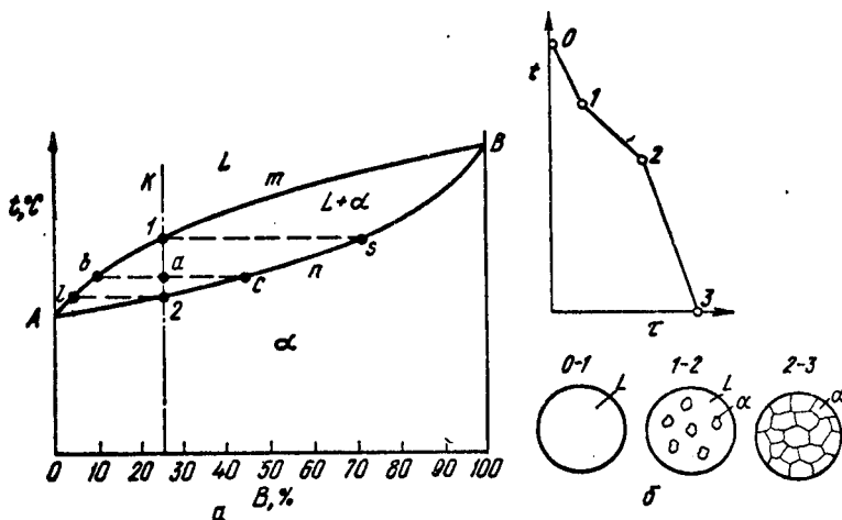
Рис. 96. Диаграмма состояния (неограниченная растворимость а в твердом состоянии) и хривая охлаждения
