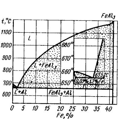
Рис. 389- Часть диаграммы состояния сплавов Al— Ре
