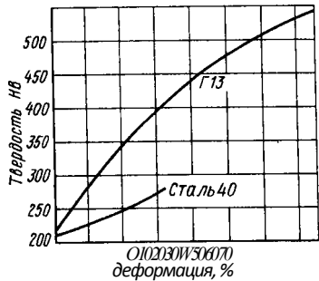
Рис. 358. Влияние наклепа на твердость углеродистой стали 40 и стали Г13
