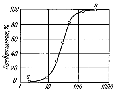
Рис. 184. Кинетическая кривая превращения аустенита в перлит
