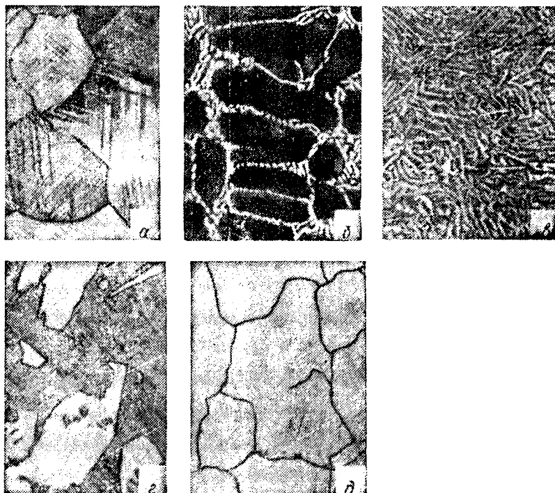
Рис. 94. Структура сплавов свинец — олово, X 100:
