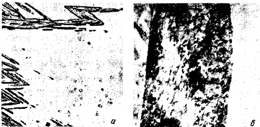
Рис. 213. Изотермический мартенсит (сплав \text{Fe}-\text{Ni}-\text{Mo} ) а — световая микроскопия, \times 400 ; б — просвечивающая электронная микроскопия, \times 30\,000
