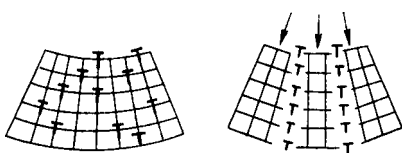
Рис. 88. Олбрачорание дислокационной сетк и (полнигонизация)
