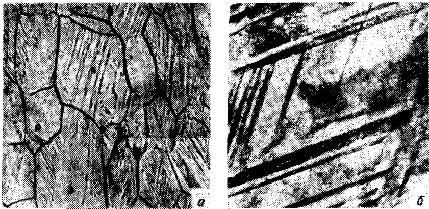
Рис. 357. Структура стали Гадфильда после деформации: а — световая микроскопия, Х400; б — электронная микроскопия, Х33000
