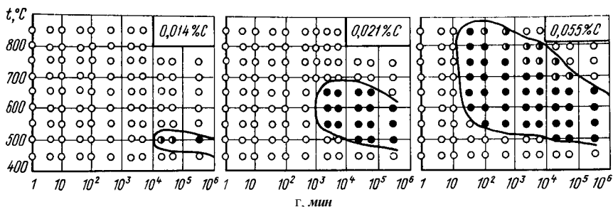
Рис. 352. Склонность к межкристаллитной коррозии аустенитной хромоникелевой стали 12X18H9 с различным содержанием углерода (светлые точки — не склонна к МКК; черные точки — склонна к МКК; наполовину светлые — мало склонна к МКК)
