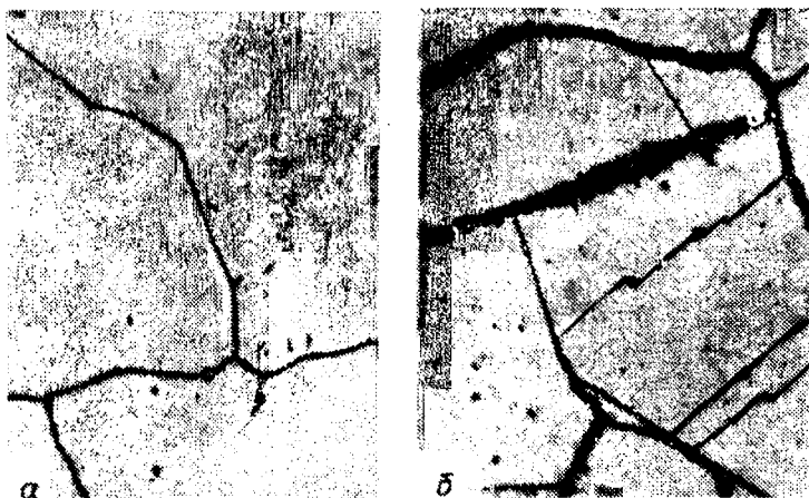
Рис. 336. Микроструктура аустенитной жаропрочной стали, X500: а — после закалки; б — после старения при 650 °С
