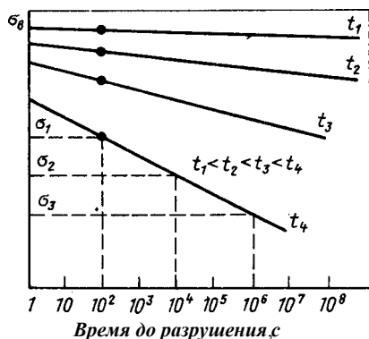
Рис. 327. Зависимость прочности от продолжительности испытания
