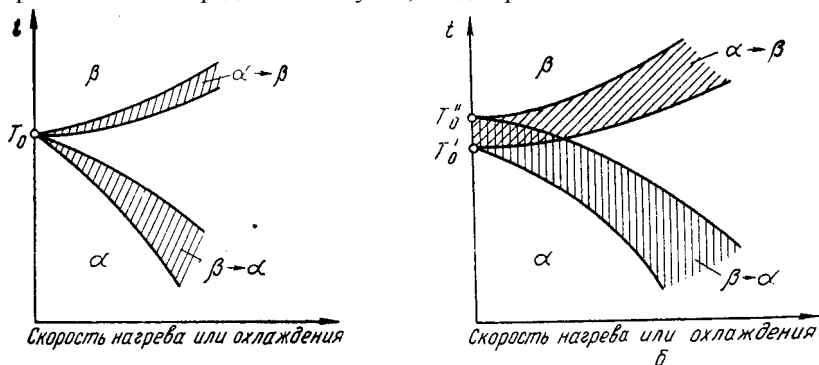
Рис. 106. Влияние скорости нагрева или охлаждения на температуры превращения: а — для систем с нулевой степенью свободы; б — для систем с одной или более степенями св.боды
