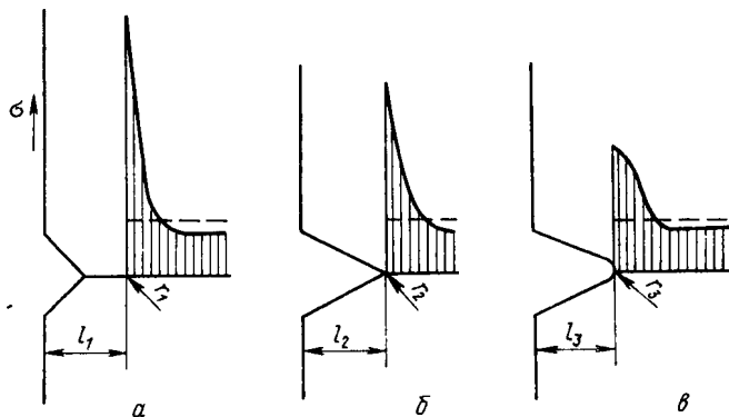
Рис. 51. Концентраторы напряжений в устье дефекта (штриховые линии a_{\text{теор}}/l, > l, > l, < l, < l );
