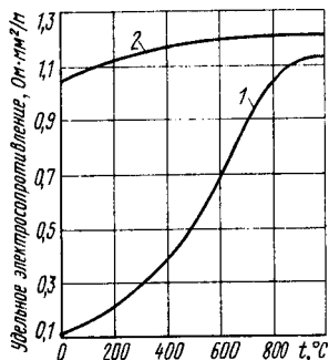
Рис. 386. Изменение электросопротивления железа (1) и никрома (2) при повышении температуры
