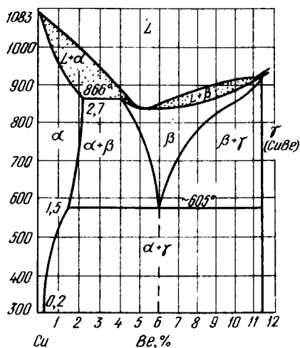
Рис. 428. Диаграмма состояния Си — Ве
