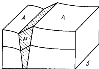
Рис. 197. Рельеф (а) на поверхности шпифа, возникающей в результате мартенситного превращения, и схема рельефа (б)
