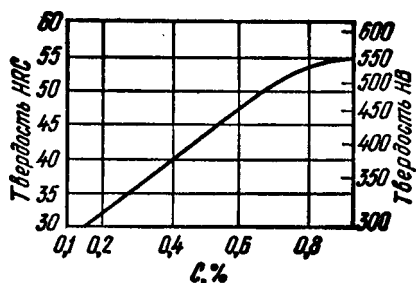
Рис. 238. Твердость полумартенситного слоя в зависимости от содержания углерода
