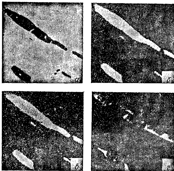
Рис. 24. Идентификация включений рентгеноспектральным методом: а — в отраженных электронах, X600; б - з — в характеристическом излучении серы (б), марганца (в) и свинца (з)
