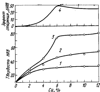
Рис. 399. Влияние содержания меди на твердость алюминиево-медного сплава в трех состояниях:
