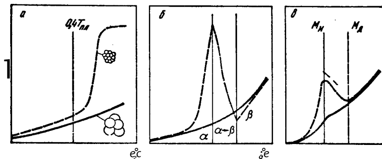
Рис. 50. Виды сверхпластичности; сплошные линии — ожидаемая пластичность; штриховые — сверхпластичность:
