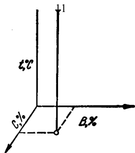
Рис. 112. Координаты для трехкомпонентной системы
