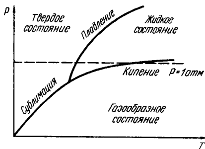
Рис. 5. Диаграмма состояния вещества в зависимости от давления и температуры
