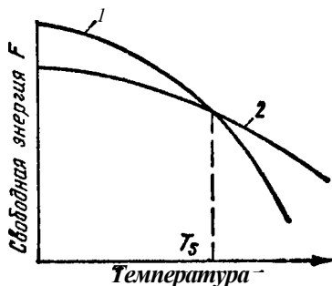
Рис. 26. Изменение свободной энергии жидкого (1) и кристаллического (2) состояния в зависимости от температуры
