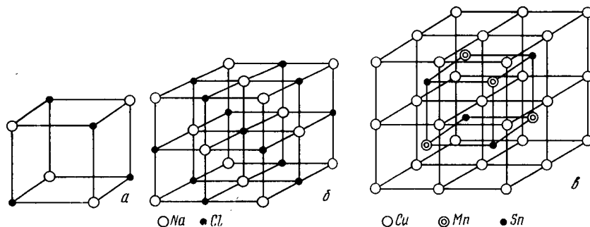
Рис. 79. Кристаллические решетки:
