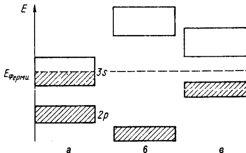
Рис. 3. Схема энергетической зонной структуры твердых тел (зоны, занятые электронами, заштрихованы): а — металл (Ba, а — полупроводник б — диэлектрик;
