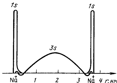
Рис. 1. Относительная вероятность пребывания электронов различных ионов в твердом теле уровней в металлическом натрии (схема дана только для самых внутренних 1s и внешних 3s электронов)
