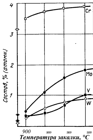
Рис. 312. Влияние температуры закалки на состав твердого раствора (сталь P6M5)
