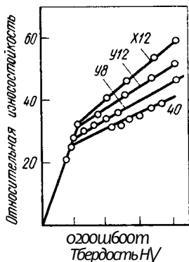
Рис. 355. Инос в зависимости от твердости материала
