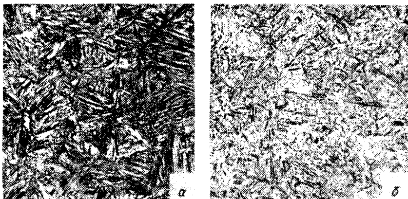
Рис. 203. Структура мартенсита в сталях массового назначения: а — крупноигльчатый; б — мелкоигльчатый, X 500
