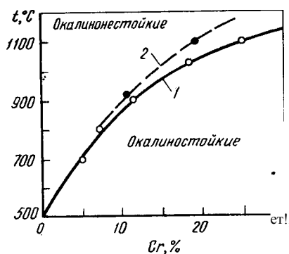
Рис. 326. Влияние хрома на окалиностойкость сталей:
