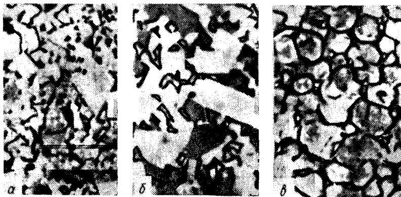
Рис. 322. Микроструктура твердых сплавов, X 100: а — ВКЗ; б — Т15К6; в — ГЭ0К4
