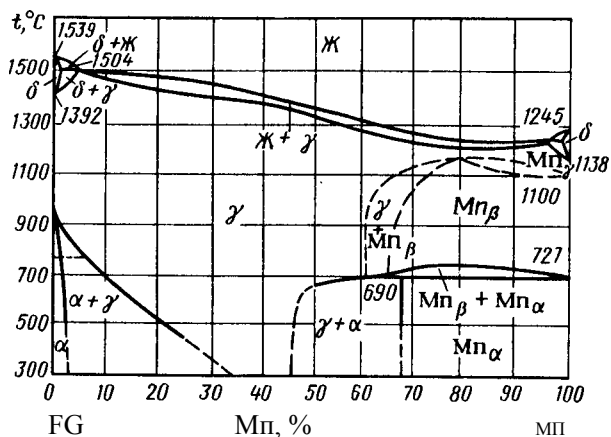
Рис. 274. Система Fe—Mn
