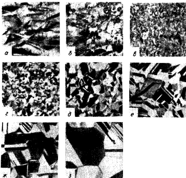
Рис. 71. Изменение микроstructures наклепанной латуни в зависимости от температуры нагрева, °C, X100:
