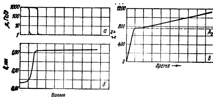
Рис. 251. Изменение магнитной проницаемости (ц) к глубины проникновения тока (в) при высокочастотном нагреве
