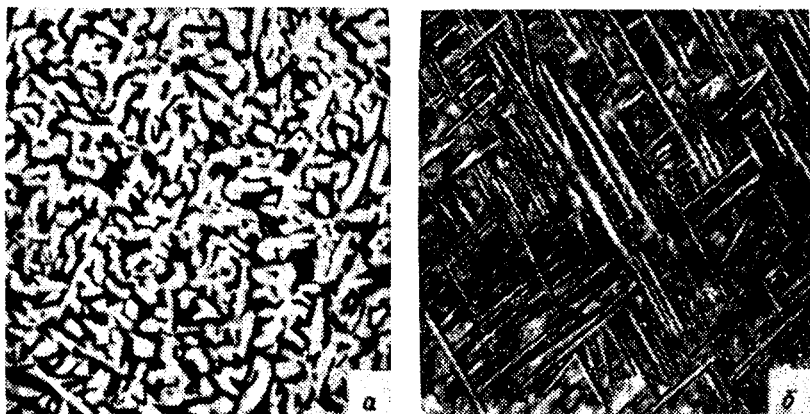
Рис. 427. Микроструктура алюминиевой бронзы с 10,5 % Al, X 100: а — после медленного охлаждения с 900 °С + эвтектид; б — после быстрого охлаждения (мартенсит)
