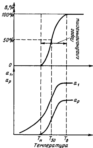
Рис. 54. Сериальные кривые
