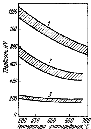
Рис. 289. Твердость (поверхностная) азотированного слоя в зависимости от температуры азотирования:
