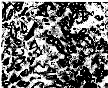
Рис. 423. Структура литой бронзы с 5 % Бп, X200
