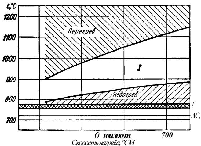
Рис. 250. Диаграмма выбора температуры нагрева для стали У10: / — скоростной электронагрев; // — медленный печной нагрев
