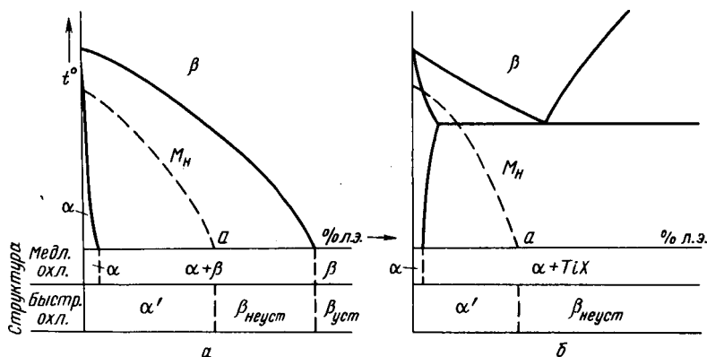
Рис. 363. Образование структур в титановых сплавах в зависимости от скорости охлаждения и содержания легирующего элемента
