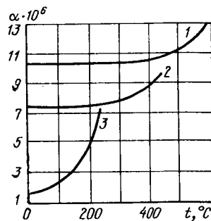
Рис. 380 Коэффициент линейного расширения сплавов Fe—Ni при различных температурах и содержании никеля %: /— 50; 2—42; 3—3
