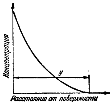
Рис. 264. Изменение концентрации диффундирующего элемента по глубине
