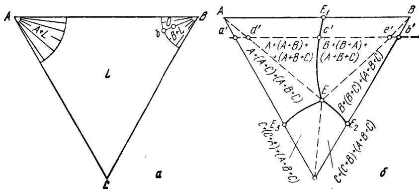
Рис. 125. Изотермическое сечение тройной системы, показанной на рис. 122:
