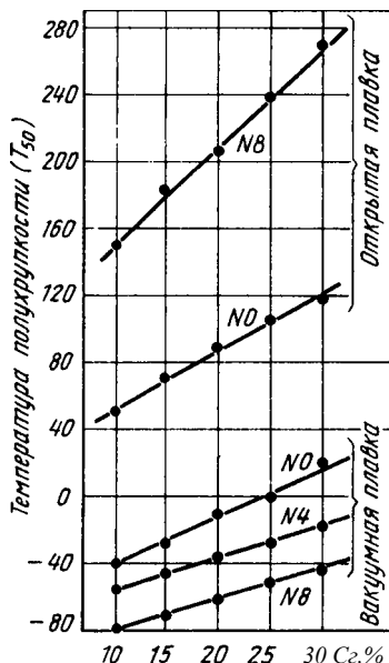
Рис. 344. Влияние углерода и азота (суммы) на положение порога хладноломкости (определено по значению ударной вязкости 1000 кДж/м²)
