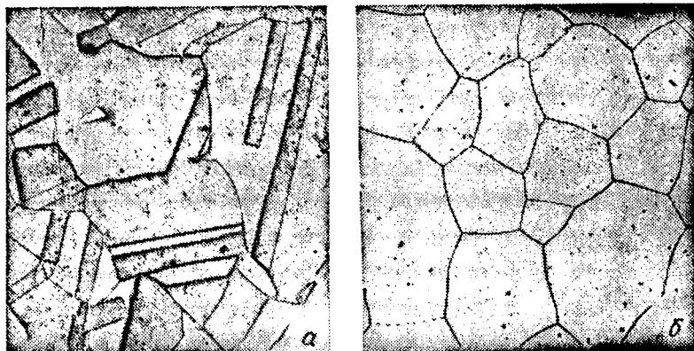
Рис. 139. Микроструктура железа. X400i а —* аустенит; б — феррит
