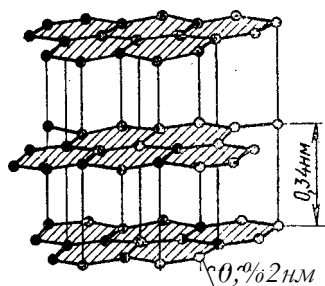
Рис. 160. Кристаллическая структура графита
