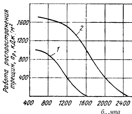
Рис. 287. Зависимость работы распространения трещины (при нормальной температуре) от прочности стали:
