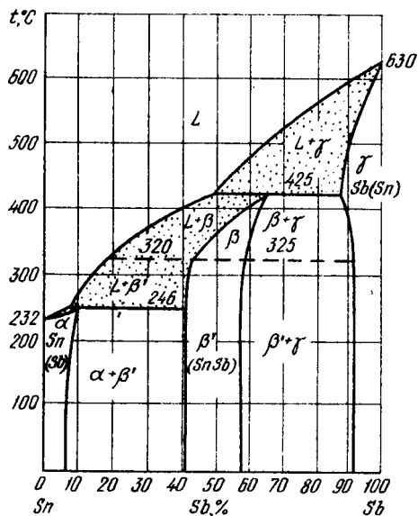
Рис. 432. Диаграмма состояния Бп — СБ
