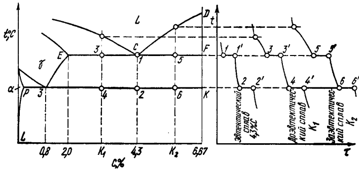
Рис. 145. Диаграмма состояния Fe—C. Вторичные превращения ■ высокоуглеродистых сплавах (чугунах)
