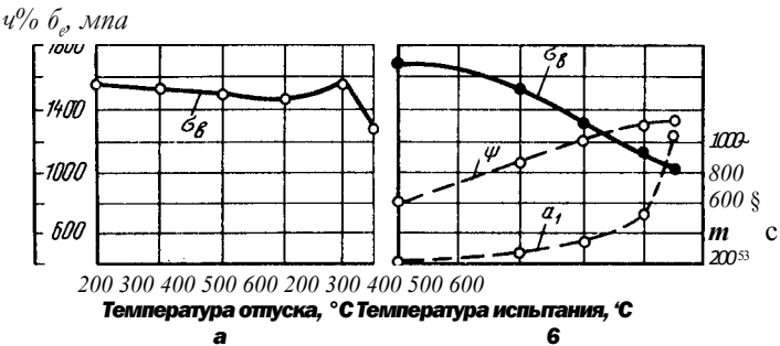
Рис. 321. Влияние отпуска (в) и температуры испытания (б) на свойства стали 3Х2В8
