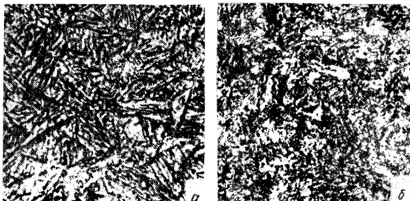
Рис. 220. Микроструктура стали (0,46% С). X 500: а — отпуск при 400 °С, троостит; б — отпуск при 550 °С, сорбит
