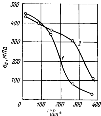
Рис. 409. Свойства сплавов АК2 (1) АК4 (2) при повышенных температурах
