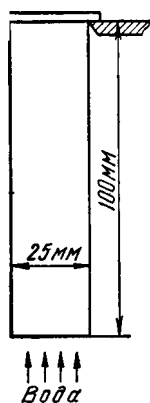
Рис. 236. Схема заковки образца при испытании на прокаливаемость методом торцевой заковки
