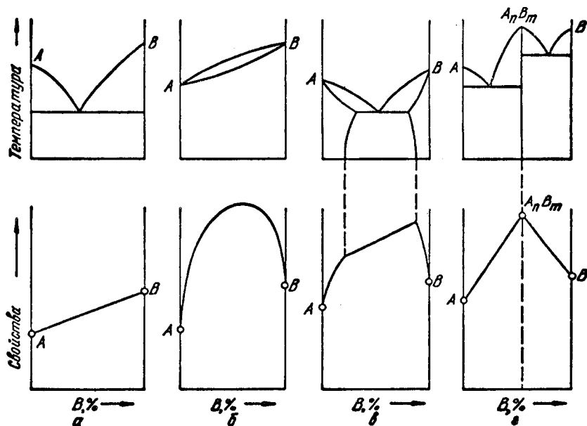
Рис. 127. Свойства сплавов и их диаграммы еостояния
