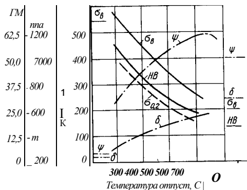
Рис. 226. Механические свойства стали 40 в зависимости от температуры отпуска
