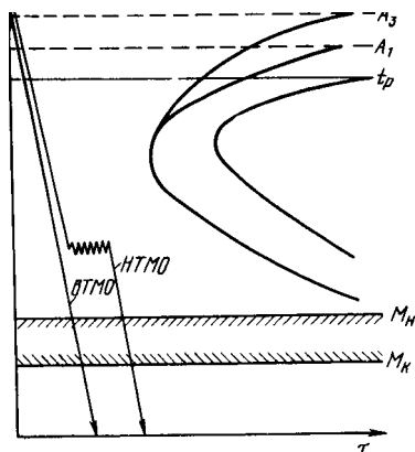
Рис. 226. Классификационная схема ТМО
