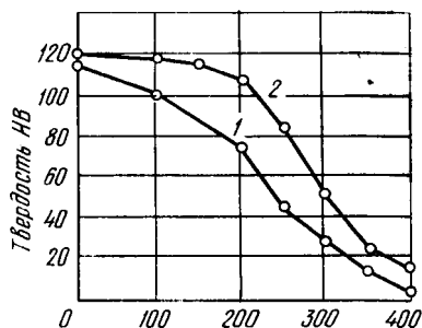
Рис. 409. Свойства сплавов АК2 (1) АК4 (2) при повышенных температурах
