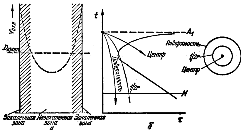
Рис. 233. Схемы, показывающие различную скорость охлаждения по сечению ■ в связ* с этим несквозную прокаливаемость
