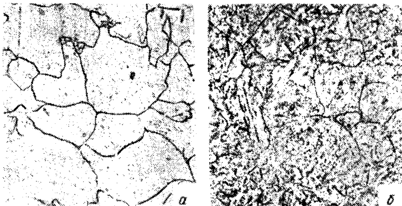
Рис. 282. Структура феррита в сплаве с 4.2 % Сг:
