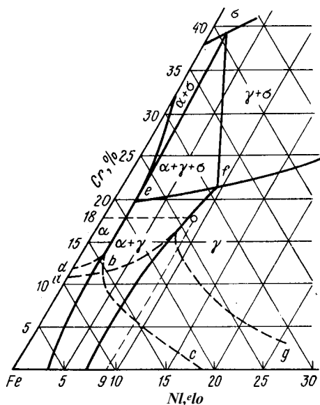
Рис. 346. Железный угол системы Fe—Cr—Ni. Туры. С понижением температуры область \gamma + \alpha уходит вправо и ее крайнее положение при 20^{\circ}\text{C} показано пунктирными линиями, закончившимися в точках c и g , а при повышении температуры область уходит влево и ее крайнее положение при 1100^{\circ}\text{C} показывает пунктирные линии, заканчивающиеся в точках a , d .
