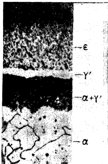
Рис. 265. Микроструктур* азотированного слоя железа (при 650^\circ\text{C} с медленным охлаждением), \times 500
