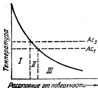
Рис. 249. Распределение температур по глубине при поверхностной закалке
