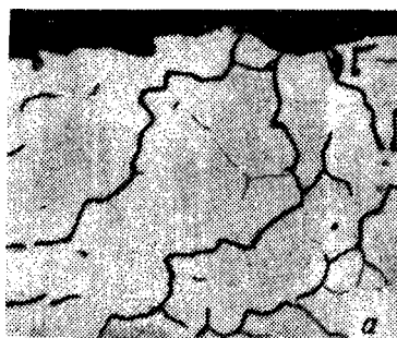
Рис. 350. Микроструктура нержавеющей стали, пораженной интеркристаллитной коррозией: а — X 200; б — X 500
