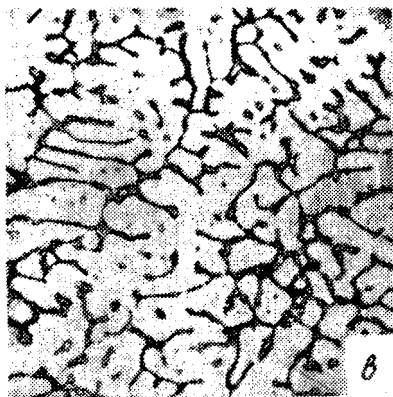
Рис. 407. Микроструктура литейных сплавов алюминия, X200:
