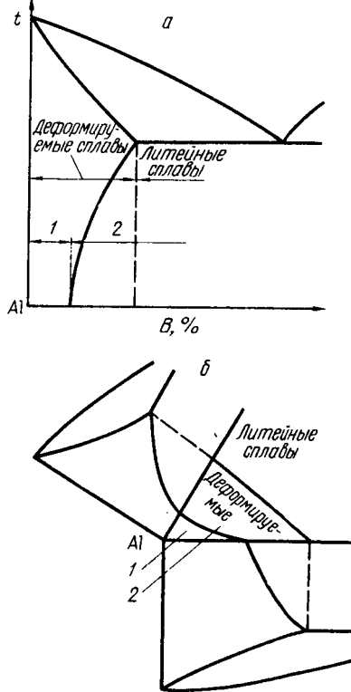
Рис. 403. Классификация алюминиевых сплавов по диаграмме состояния: а — двойная система; б — тройная система; 1 — сплавы, не упрочняемые термической обработкой; 2 — сплавы, упрочняемые термической обработкой
