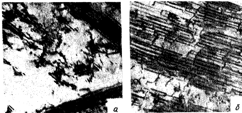
Рис. 16. Дефекты упаковки в марганцевой стали: а — единичные; б — скопления. ХЗО 000
