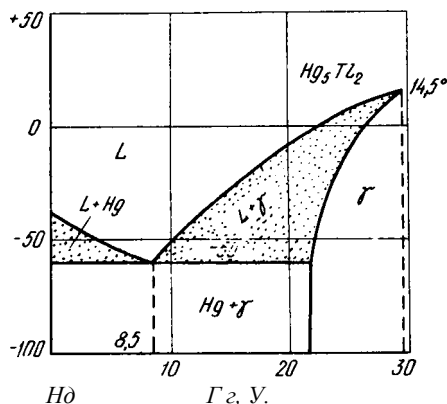
Рас. 439. Дмграмм* состояния Нс—А1
