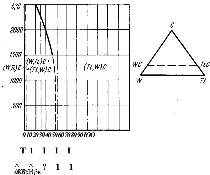
Рис. 323. Псевдобинарный разрез системы —Ti—C
