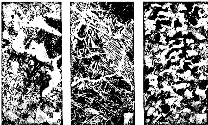
Рис. 247. Структура стали Б0, X100:
