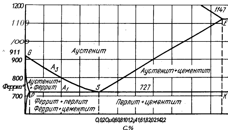
Рис. 172. «Стальной» участок диаграммы Fe—C
