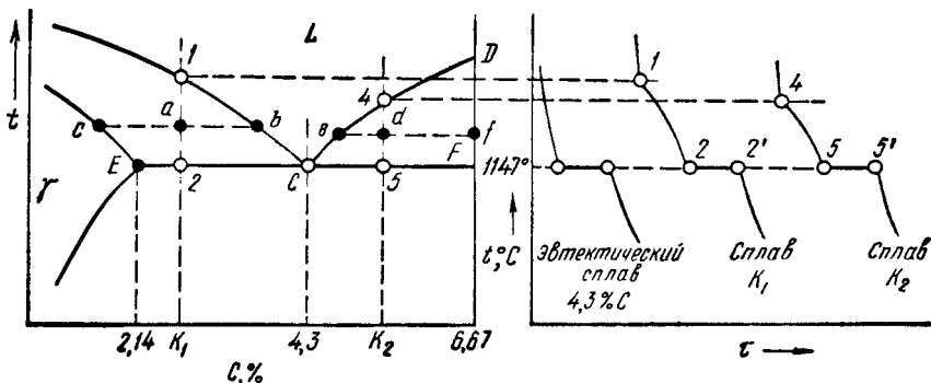
Рис. 137. Часть диаграммы состояния Fe—C. Первичная кристаллизация высокоуглеродистых сплавов
