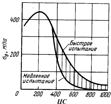
Рис. 328. Предел прочности железа в зависимости от температуры испытаний (заштрихована область напряжений, вызывающих ползучесть)
