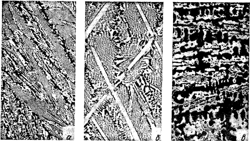
Рис. 146. Микроструктура чугуна:
