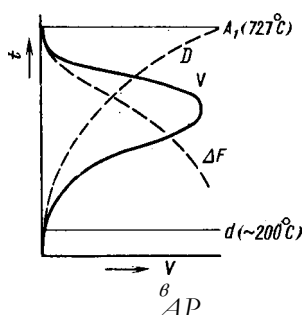
Рис. 182. Скорость распада аустенита (сплошная линия) в зависимости от степени переохлаждения (температуры)
