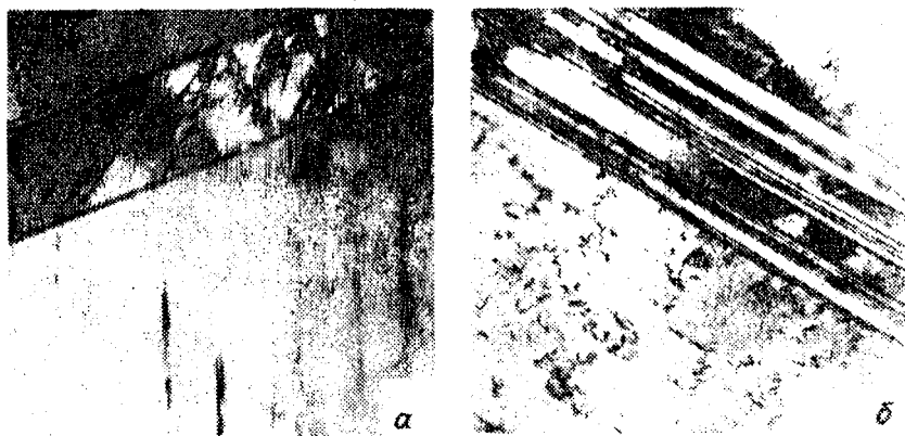
Рис. 18. Двойники отжига (а) и деформационные, X 16 000 (б)
