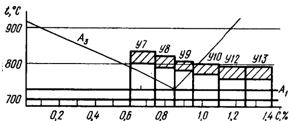
Рис. 306. Температура закаливания углеродистых инструментальных сталей
