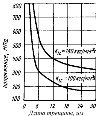
Рас. 57. Кривые разрушающего напряжения в зависимости от длины трещины
