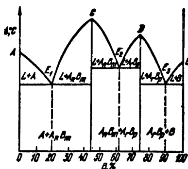
Рис. 102. Диаграмма состояния с двумя устойчивыми химическими соединениями
