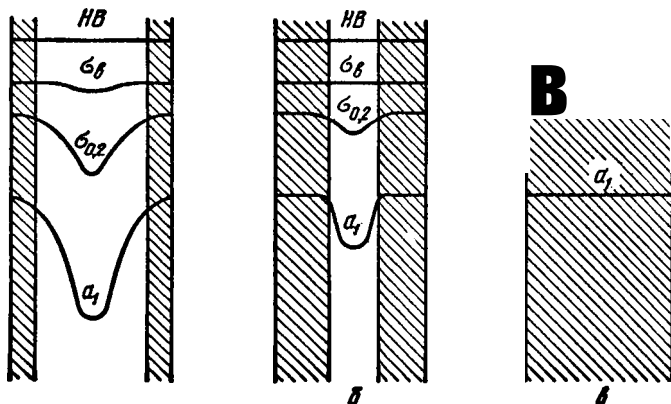
Рис. 241. Влияние глубины заделки на механические свойства закаленной и отпущенной сталей с различной прокаливаемостью
