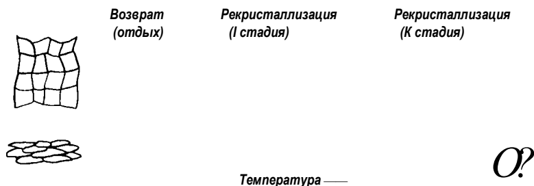
Рис. 69. Схема изменения строения нагнатованного металла при нагреве
