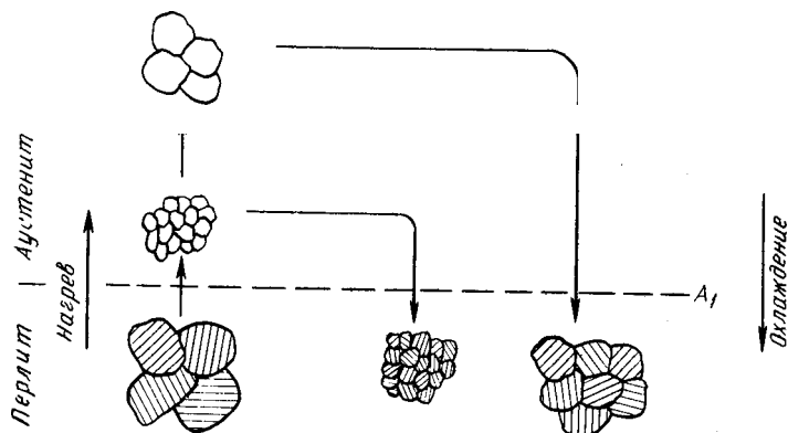
Рис. 176. Схема изморозения рванера крип перлита в зависимости от нагрева и аустенитноА области
