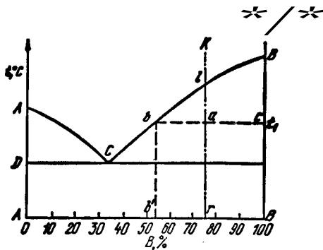
Рис. 95. Диаграмма состояния (к применению на ней правила отрезков)
