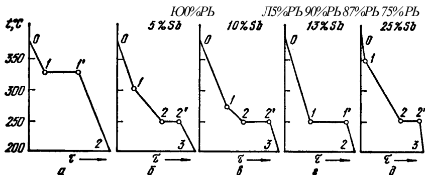
Рис. 90. Кривые охлаждения сплава РЬ—БЬ
