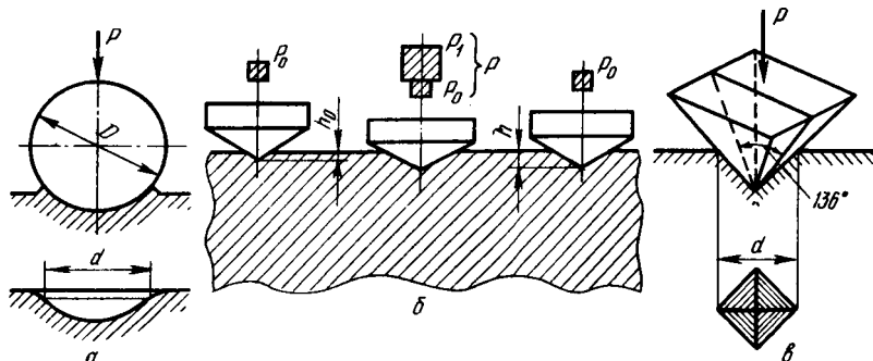
Рис. 59. Схемы испытания на твердость:
