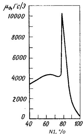
Рис. 385. Начальная магнитная проницаемость сплавов Ре-Ы1
