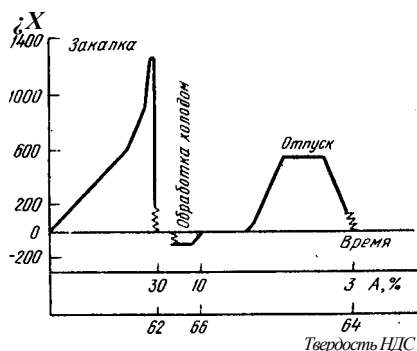
Рис. 314. Режим термической обработки инструментов из быстрорежущей стали с обработкой холодом
