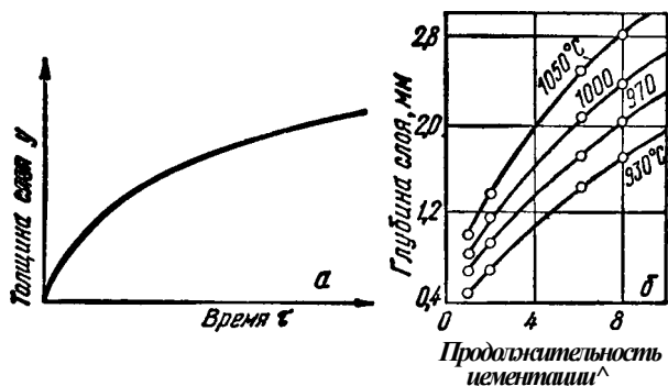
Рис. 268. Влияние на глубину слоя продолжительности диффузионного насыщения (а) и продолжительности цементации при различных температурах (б)
