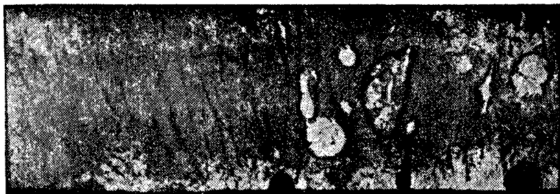
Рис. 304. Флокены в стали (нзлом)
