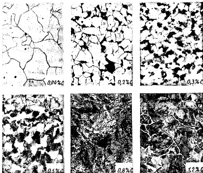
Рис. 143. Структура сталей с различным содержанием углерода, Ж 200
