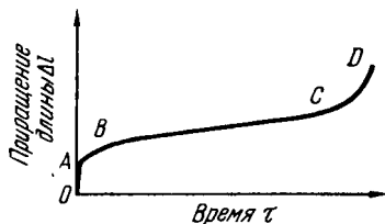
Рис. 329. Кривая ползучести
