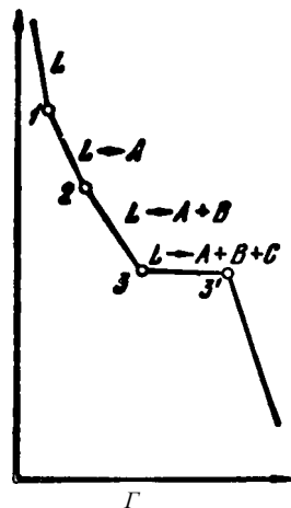
Рис. 119. Кривая охлаждения тройного сплава с образованием двойной и тройной эвтектик, состоящих из числа компонентов A , B , C
