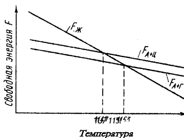
Рис. 161. Изменение свободной энергии жидкого сплава (ж) * смеси аустенит + цементит (а + ц) и аустенит + графит (а + р) с изменением температуры (схема)
