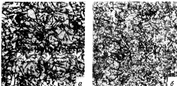
Рис. 316. Структура (X500) отпущенной быстрорежущей стали P6M4 при температуре отпуска, °С: а — 600; б — 600
