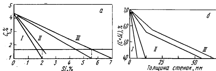
Рис. 168. Структурная диаграмма для чугуна, показывающая, какая должна получиться структура в отливке в зависимости от: а — содержания кремния и углерода (толщина стенки 50 мм); б — суммы содержания углерода и кремния и от толщины стенки; I — белые чугуны; II — перлитные чугуны; III — серые ферритные чугуны
