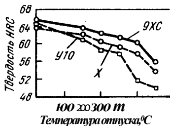
Рис. 307. Влияние температуры отпуска на твердость сталей
