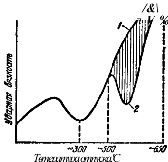
Рис. 290. Влияние отпуска на ударную вязкость легированной стали:
