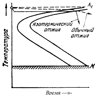
Рис. 248. Кривые изотермического обычного отжига
