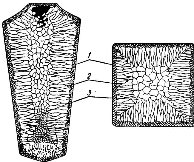
Рже. 34. Схема строения стального слитка
