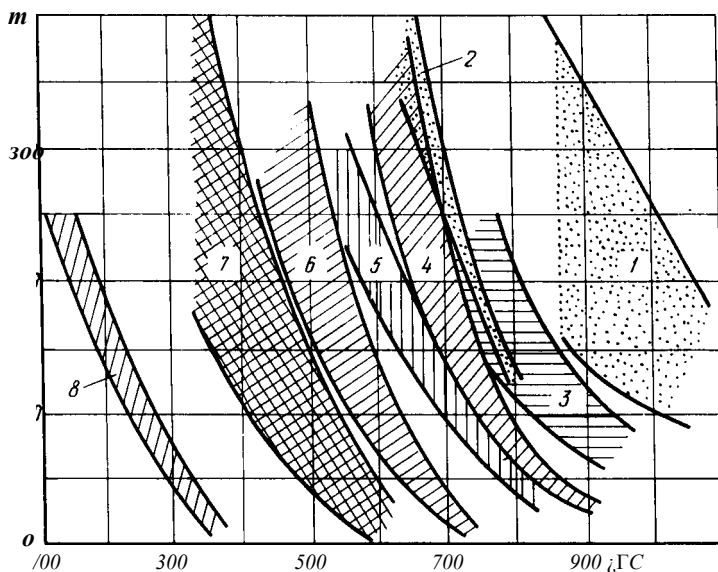
Рис. 330. Зависимость длительной прочности (1000 ч) от температуры сплавов: 1 — молибдена; 2 — никеля; 3 — кобальта; 4 — сплава типа ХНЗб; 5 — аустенитные стали; 6 — теплоустойчивые стали; 7 — титана; 8 — алюминия
