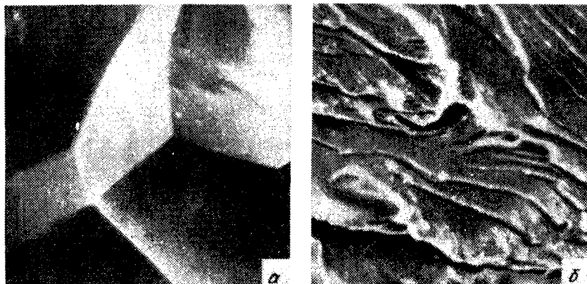
Рис. 373. Стереоскопическая фрактография излома молибдена: а — межкристаллический излом, ХЗО; б — транскристаллитный излом, ХИО
