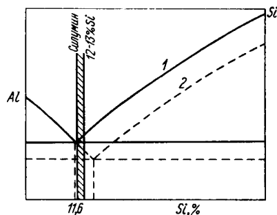
Рис. 408. Влияние модифицирования на кристаллизацию в системе Al— У —* без модифицирования; 2 — после модифицирования
