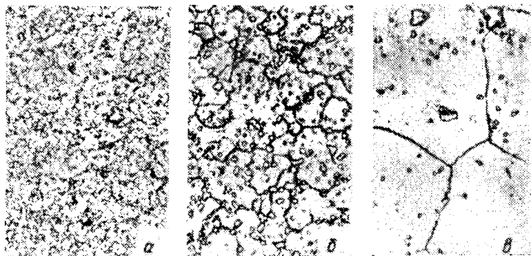
Рис. 315. Структура (Х500) закаленной быстрорежущей стали Р6М5 при тем* пературе закалки, °С:
