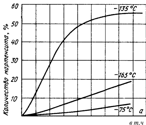
Рис. 212. Изотермическое превращение аустенита в мартенсит (сплав \text{Re}-23\% \text{Ni}-3\% \text{Mn} ) при разных температурах (а) и диаграмма изотермического превращения (б) (цифры у кривых — степень превращения)
