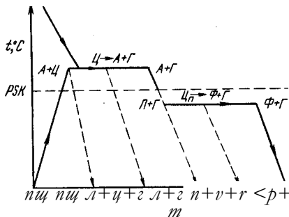
Рис. 163. Схема образования структур при графитизации чугуна
