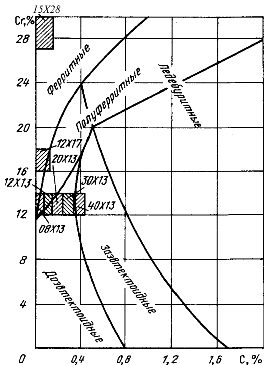
Рис. 341. Система Fe—C—Cr и положение в ней промышленных хромистых нержавеющей сталей
