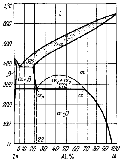
Рис. 437. Диаграмма состояния Zn—Al
