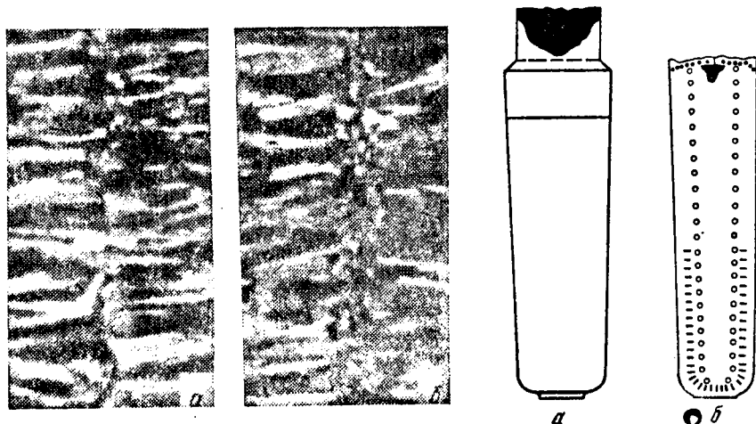
Рис. 36. Транскристаллизация слитка алюминиевой бронзы
