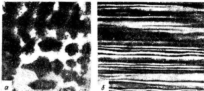
Рис. 303. Дефекты махро* и микроструктуры легированной стали, X 130 (Совер): а — дендритная ликвация; б — полосчатость
