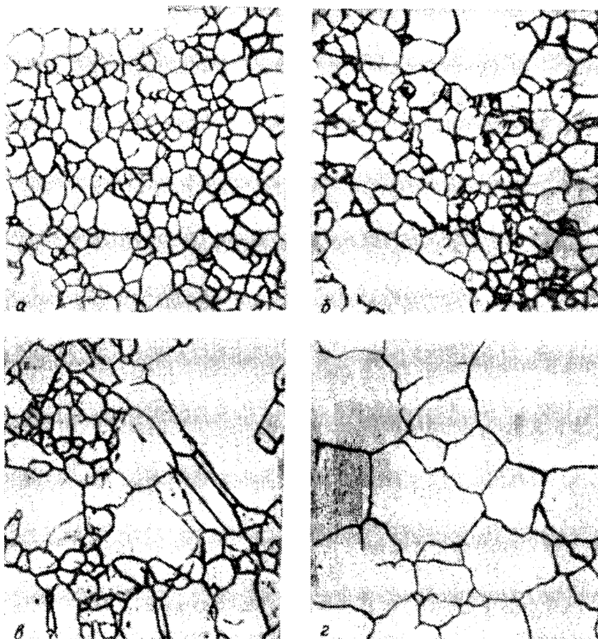
Рис. 72. Процесс роста зерна при рекристаллизации (X 100)
