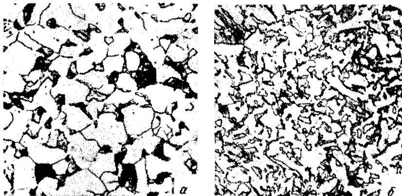
Рис. 262. Микроструктура сердцевины цементированной углеродистой стали, феррит+перлит. X250:
