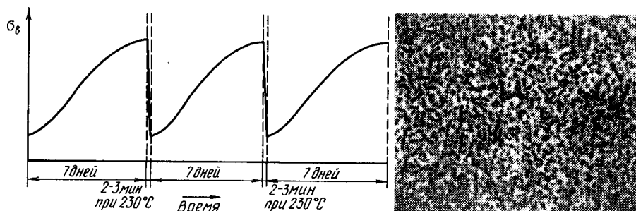
Рис. 397. Кривые старения после возврата к свежезакаленному состоянию (кратковременный нагрев при 230 °С.)
