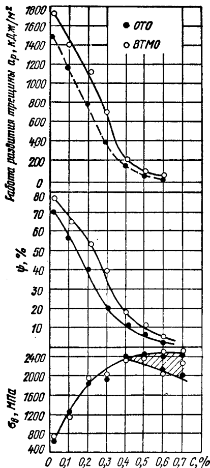
Рис. 296. Влияние углерода на прочность ( \sigma_B ), пластичность ( \phi ) и работу распространения трещины. Сталь типа X5M2CФ
