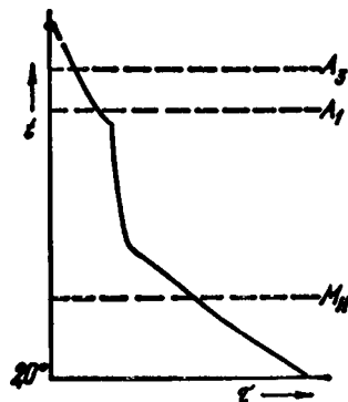
Рис. 232. Идеальная кривая охлаждения при закалке
