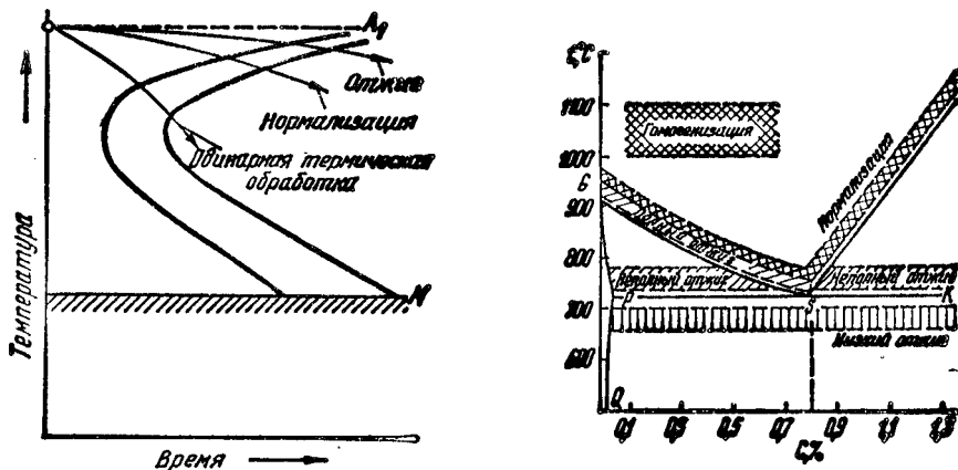
Рис. 246. Кривые охлаждения для отжига, нормализации и однородной термической обработки* Сетки» наложенные на диаграмму изотермического распада аустенита
