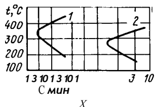
Рис. 393. Диаграмма изотермического распада переохлажденного твердого раствора в алюминиевых сплавах (указано начало распада):
