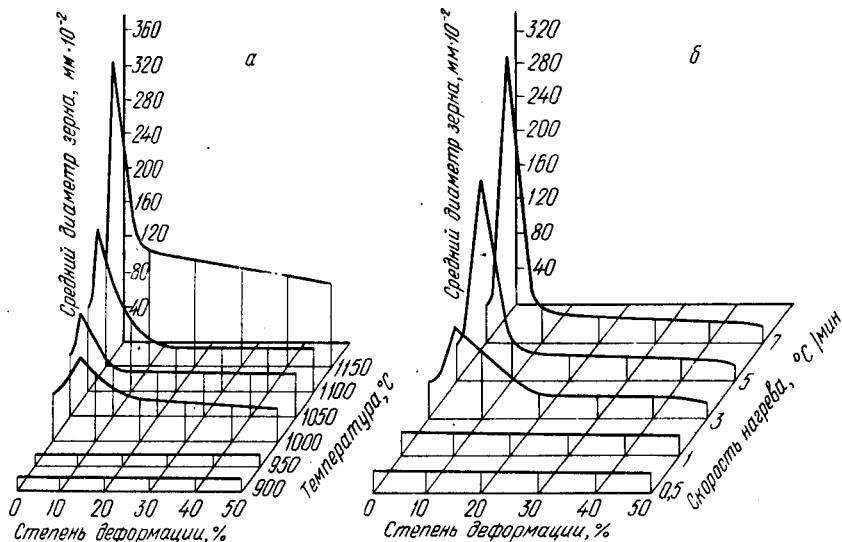
Рис. 77. Диаграмма рекристаллизации жаропрочного никелевого сплава а — скорость нагрева 7 °С/мин; б — температура нагрева 1080 °С
