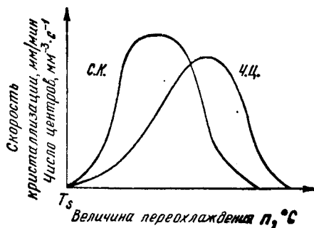
Рис. 30. Скорость роста кристаллов (с. к.) и скорость зарождения центров кристаллизации (ч. ц.) в зависимости от степени переохлаждения
