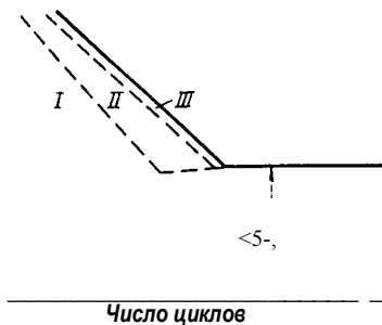
Рис. 61. Кривая усталости
