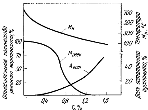
Рис. 206. Влияние содержания углерода на относительное количество речного мартенсита, температуру M_s и количество остаточного аустенита
