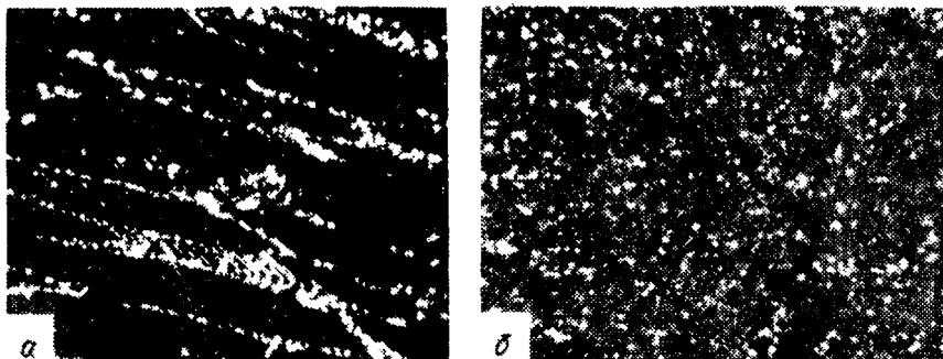
Рис. 320. Микроструктура сталей, X 100: а — X12; б — X6ВФ
