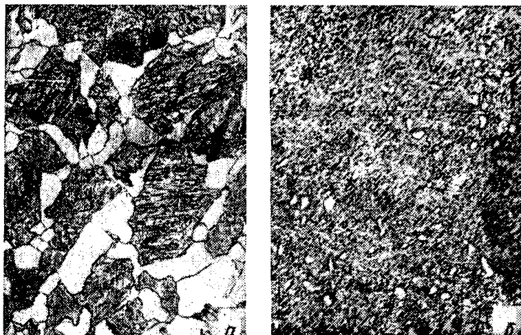
Рис. 229. Микроструктура аакаленной стали:
