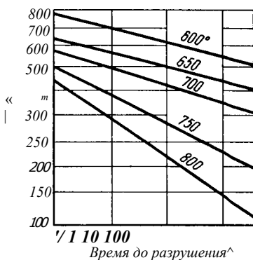
Рис. 338. Жаропрочные свойства сплава нимоник (типа ХН77ТЮР)
