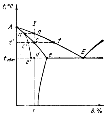
Рис. 107. Изменение среднего состава кристаллов при неравновесной кристаллизации
