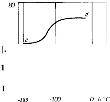
Рис. 214. Изотермическая (Бс) и атермическая (об и с. I) кинетики мартенситного превращения в сплаве Fe—24 % N1—5 % Mo
