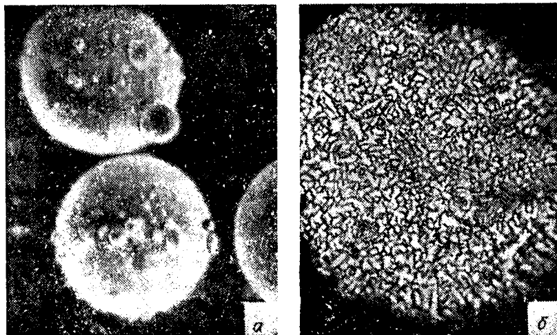
Рис. 109. Гранулы ( а ) и их структура ( б ) быстрорежущей стали, полученной закалкой из жидкого состояния
