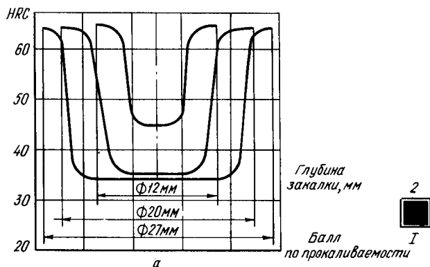
Рис. 305. Прокаливаемость углеродистой стали У12:
