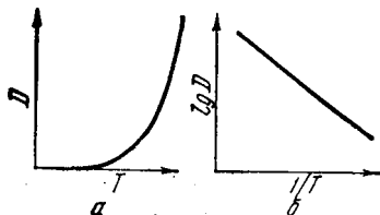
Рис. 287. Зависимость коэффициента диффузии от температуры
