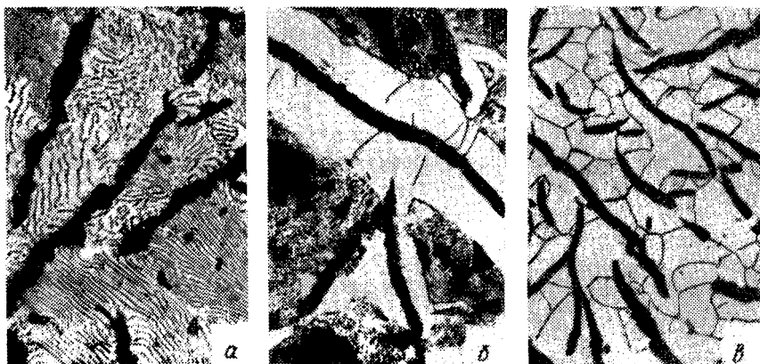
Рис. 164. Микроструктура серого чугуна:
