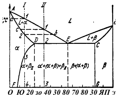
Рис. 97. Диаграмм, стояния с,вт.ктикой 33 Пределами рзСТВОРИМОСТИ и яв- ляются двухфазными, состоящими из \alpha\alpha + \beta . Окончание кристаллизации происходит по эвтектиче- ской реакции
