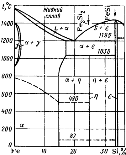
Рис. 278. Система Fe—Si
