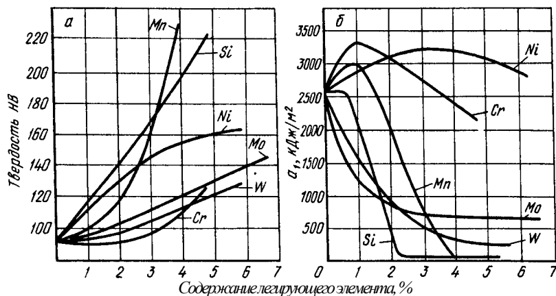
Рис. 280. Влияние легирующих элементов на свойства феррита: a — твердость; б — ударная вязкость
