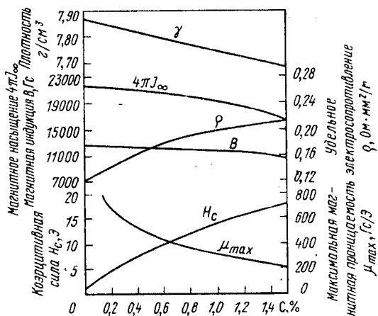
Рис. 149. Влияние углерода на некоторые физические свойства стали
