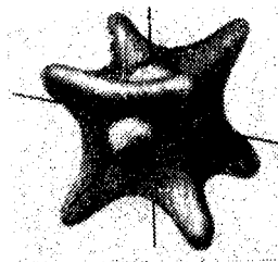
Рис. 21. Модель, показывающая изменение предела прочности кристалла меди в зависимости от направления приложения нагрузки
