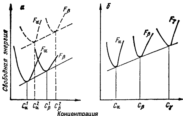
Рис. 88. Изменение свободной энергии P твердых растворов в зависимости от их концентрации:
