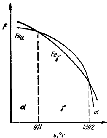
Рис. 130. Изменение свободных энергий \alpha - и \gamma -модификаций железа при изменении температуры
