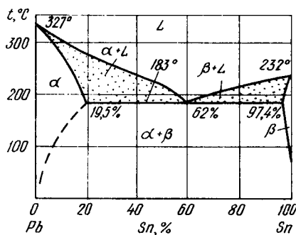
Рис. 434. Диаграмма состояния РЬ—Бп
