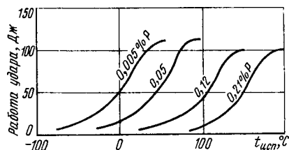
Рис. 151. Влияние фосфора* на хладноломкость стали (0,2 К С. 1,0 % Мп)
