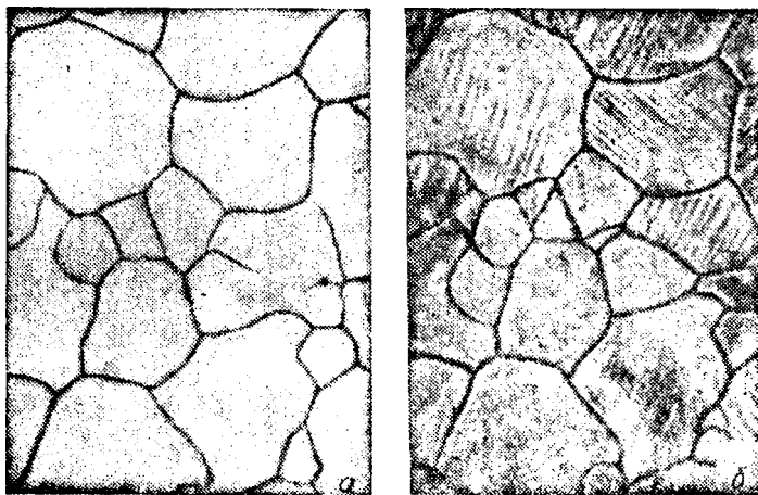
Рис. 42. Изменение структуры железа при пластическом деформировании (Розенгейн), X 100:
