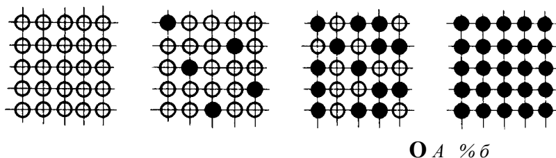
Рис. 84. Кристаллические решетки твердых растворов замещения при неограниченной растворимости компонентов
