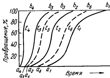
Рис. 185. Кинетические кривые превращения аустенита в перлит при различных температурах U, > U > I, > \dots
