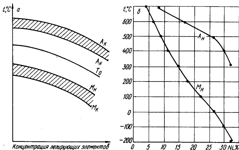
Рис. 209. Температуры прямого ( A_{1\Gamma} — A_{1K} ) и обратного ( M_{\Gamma} — A_{\Gamma} ) превращений: а — схема; б — температуры M_{\text{н}} и A_{\text{н}} в системе Fe—Ni
