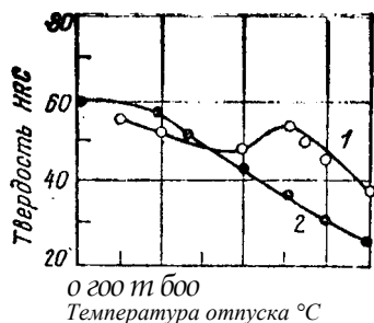
Рис. 294. Влияние температуры отпуска на твердость сталей: 1 — 30ХМ2СФ; 2 — 40ХНМ
