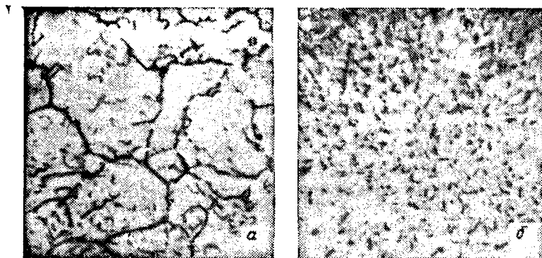
Рис. 291. Микроструктура хромоникелевой стали после отпуска при 550 °С, X 500:
