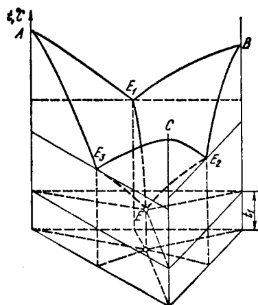
Рис. 121. Диаграмма состояния трехкомпонентной системы. Компоненты нерастворимы в твердом состоянии и образуют тройную эвтектику (пространственное изображение)
