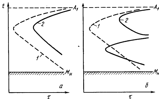
Рис. 283. Диаграммы изотермического распада аустенита: а — углеродистая (1) и легированная некарбидообразующими элементами (2) стали; б — углеродистая (1) и легированная карбидообразующими элементами (2) стали
