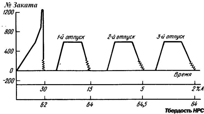
Рис. 313. Обычный режим термической обработки
