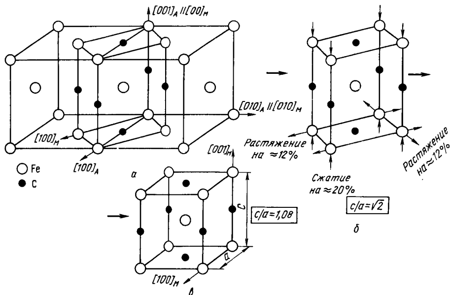
Рис. 208. Схема Бейна:
