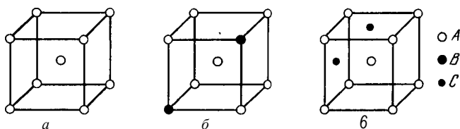
Рис. 81. Кристаллическая решетка о. ц. к.:
