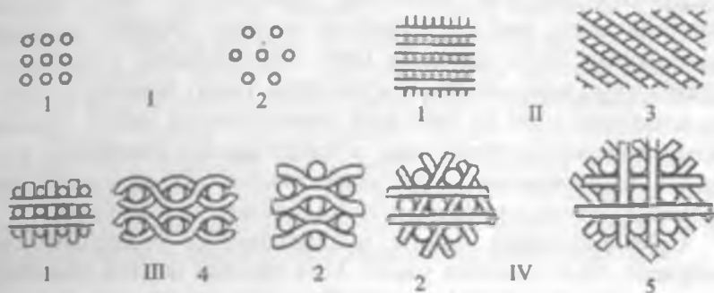
2.2-rasm. Kompozitsion materiallarni mustahkamlovchilar bilan armirlash turlari: I – bir tamonlama yo'naltirilgan taxlash, II – ikki tamonlama yo'nalishda taxlash, III – uch tamonlama yo'nalishda taxlash; 1 – to'g'ri burchakli, 2 – olti burchakli, 3 – og'ma burchakli, 4 – to'kilgan, 5 – ko'p to'kilgan
