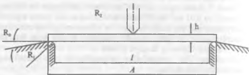
1-rasm. Namunaning statik egilishda mustahkamlikka sinashdagi holat.
