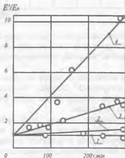
3.1-rasm. SKB kauchuginig yorug'lik nuri ta'sirida ularning cho'zilishga bo'lgan mustahkamligining pasayish diagrammasi: 1 – 25 °C da yorug'liksiz; 2 – 80 °C da yorug'liksiz; 3 – 25 °C yorug'likda va 4 – 80 °C yorug'likda
