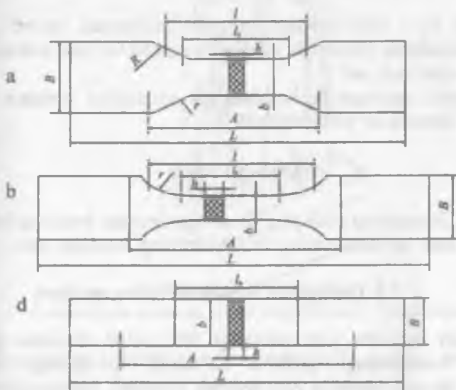
2-rasm. Namunaning cho'zilishda buzuvchi kuchlanishni aniqlashdagi shakllari va o'lchamlari:
