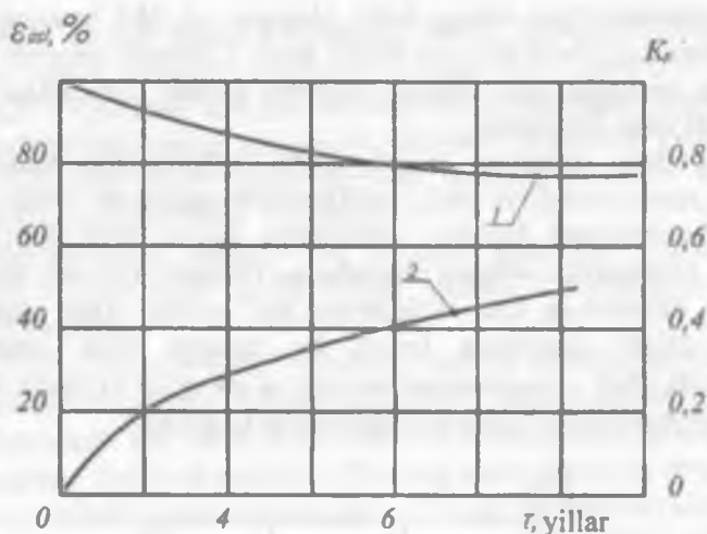
3.2-rasm. Rezina materialining cho'zilgan va erkin holatlarda ularda eskirishning jadallashuvini ko'rsatuvchi diagramma. 1 – eskirish jadalligini o'zgarishi; 2 – qoldiq deformatsiya paydo bo'lishligi
