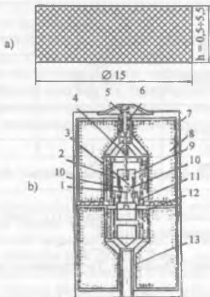
10-rasm. Namuna (a) va issiqlik o'tkazuvchanlik koeffitsiyentini aniqlash uchun (b) IT-L-400 uskunasiining prinsipial sxemasi: 1 – teplomer; 2 – termojuft; 3 – adiabat; 4 – qisqich; 5 – prujina; 6 – kirish patrubbasi; 7 – korpus; 8 – issiqlik himoya; 9 – sterjen; 10 – sinalayotgan namuna; 11 – asos; 12 – istuvchi blok; 13 – chiqish patrubbasi Issiqlik o'tkazuvchanlikni o'lchashda, unga tegishli t_s harorat quyidagicha aniqlanadi.
