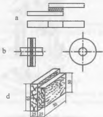
4-rasm. Yelimlarni sinash uchun namunalar: a) elimlarning siljishda mustahkamligini sinash; b) elimlarning uzilishda mustahkamligini sinash; d) elimlangan yog'ochlarni siljishda sinash.
