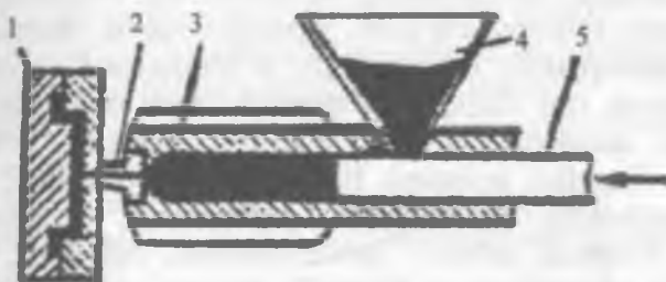
1.8-rasm. Quyish yo'li bilan buyumlarni bosim ostida hosil qilish sxemasi:
