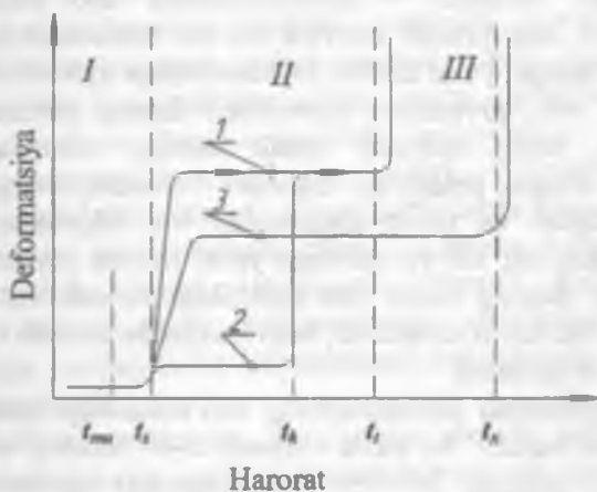
1.3-rasm. Polimerlarning termomexanik egri chizig'i: 1 – nokristal chiziqli; 2 – kristalli; 3 – siyrak to'rsimon polimerlar; t_\mu , t_b , t_h , t_x – shishalanish, kristallanish, oquvchan va kimyoviy parchalanish harorat nuqtalari; I – III – shishasimon, yuqori elastiklik va qovushqoq oquvchan holat joylari
