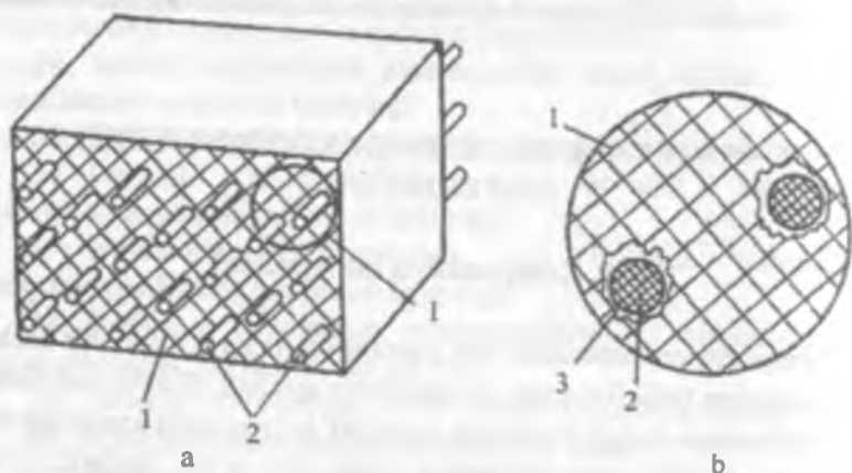
2.1-rasm. Kompozitsion material kesimi: a – kvadrat kesimi; b – aylana kesimli; 1 – matritsa; 2 – mustahkamlovchi; 3 – chegara qoplami
