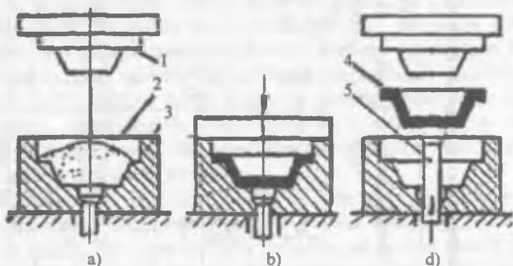
1.7-rasm. To'g'ri presslash sxemasi:
