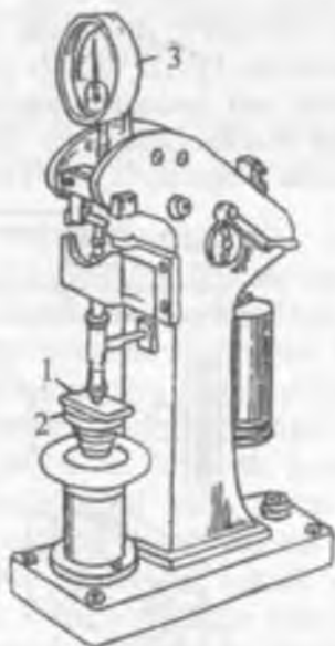
3-rasm. Brinell uskunasi: 1—sinaladigan namuna; 2—ko'targich stoli; 3—indikator.
