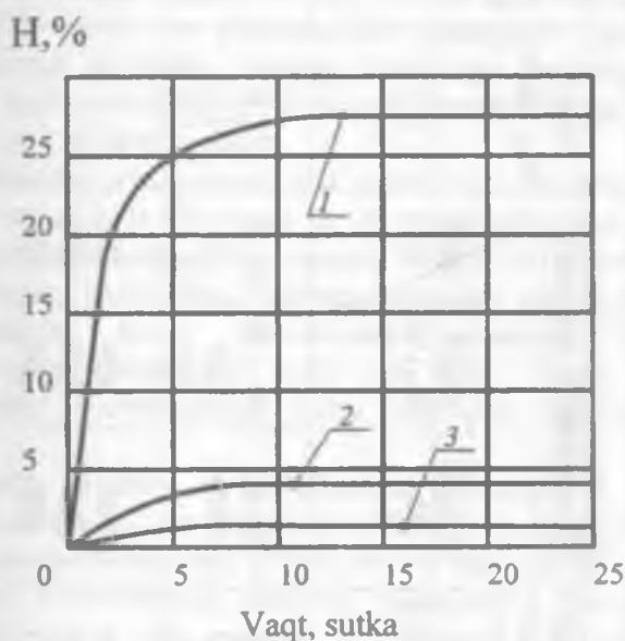
1.6-rasm. Qatlamli plastik massalarning suv shimish darajasi (N): 1 – yog'ochqatlamli; 2 – tekstalit; 3 – shishaqatlamli
