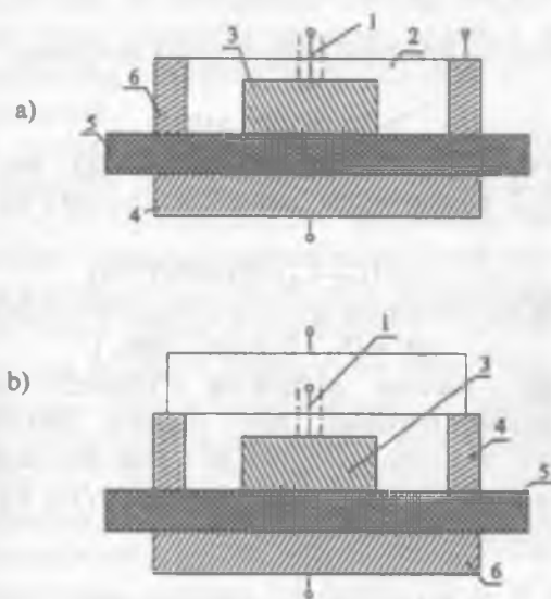
7-rasm. Solishtirma yuza (a) va solishtirma hajm (b) elektr qarshiliklarini aniqlashda elektrodلarni yoqish sxemasi:
