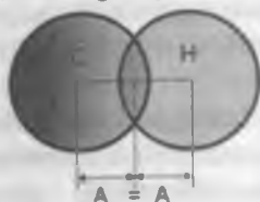
1.2-rasm. Elementlari qutubsiz (a) va qutubli (b) bog'lanish sxemasi
