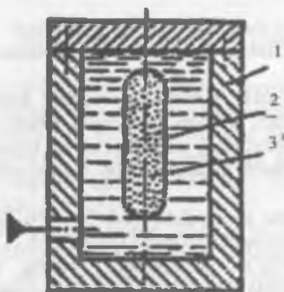
6.5-rasm. Hidrostatik presslash sxemasi: 1–kamera-mahsus germetik; 2–elastik qobiq; 3–kukun
