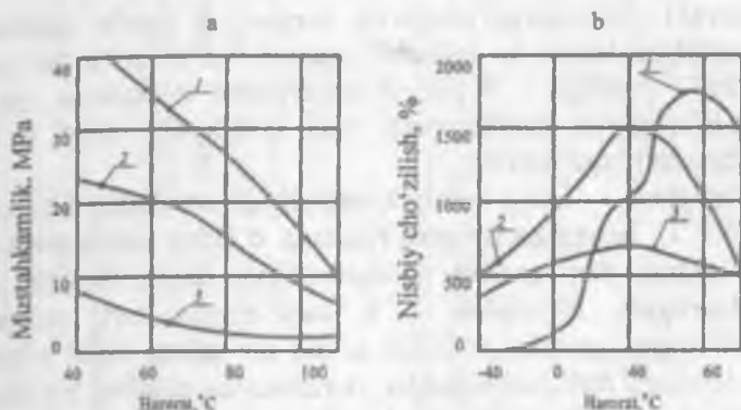
1.4-rasm. Polietilen va SEP cho'zilishdagi mustahkamligining hamda nisbiy cho'zilish darajasining haroratiga bog'likligini ko'rsatuvchi diagramma: a – mustahkamligi; b – nisbiy cho'zilishi; 1 – PEND; 2 – SEP; 3 – PEVD
