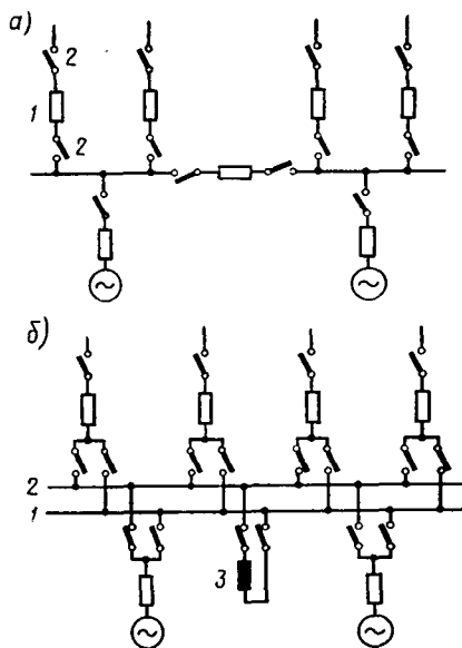
Рис. 8.12. Схема с одной системой сборных шин (а):
