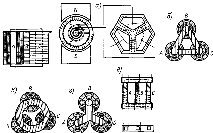
Рис. 6.25. Трансформаторы М. О. Доливо-Добровольского: а — с радиальным расположением сердечников; б — в — «призматические»; г — с параллельным расположением стержней в одной плоскости
