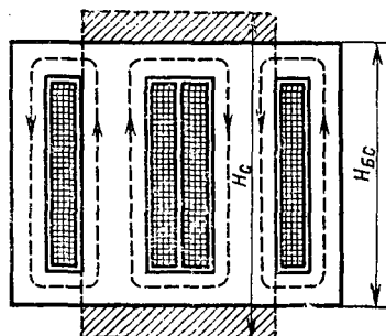
Рис. 9.10. Бронестержневой однофазный трансформатор:
