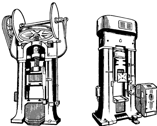
Рис. 9.26. Отечественный винтовой пресс до и после модернизации
