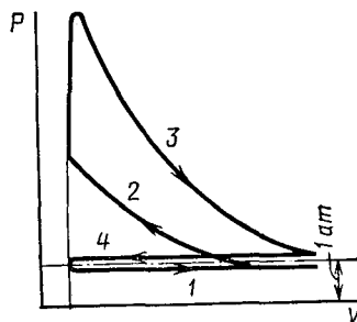
Рис. 4.19. Индикаторная диаграмма работы четырехтактного двигателя:
