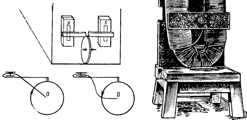
Рис. 5.10. Схема униполярного генератора (по рисунку Фарадея): справа — большой электромагнит Королевского института, который использовал Фарадей
