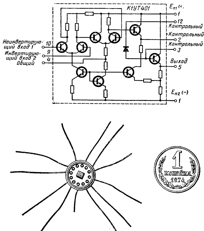
Рис. 10.13. Серийный линейный операционный усилитель К19Т401, выполненный в виде интегральной микросхемы (без верхней части корпуса); сверху схема усилителя, содержащая 9 транзисторов, 1 диод и 12 резисторов
