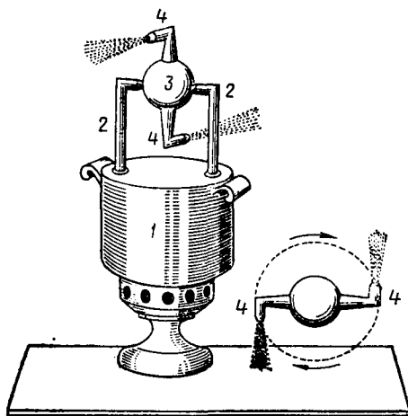
Рис. 4.21. Эолипил Герона:
