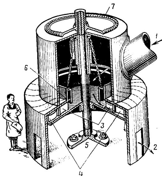
Рис. 3.8. Гидравлическая турбина Сафонова: 1 — подвод воды; 2 — отвод воды; 3 — лопасти направляющего аппарата; 4 — рабочие лопасти; 5 — подпятник вала; 6 — кольцевая заслонка, регулирующая количество поступающей воды; 7 — коническая шестерня для передачи энергии машине-орудию
