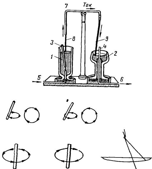
Рис. 5.11. Схема установки Фарадея для демонстрации электромагнитного вращения (по рисунку Фарадея):
