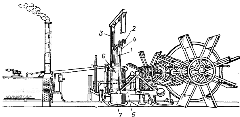
Рис. 4.16. Паровой двигатель парохода Фультона «Клермонт»: 1 — шток; 2 — крейцкопф; 3 — направляющая; 4 — шатун; 5 — баланси́р; 6 — пор- шень; 7 — цилиндр
