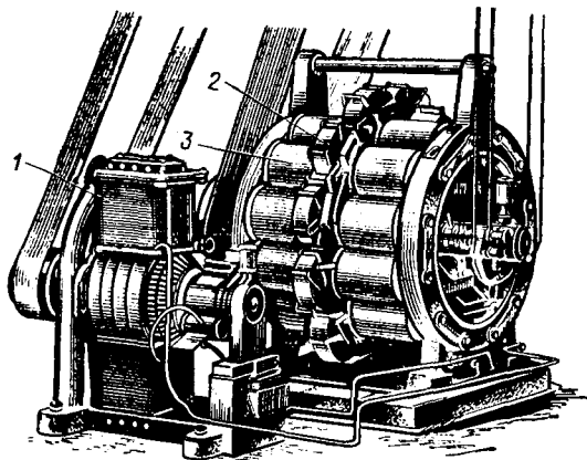
Рис. 6.5. Генератор Сименса:
