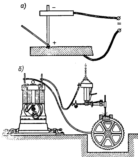
Рис. 7.8. Схема дуговой электросварки: а — по способу Н. Н. Бенардоса; б — по способу Н. Г. Славянова
