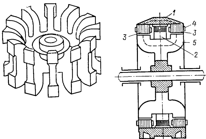
Рис. 9.4. Индукторный генератор:
