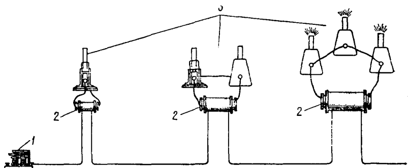
Рис. 6.2. Схема распределения электрической энергии с помощью индукционных катушек: 1 — прерыватель; 2 — индукционные катушки; 3 — электросвечи
