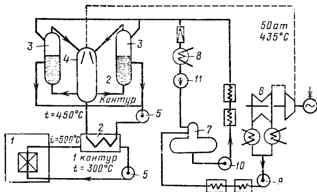
1 — реактор; 2 — теплообменник натрия; 3 — испаритель; 4 — пароперегреватель; 5 — насос для перекачки натрия; 6 — турбогенератор; 7 — диазотер; 8 — технологический конденсатор; 9, 10, 11 — насосы
