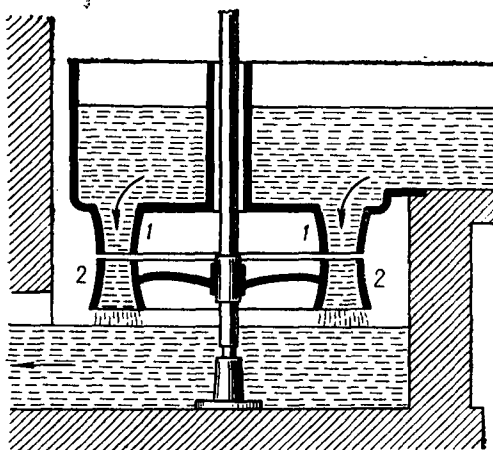
Рис. 3.9. Осовая турбина Геншеля — Жонваля:
