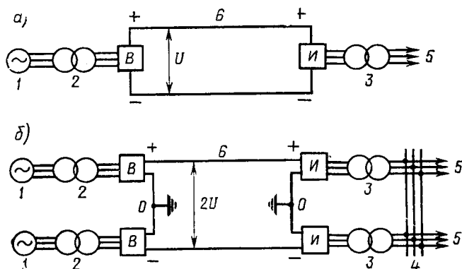
Рис. 8.17. Схемы передачи электроэнергии постоянным током:
