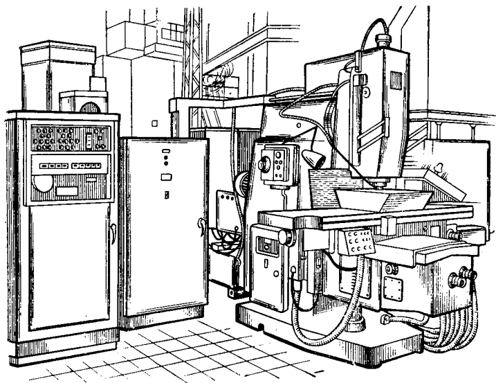
Рис. 9.27. Вертикально-фрезерный консольный станок модели 6P13ФЗ с числовым программным адаптивным управлением
