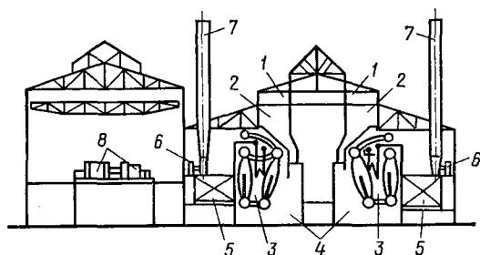
Рис. 8.2. Схема компоновки электростанции «Электропередача»
