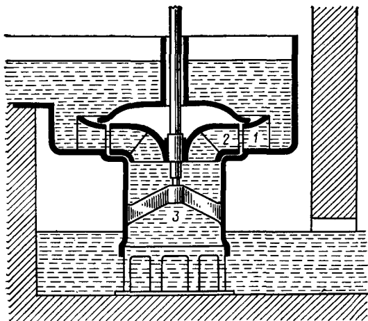
Рис. 3.10. Радиально-осевая турбина (с наружным подводом воды):
