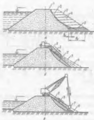
13.2 – rasm. Grunt to'g'onlar qiyaliklarini kengaytirish va yotiqdash sxemalari:
