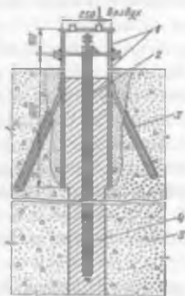
13.14 - rasm. Elektr isitish yordamida asfaltli mastika bilan shponkani qayta tiklash va uni siqilgan havo bilan zichlash: 1 - siqilgan havo bilan shponkani zichlash uchun ogolovka (og'iz); 2 - elektr isitgich; 3 - anker; 4 -shponka; 5 - beton. O'lchamlari mm.da.
