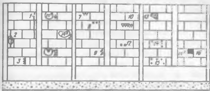
7.2.- rasm. Beton sirtlardagi nuqsonlarning shartli belgilari: 1 - yoriq; 2- oqimi hor yoriq; 3 – quruq g‘uborlanishi bor yoriq; 4- xo‘l dog‘; 5- oq g‘uborlanishi bor ho‘l dog‘; 6 – qoramir g‘uborlanishi bor oqish dog‘i; 7 – zang olib chiquvchi filtratsiya; 8 va 9 –tomchili va struykali oqish; 10 – mastikani oqib chiqishi; 11 – oq quruq dog‘lar; 12 – qoramtir quruq dog‘lar; 13- o‘yiq; 14- plita ostidagi bo‘shliq; 15 – plitani sezilarli yemirilishi; 16- ochilib qolgan armaturasi bilan plitani buzulishi
