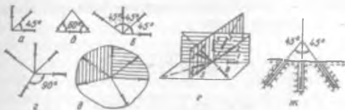
7.13- rasm. Tenzometrik rozetkalar sxemalari:
