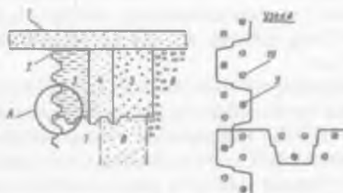
13.6 - rasm. Yadroni betonli tutashtiruvchi devorga tutashgan uchastkasini ta'mirlash: 1 - tutashtiruvchi devor; 2 - shpuntli devor; 3 - glinadan iborat teskari to'kma; 4 - qo'shimcha filtrning teskari to'kmasi; 5 - teskari filtr; 6 - tosh to'kma; 7 - morena suglinokdan yadro; 8 - shag'al toshli filtr; 9 va 10 - sementli va kimyoviy aralashmalarni bosim ostida yuborish uchun skvajinalar.
