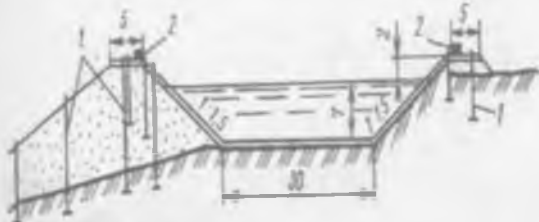
5.1 - rasm. Kanalda pezometrlar va markalarini joylashtirish sxemasi:
