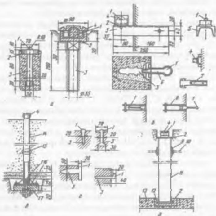
7.3.-rasm. Betonli inshootlarning balandlik murkalari: a – yuza; b – devoriy markalar; v – chuqurlik markasi; g – vaqtinchalik markalar; d – qurilish quvur markasi; 1 – marka; 2 – flans; 3 – tayanch; 4 – qopqoq; 5 – shveller; 6 – shar boshli bolt; 7 – kalit; 8 – korpus; 9 – skoba(qo'sh mix); 10 – armatura; 11,14 – quvurlar; 12 – betonga qotirilgan shtraha; 13 – betonli tayyorlama; 15 – tutashtiruvchi musta; 16 va 17 – metall va beton plita; O'lchamlari mm. da
