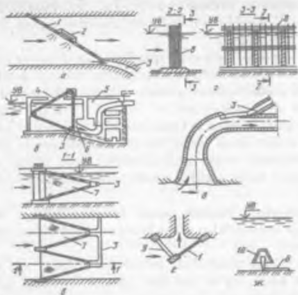
10.3. – rasm Baliqlarni himoya qiluvchi inshootlarning asosiy sxemalari:
