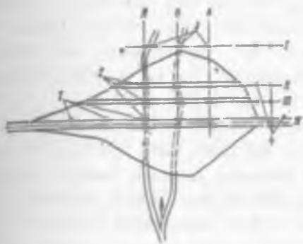
6.10 – rasm. Gruntli to'g'onda markalar va stvor belgilarini joylashtirish sxemasi:
