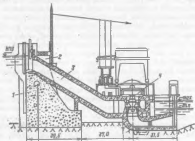
14.6 - rusm. DneproGES to'g'oni chap qirg'oq vodostiv seksiyalarini rekonstruksiya qilish sxemasi: 1 - ilgarigi suv tashlama to'g'on; 2 - ustun; 3 - suv tashigich; 4 - GES binosi. O'lchamlari m da.
