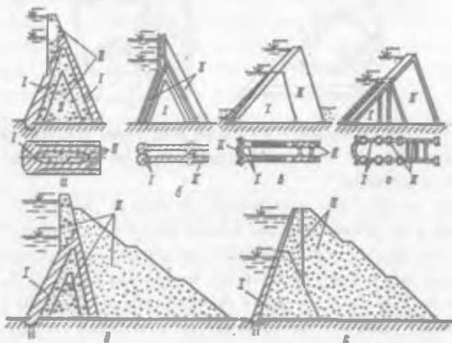
14.7 - rasm. Kontrfors toʻgʻonlarni oʻstirish sxemalari:
