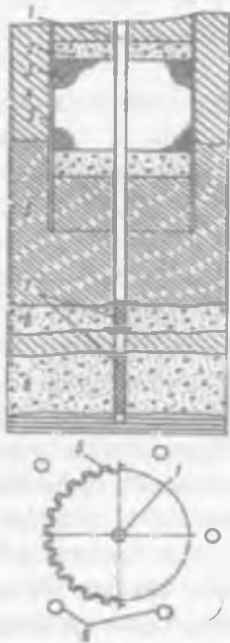
13.10 – rasm. Suv (bosimini) pasaytiruvchi kontakt bo'yicha filtratsiyani bartaraf qilish:
