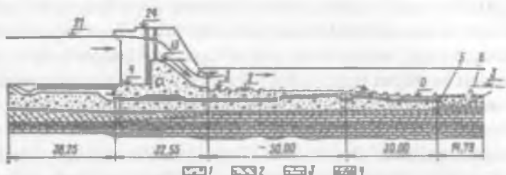
12.3 – rasm. Dnestr daryosidagi Dubossar gidrouzelining suv tashlamasi bo'yicha qirgimi: 1 – shag'al tosh-qumli grunlar; 2 – glinasimon mergel; 3 – o'rtacha zichlikdagi ohaktosh; 4 – mergel; 5 – shpunt; 6 – tubning yuvilishgacha bo'lgan sirti. O'lchamlari m.da
