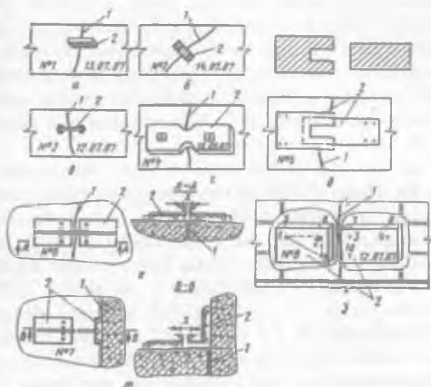
7.7- rasm. Yoriqlarni kuzatish uchun mayaklar: a - gipsli; b va v - organik va oddiy oynadan; g - alebastroli; d - metalli; e , j - I.M.Litvinov konstruksiyalagan mayak; z - F.A.Belyakov konstruksiyalagan mayak ; 1 - yoriq; 2 - mayak.
