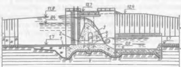
14.3 – rasm. Tezoqarning bosh qismiga qurilgan vodosliv to'g'onining ko'ndalang kesimi: 1 – ponur; 2 – tub oldi suv qo'ygich; 3 – vodosliv; 4 – ko'rish (kuzatish) galereyasi; 5 – pezometr; 6 – argillga o'xshash grunt.
