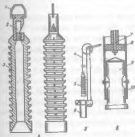
6.15 – rasmi. Pezometrlardagi suv sathini o'lchash uchun asboblari:
