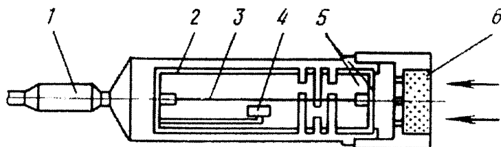
6.6-rasm. Simli pezodinamometr.
