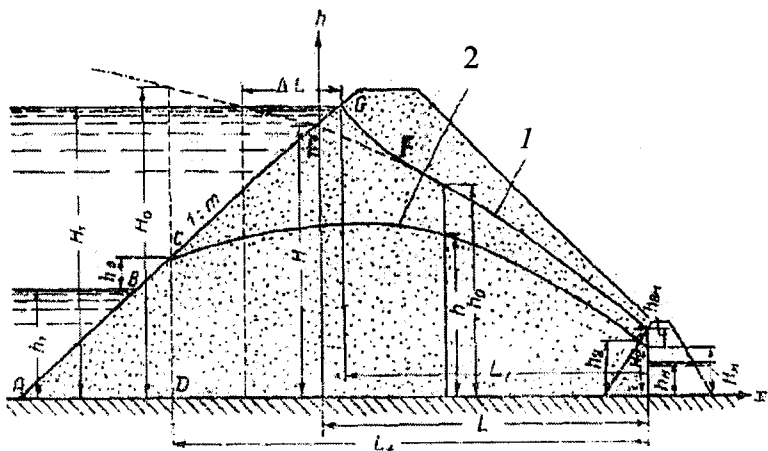
1.2-rasm. Yuqori befdan suv sathi pasayganda to'g'on tanasida depressiya egri chizig'ini holatini hisoblash sxemasi 1-depressiya egri chizig'ini boshlang'ich holati ( t=0 ); 2- depressiya egri chizig'ini hisobiy holati ;
