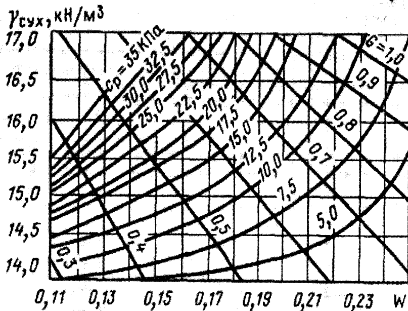
3.3-rasm. Gilli gruntning uzilishdagi tutashuvchanligini aniqlash grafigi
