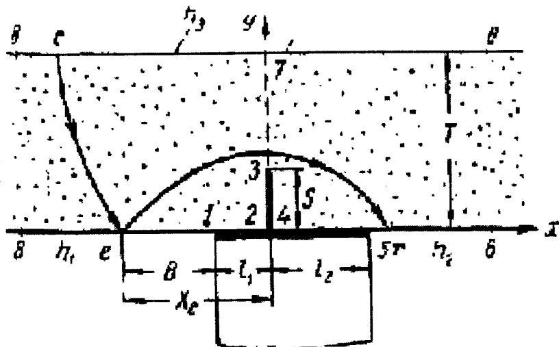
4.2-rasm. Tabiiy grunt suvlari oqimi ta'sirini hisobga olganda, ixtiyoriy joylashgan suv o'tkazmaydigan diafragnali ustun inshootda aylanma filtratsiyani hisoblash sxemasi
