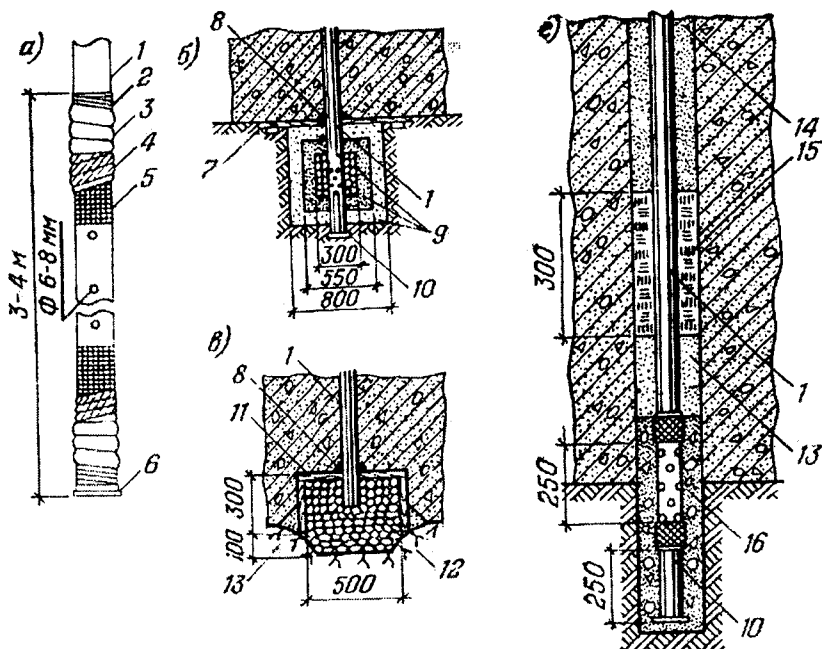
6.5-rasm. Pezometr suv qabul qilish qismi konstruksiyasi
