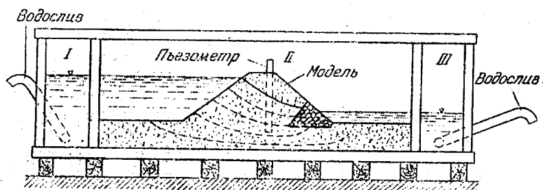
6.1-rasm. Gruntli novni sxemasi.
