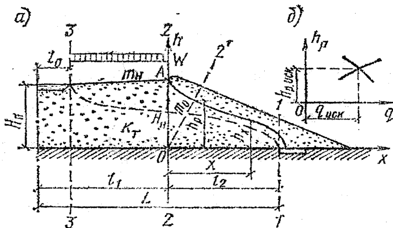
2.5-rasm. Suv o'tkazmaydigan zaminlardagi bir jinsli qavatli drenajli yuvma to'g'oni filtratsiya hisobi sxemasi
