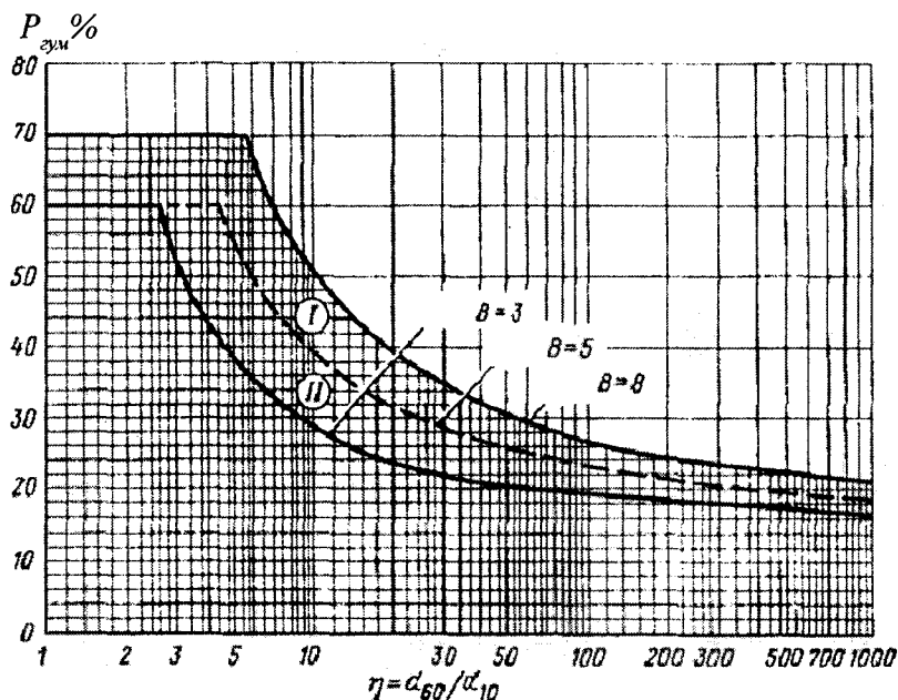
3.7-rasm. Teskari filtr bilan himoyalanganayotgan gumbaz hosil qiluvchi grunt zarrachalarini hisobiy o'lchamlarini aniqlash grafigi
