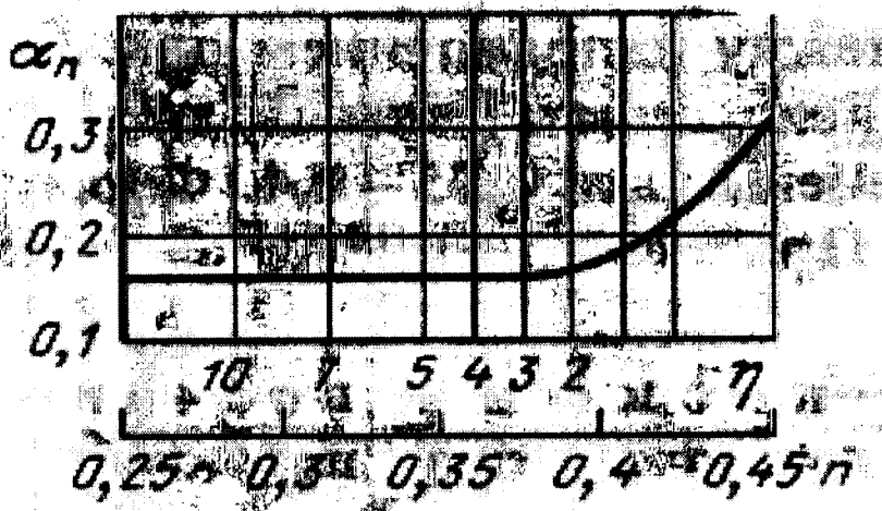
3.4-rasm. \alpha_n ni aniqlash grafigi
