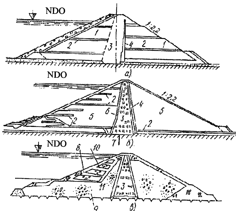
1.15-rasm. To'g'on ko'ndalang kesimlari
