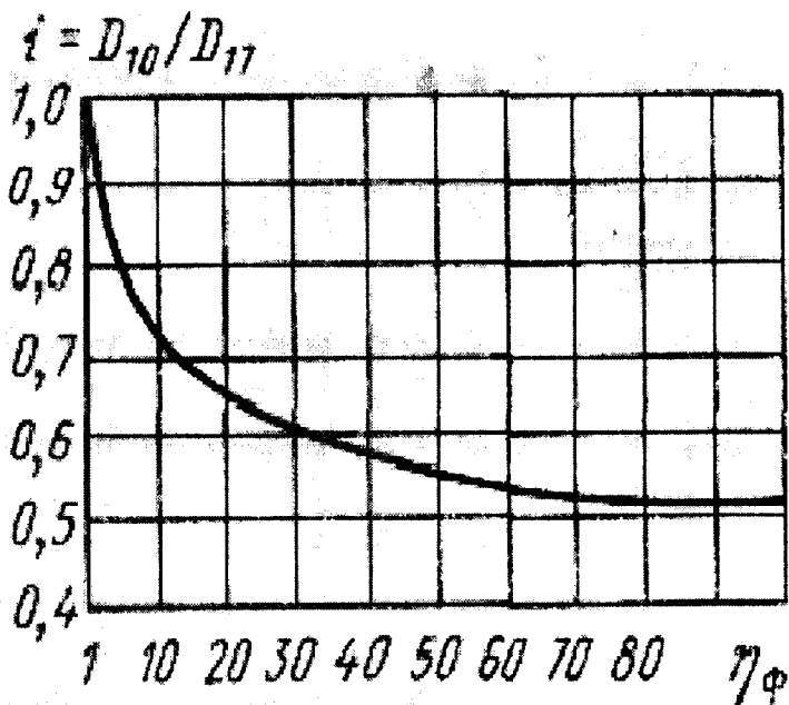
3.11-rasm. \eta_\phi = f(i) grafigi.
