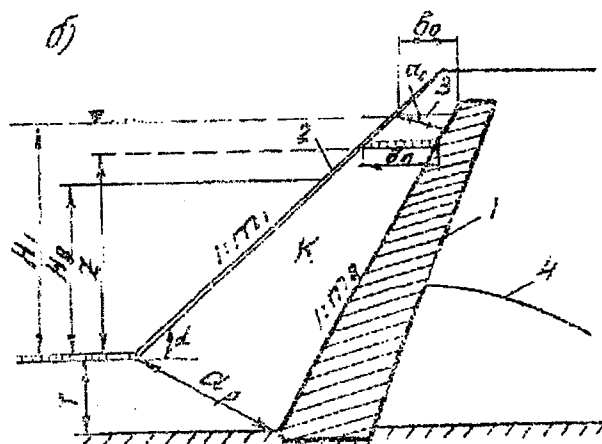
1.9-rasm. To'g'on yuqori qiyaligi qoplamasi tubidagi qumli qatlamda noturg'un filtratsiyani hisoblash sxemasi
