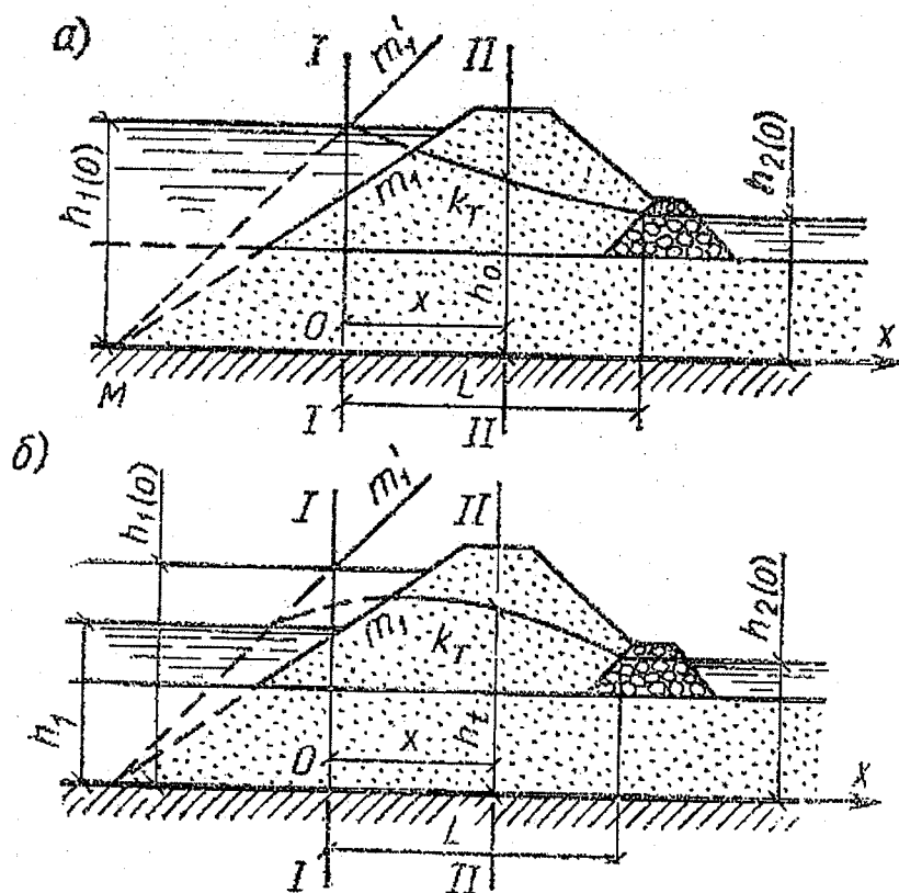
1.8-rasm. Bir jinsli suv o'tkazuvchi zamindagi drenaj prizmati to'g'unda noturg'un filtratsiya hisobi
