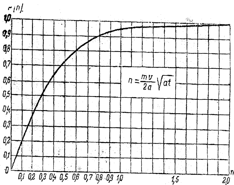
1.4-rasm. P(n) miqdorini aniqlash grafigi
