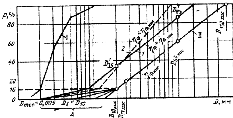
3.12-rasm. Gruntni hisobiy tarkibi grafigi va birinchi qavat filtri donadorlik tarkibini yo'l qo'yilgan oralig'ini belgilash.
