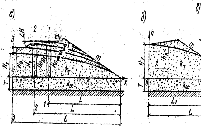
2.9-rasm. Suv o'tkazuvchi zamindagi bir jinsli drenajsiz yuvma to'g'onda depressiya egri chizig'ini pasayish tezligini hisoblash sxemasi
