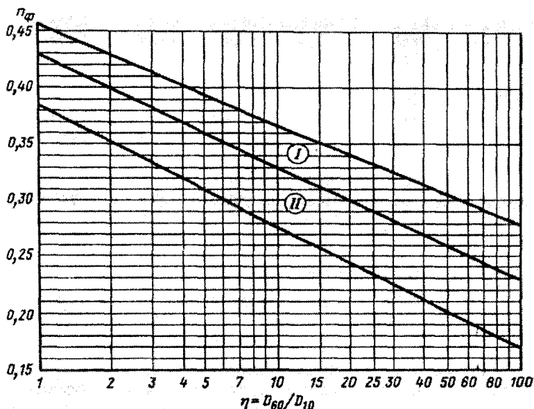
3.9-rasm. Teskari filtr gruntlarini yo'l qo'yilgan g'ovakligi n_\phi ni aniqlash grafiqi. I - shebenli grunt uchun; II - qum, mayda va yirik shag'al gruntlar uchun.
