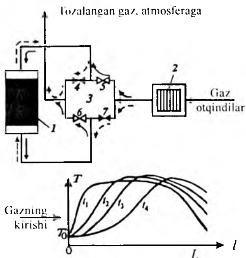
6.22-rasm. Noturg'un rejimda gaz o'tqindilarini zararsizlantirish qurilmasining sxemasi va katalizator qatlamida uzunlik l bo'yicha harorat ( T ) ning vaqt bo'yicha o'zgarishi ( t_1 \dots t_4 ): 1—katalitik reaktor, 2—ishga tushiruvchi isitgich; 3—uzib ulovchi klapanlar bloki (4–7). Tutash va uziq chiziqlar – jarayonning turli sikllarida oqimning yo'nalishlarini ko'rsatadi
