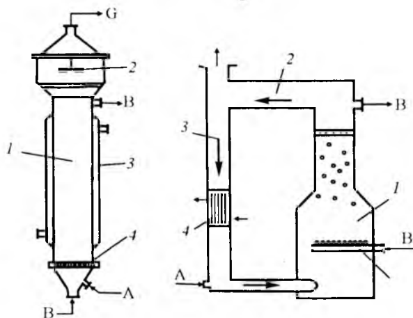
3.23-rasm. Fermenterlar sxemalari:
