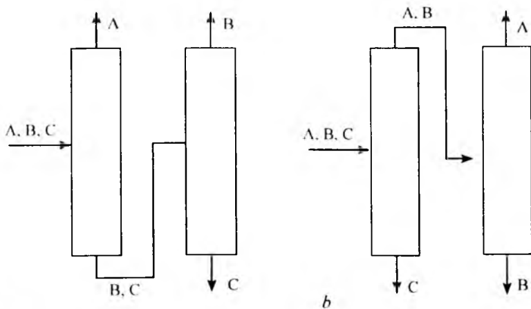
5.48-rasm. Uchkomponentli aralashmani ajratib olish sxemasi. (Izox mavzu ichida berilgan)
