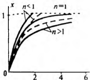
2.44-rasm. C_0 ning x(\tau) ga n tartibli reaksiya uchun ta'siri. Uzluksiz ehiziq C_{01} da, punktir -C_{02} > C_{01} bo'lganda.
