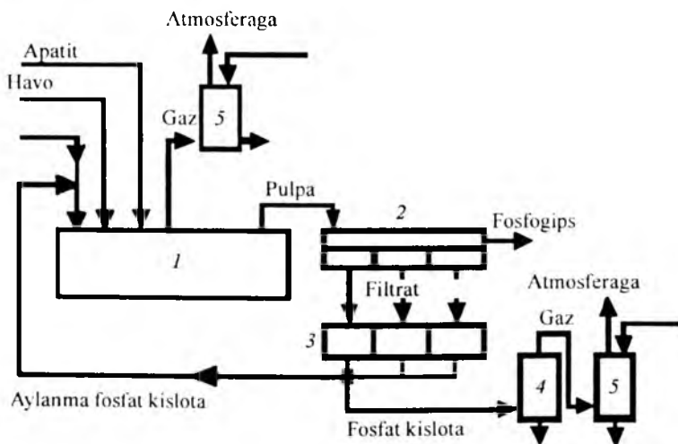
4.48-rasm. Ekstraksiya fosfat kislotasi ishlab chiqarish funksional sxemasi:
