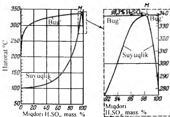
4.4-rasm. Sulfat kislota suvli eritmasining 0.98 MPa bosimda qaynash diagrammasi.
