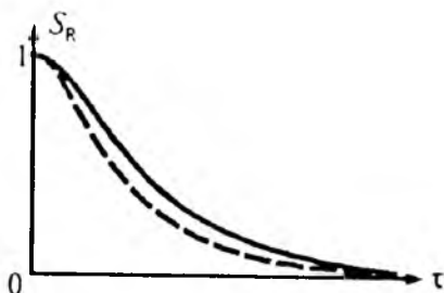
2.50-rasm. Integral selektivlik S_R \tau ga bog'liqligi (ketma-ket reaksiyada). Uzlaksiz chiziq – T_1 temperaturada, punktirda – T_2 > T_1 va E_1 > E_2 bo'lganda.
