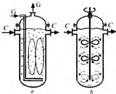
2.56-rasm. Kolonnali reaktorlardagi sirkulyatsion oqimlar.
