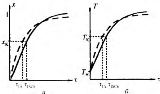
2.68-rasm. x(\tau) (a) va T(\tau) (b)larning oqim reaktorida ISCh (yaxlit chiziqlar) va IA ning adiabatik reaktorlarda (punktir) bog'liqligi.
