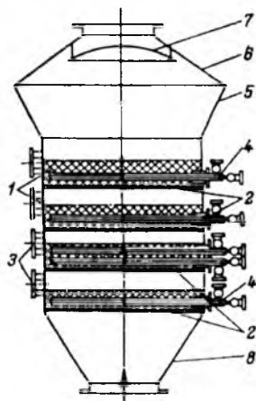
4.18-rasm. Qaynama qatlamli kontakt massali kontakt apparati: 1 – kontakt massa; 2 – gaz taqsimlaydigan panjara; 3 – darcha (lyuklar); 4 – sovutgich; 5, 8 – diffuzorlar; 6 – konfuzor; 7 – otboynik.
