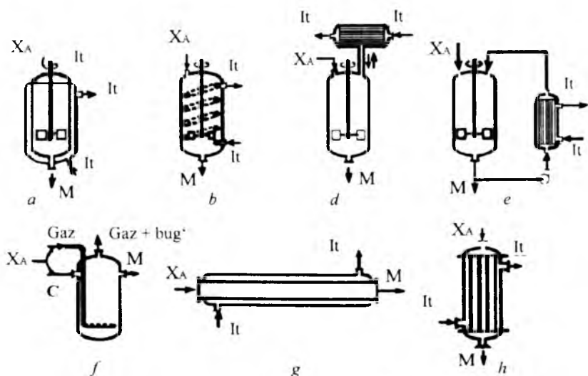
2.59-rasm. Kimyoviy reaktorlardagi reakcion zonada issiqlik almashinishini tashkil etish. X_A – xomashyo; M – mahsulot; It – issiqlik tashitgich.
