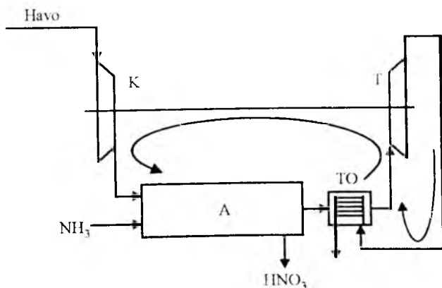
5.25-rasm. Tebranma rejimlarni (azot kislotasini ishlab chiqarishda) amalga oshirish imkoniyati bo'lgan kimyoviy texnologik tizim.
