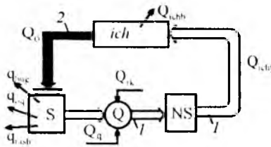
6.8-rasm. Ishlab chiqarishni suv bilan ta'minlashning yarim berk tizimi:
