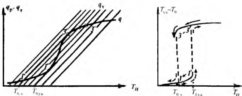
2.39-rasm. G'ovaksiz katalizator donasidagi noizotermik jarayonning stasionar rejimlari. q_p , q_r ( T_{yu} ) (a) diagrammasi va yuza temperaturasi T_{yu} ning oqim temperaturasi T_0 (b) bilan o'zgarishi.
