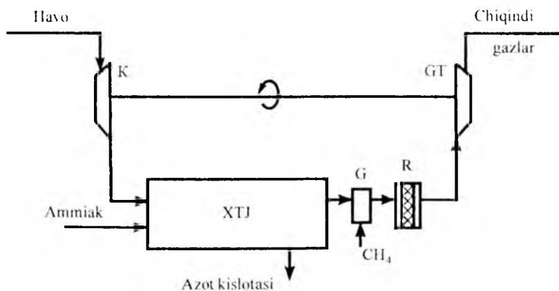
5.39-rasm. Azot kislotasi ishlab chiqarishdagi energotexnologik sistema: R – tozalash reaktori (qolgan ifodalar 5.36-rasmdagi singaridir). XTJ – kimyo- texnologik jarayoni.
