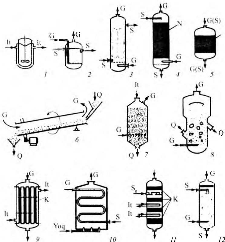
2.1-rasm. Kimyoviy reaktorlar sxemalari: G – gaz, suyuqlik; Lt – issiqlik tashigich; N – nasadka, Q – qattiq reagent; K – katalizator, S_g – sovuq gaz.
