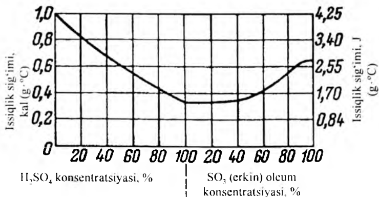
4.5-rasm. Sulfat kislota va oleumning issiqlik sig'imi.
