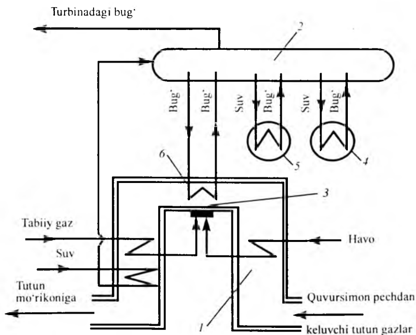
4.39-rasm. Ammiakni sintez qilish agregatining energotexnologik tizimi: 1–quvursimon pechdan keyingi gaz yo'li; 2–bug' to'plagich; 3–qo'shimcha gorelka; 4–5–utilizator-qozonlari (shaxtali metan konvertoridan va tegishli SO konversiyasidan keyingi); 6–yordamchi qozon.
