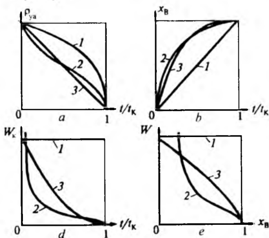
2.27-rasm. t vaqt ichida yadro \rho_{ya}(a) kattaligi, qattiq reagentning x_B(b) aylanish darajasi, kuzatilgan aylanish tezligi W_k(d) ning o'zgarishi va W_k(x_B) ning «siqiluvchi yadro» geterogen jarayonga boqliligi.
