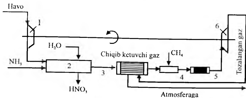
4.47-rasm. Azot kislotasi ishlab chiqarishda energotexnologik tizim: 1–kompressor; 2–texnologik apparatlar; 3–issiqlik almashtirgich; 4–gaz gorelkasi; 5–katalitik tozalash reaktori; 6–gaz turbinasi.
