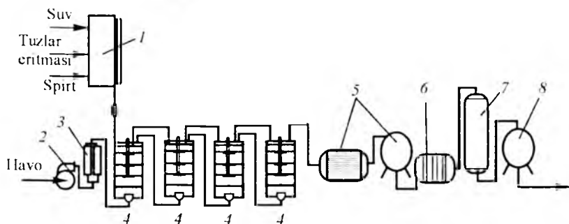
3.21-rasm. Spirtidan sirka kislotaga ishlab chiqarish texnologik sxemasi:
