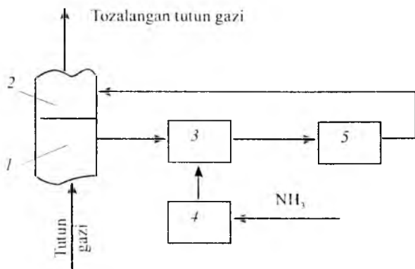
6.24-rasm. Tutun gazlarini azot oksidlaridan tozalash sxemasi: 1–dudburon; 2–to'siq; 3–ammiakni tutun gazi bilan aralashtirgich; 4–ammiakni dozalash bloki; 5–reaktor.
