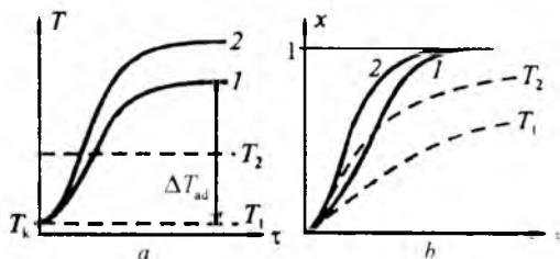
2.62-rasm. Temperatura T (a) va aylanish darajasi x (b) ning ISCh rejimidagi profilari. Uzluksiz chiziqlar – T_{ad} (1) va T_{ad} > T_{ad} (2) bo'lganda ekzotermik adiabatik jarayon; punktir chiziqlar – T_1 va T_2 temperaturalardagi izotermik jarayon.
