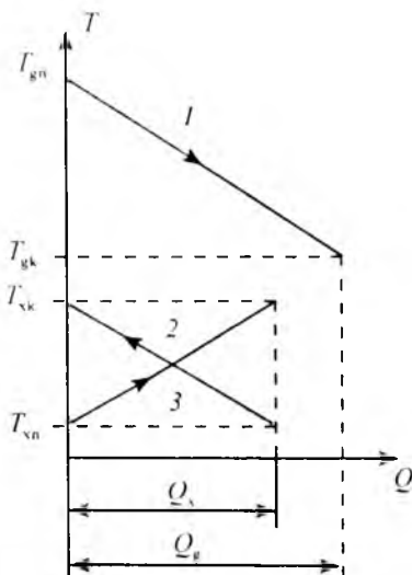
5.49-rasm. Sovutiladigan (1) va isitiladigan (2, 3) oqimlarning « Q – T » diagrammasi.
