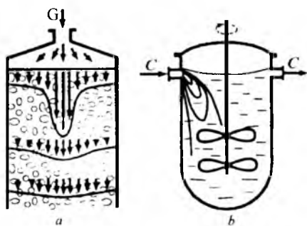
2.57-rasm. Reaktorga oqim kirishida uning bir jinsli tarqalmasligi donador qavatda ( a ) va aralashtiriluvchi suyuqlik reaktorida ( b ) ko'rinishi.
