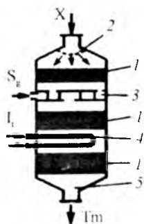
2.2-rasm. Reaktorning strukturaviy elementlari: 1 – reaksiya zona; 2 – reaksiya aralashma kirishi uchun moslama; 3 – aralashtirgich; 4 – issiqlik aralashtirgich; 5 – chiqish moslamasi; S_g – sovuq gaz; I_i – issiqlik tashigich; X va Tm – tegishli xomashyo va tayyor mahsulotlar.
