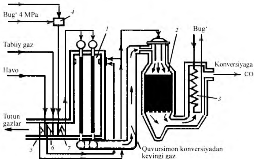
4.32-rasm. Metan konversiyasining texnologik sxemasi:
