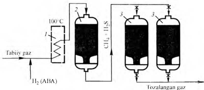
4.30-rasm. Tabiiy gazni oltingugurt tarkibli birikmalardan tozalashning texnologik sxemasi: 1 – choʻgʻlanma isitgich; 2 – gidrirlash reaktori; 3 – absorberlar – azotovodorod AVA li aralashma.
