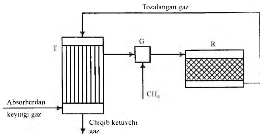
5.41-rasm. Qo'shimcha isitish orqali gazni tozalash sxemasi:
