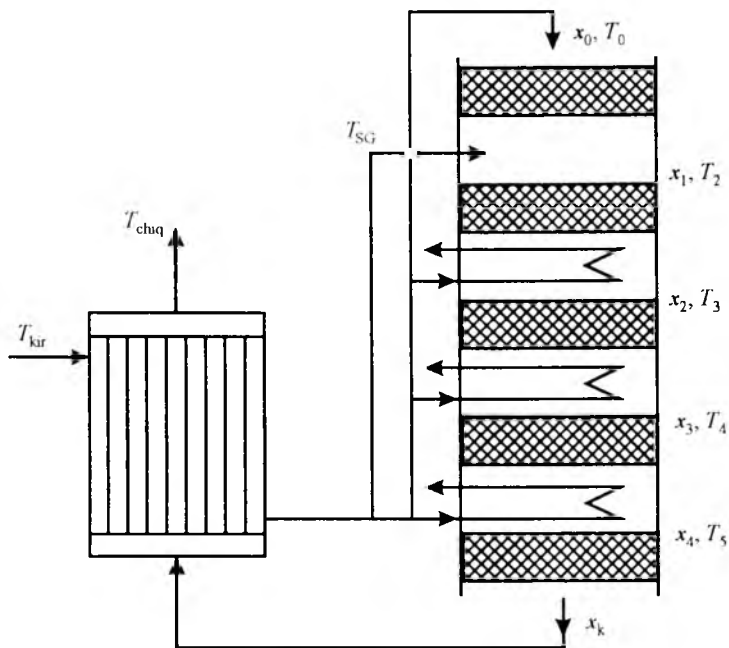
5.17-rasm. Oltingugurt dioksidi oksidlanish jarayonining reaksiyon uzeli.
