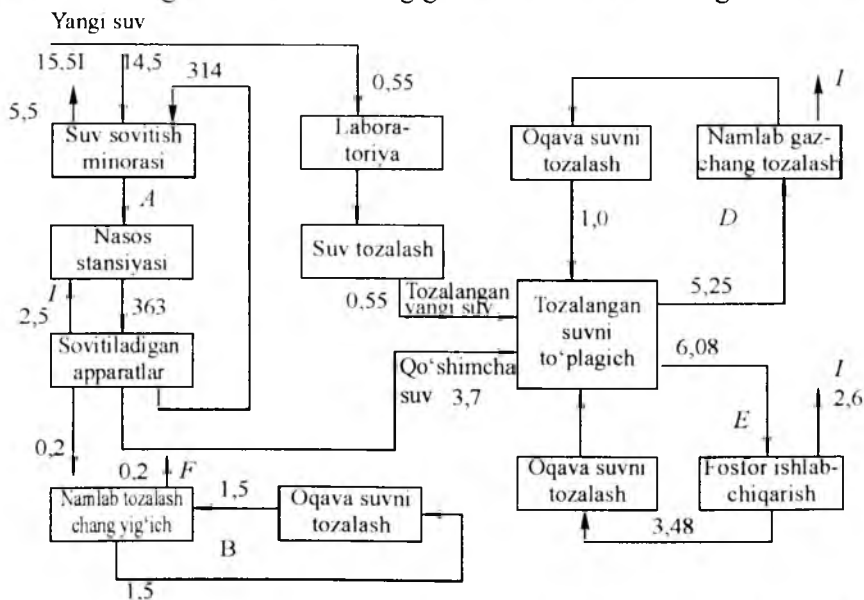
6.12-rasm. Oqimsiz fosfor ishlab chiqarishda suv oqimlari va suv aylanishi sxemasi (raqamlar m³/soat hisobidagi sarfni ko'rsatadi):
