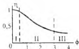
2.33-rasm. Katalizator ichki yuzasining ishlatilish darajasi \eta ning \phi parametrga bog'liqligi. Punktirlar – rejimlarning taxminiy chegaralari: I – kinetik; II – o'rtinchi; III – ichki diffuzion.
