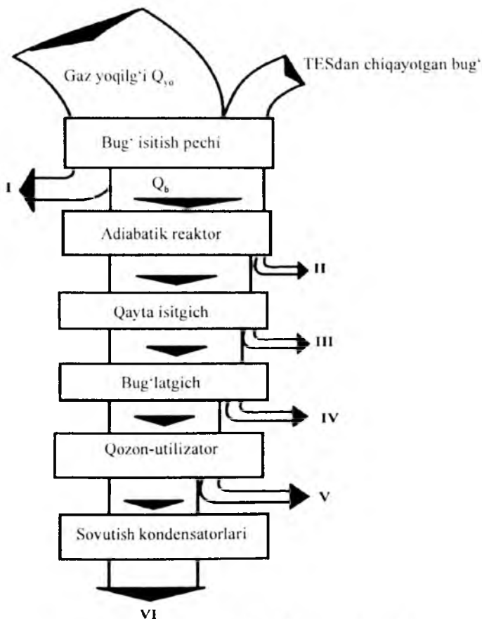
3.14-rasm. Etilbenzolni degidirlash agregatidagi issiqlik oqimlarining diagrammasi: I –bug' isitgich pechidagi tutun gazlaridan yo'qoluvchi issiqlik; II –degidirlashdagi endotermik reaksiya kompensatsiyasi; III –etilbenzol shixtasini isitish; IV –etilbenzolni bug'latish; V –suv bug'ini generirlash; VI –sovutish havosi va xladagent bilan atrof-muhitga tarqaluvchi issiqlik.
