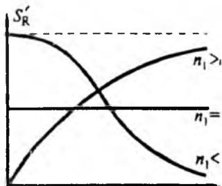
2.20-rasm. Differensial selektivlik S'_R -ning aylanishning parallel sxemasi ( n -reaksiya tartibi) uchun konsentratsiya S_A ga bog'liqligi.
