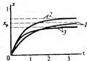
2.46-rasm. T_1 (1) va T_2 > T_1 (2, 3) temperaturalarda x(\tau) ning bog'lanishi. Reaksiyalar: endotermik (2) va ekzotermik (3). Punktir – x_M ning mazkur sharoitlar uchun aylanishining muvozanat darajalari.
