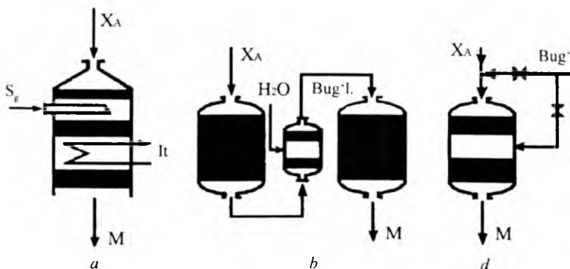
2.60-rasm. Ko'p qavatli reaktorlarda va ketma-ket reaktorlarda oraliq issiqlik almashinishini tashkil etish. X_A , M , It – 2.59-rasmdagidek. S_k – sovuq gaz. Bug'l. – bug'latgich.
