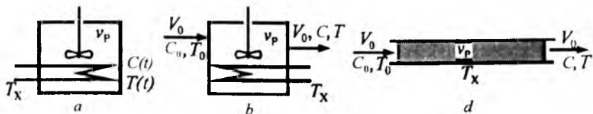
2.40-rasm. Reaktorlar sxemasi: a – ideal aralashish rejimidagi davriyligi (IA-d); b – ideal aralashishning oqimiligi (uzluksiz) (IF-u); d – ideal siqib chiqaruvchi (ISCh).
