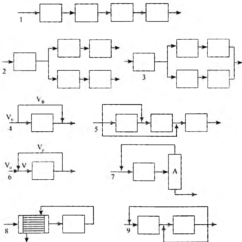
5.2-rasm. Kimyoviy-tehnologik sistemadagi bog'lanishlar: 1 – ketma-ket; 2 – tarmoqlangan; 3 – parallel; 4, 5 – aylanma (baypas) – oddiy (4) va murakkab (5); 6–9 – teskari (retsirkulyatsion); to'la retsiki (6, 9) va fraksiya (7, 8); oddiy (6) va murakkab (9); A – ajratish sistemasi
