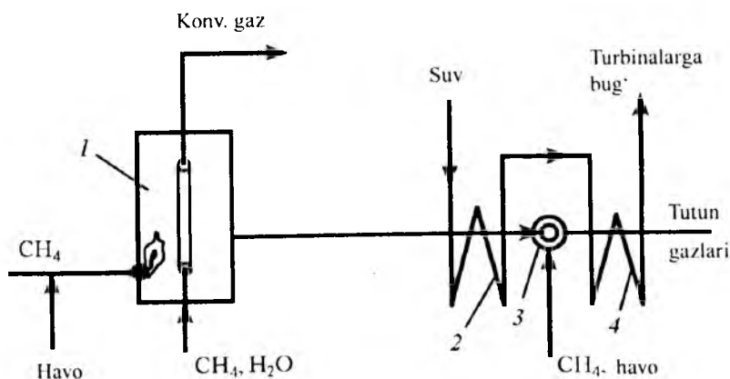
5.40-rasm. Ammiak ishlab chiqarishning energotexnologik sxemasi: 1 – metanni konversiyalash quvursimon pechi; 2 – utilitatsiyalovchi qozon; 3 – gorelka; 4 – bug'ni isitkich.
