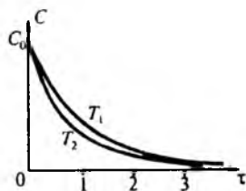
2.43-rasm. Temperatura T ning C(\tau) ( T_2 > T_1 ) ga bog'liqligi.
