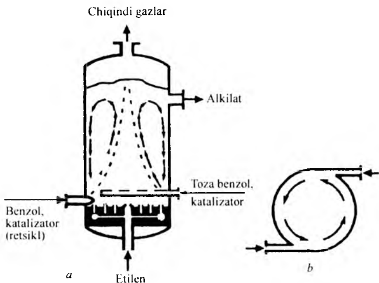
3.10-rasm. Benzolni etilen bilan alkilash reaktori:
