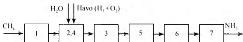
5.3-rasm. Ammiak ishlab chiqarishning funktsional sxemasi. Sxemadagi sonlar operatsion model bosqichlariga mos keladi.
