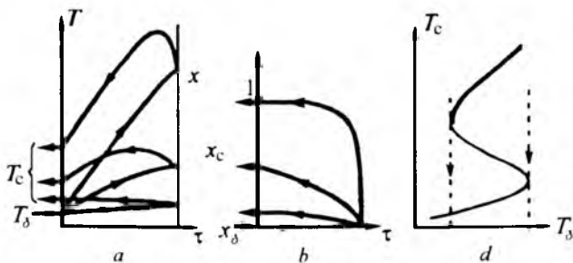
2.70-rasm. Avtotermik reaktordagi statsionar rejimlar.
