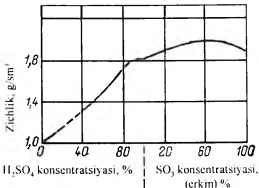
4.3-rasm. Sulfat kislota va oleumning 20°C dagi zichligi.
