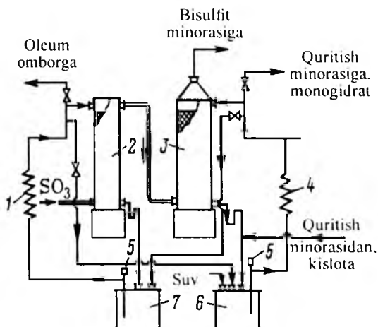
4.21-rasm. Absorbsion bo'lim sxemasi: 1—oleum sovutgichi; 2—oleum absorberi; 3—monogidrat absorberi; 4—monogidrat sovutgichi; 5—cho'ktiriladigan nasoslar; 6—monogidrat yig'gichi; 7—oleum yig'gichi.
