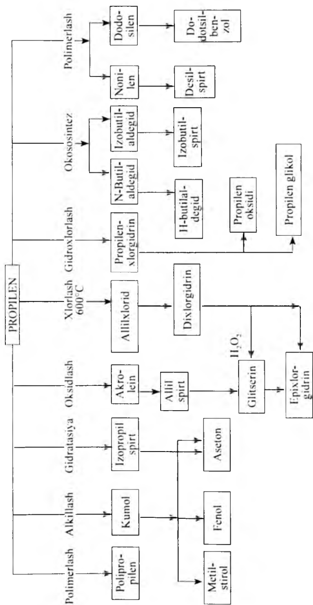
3.7-rasm. Propilenni qayta ishlashning asosiy yo'nalishlari.
