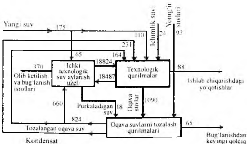
6.11-rasm. Neftni qayta ishlash zavodida suvdan foydalanish sxemasi (raqamlar m^3 /soat hisobidagi sarfni koʻrsatadi).
