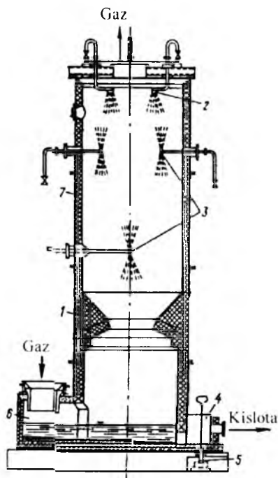
4.14-rasm. Ichi bo'sh yuvish minorasi: 1—minora korpusi; 2, 3—kislota ni changlantirgichlar; 4—kislota olib ketish qutisi; 5—shlamni chiqarib yuborish uchun nov (tarnov); 6—gaz kiritish uchun quti; 7—qoplama.
