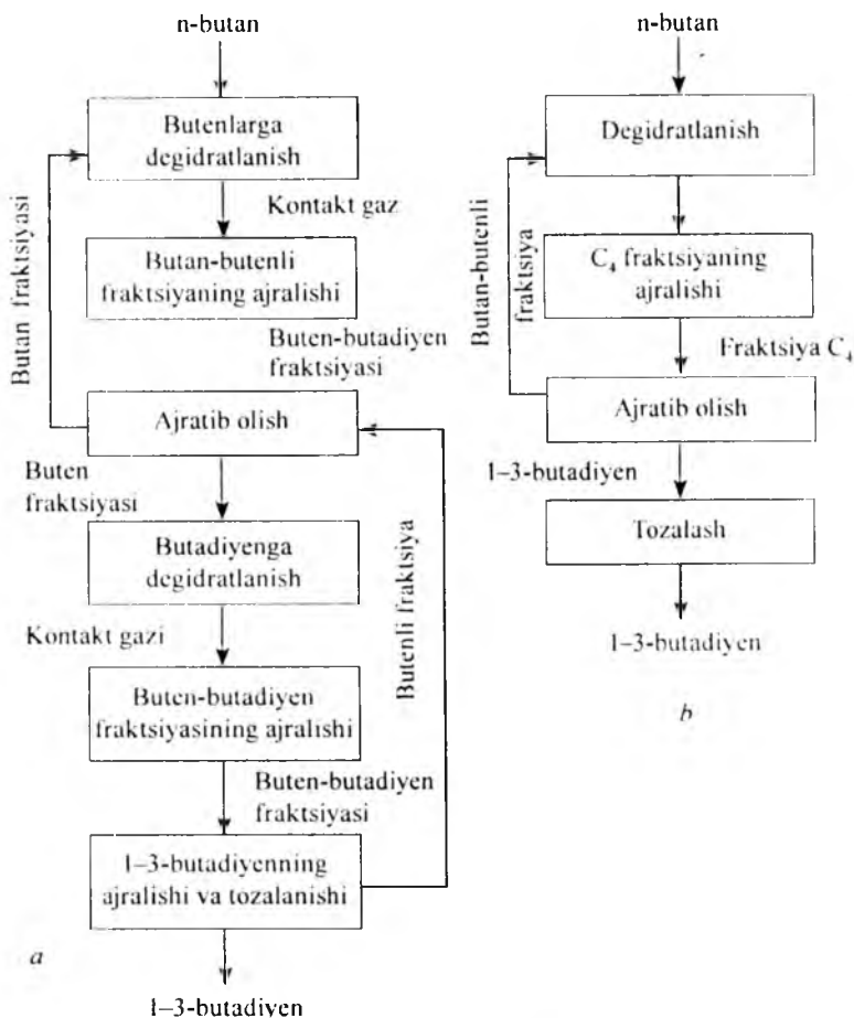
5.38-rasm. n-butanning divinilga (1,3-butadiyen) ikki bosqichda (a) va bir bosqichda (b) degidratlanish sxemasi.
