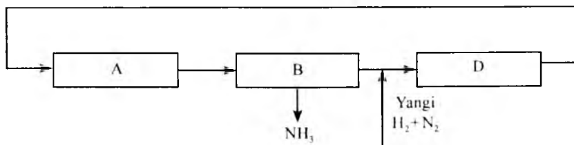
5.5-rasm. Ammiak sintezi funktsional sxemasi:
