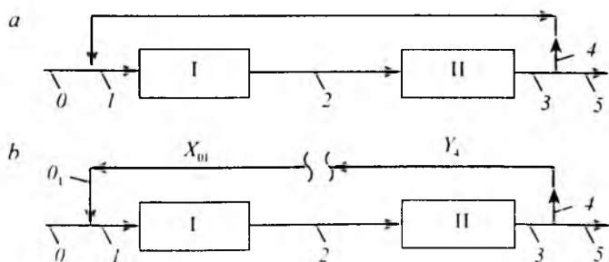
5.19-rasm. Retsikli KTS strukturası: dastlabkisining (a) va hisobiy (b) sxemalari.
