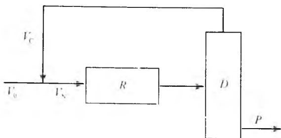
5.24-rasm. Fraktsion retsiklli sistema (statsionar rejimlarning mavjudligini aniqlashga doir): R – reaktor; D – mahsulot ajratish sistemasi; P – mahsulot.
