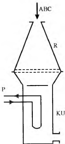
5.43-rasm. Ammiakni oksidlash reaktori (R) va utilizatsiyalovchi qozonni (KU) konstruktiv o'rindoshlash sxemasi:
