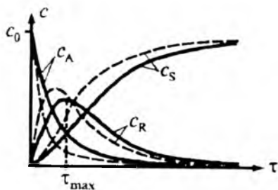
2.49-rasm. ISCh reaktori yoki (IA-d) reaktorida ketma-ket reaksiya o'tishidagi reagentlar konsentratsiyalarining o'zgarishi. Uzlaksiz chiziqlar – T_1 temperaturada, punktirda – T_2 > T_1 va E_1 > E_2 bo'lganda.
