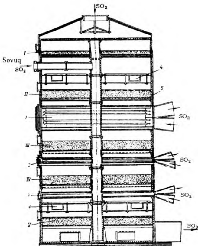
4.16-rasm. Birinchi qatlamlardan keyin sovuq gaz qo'shildigan kontakt apparat:
