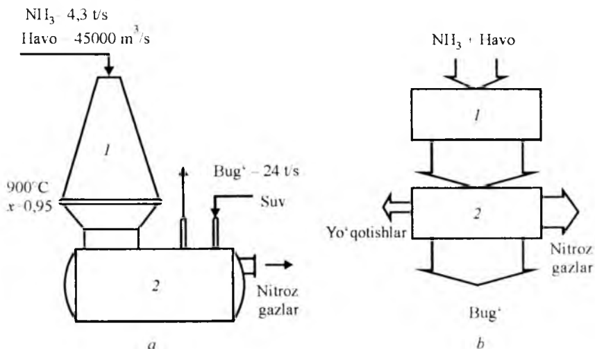
5.20-rasm. Ammiakning oksidlanish uzeli oqimining ko'rsatkichlari (a) ko'rsatilgan texnologik sxemasi va uning issiqlik diagrammasi (b): 1 – reaktor; 2 – utilizator-qozon.
