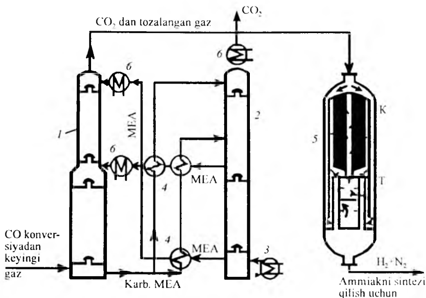
4.34-rasm. CO 2 dan (MEA-tozalash) va CO dan (metanlash) tozalashning texnologik sxemasi:
