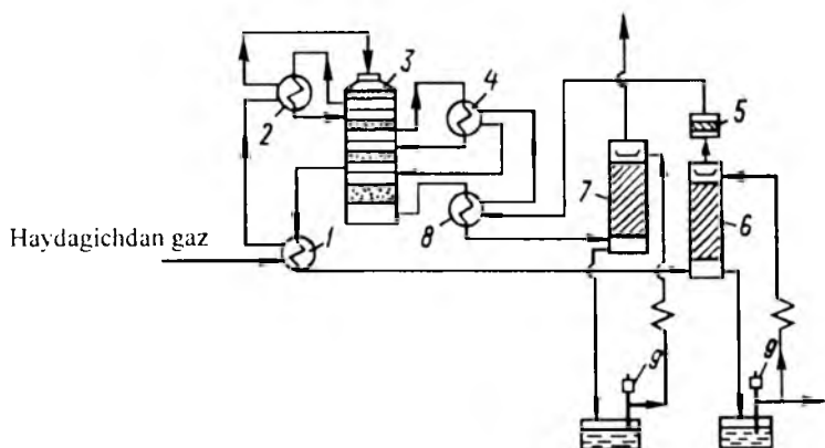
4.22-rasm. Qo'sh kontaktlashadigan kontakt bo'limi:
