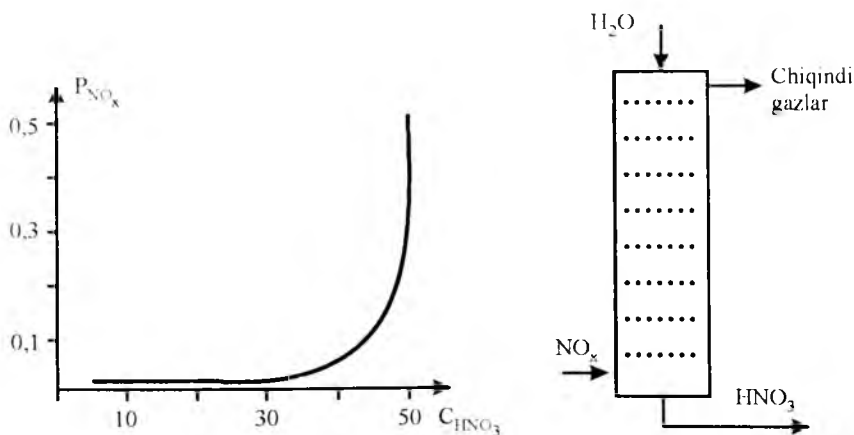
5.31-rasm. \text{HNO}_3 eritmasi ustidagi azot oksidlarining muvozanatda bo'lgan parsial bosim \text{NO}_x(P_{\text{NO}_x}) ning uning konsentratsiyasi ( C_{\text{HNO}_3} ) ga (a) bog'liqligi va adsorbsion kolonna (b) sxemasi.
