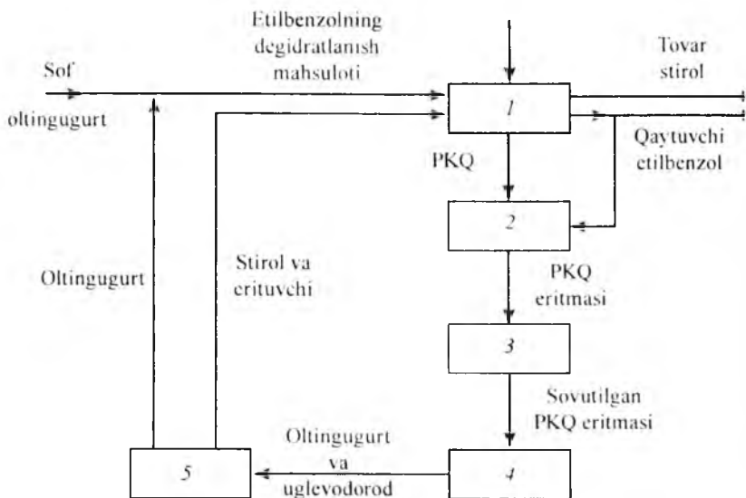
5.33-rasm. Reagentlarni regeneratsiyalash bilan stirol ishlab chiqarish sxemasi:
