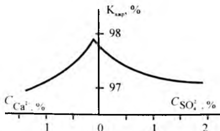
4.49-rasm. Fosforni ajratib olish darajasi K_{\text{af}} ning \text{Ca}^{2+} va \text{SO}_4^{2-} ionlarining ortiqcha miqdoriga bog'liqlik grafigi.
