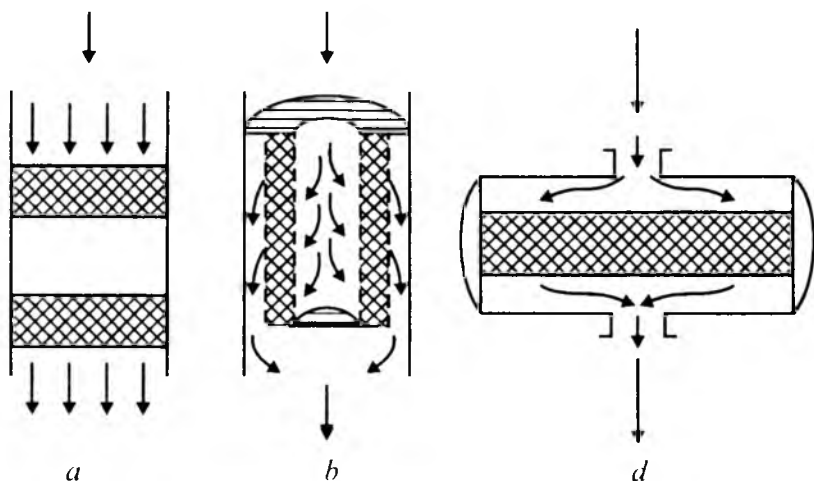
5.42-rasm. Katalizator aksial (a), radial (b) va gorizontaal (d) qatlamlar tarzida joylashuvchi reaktor.
