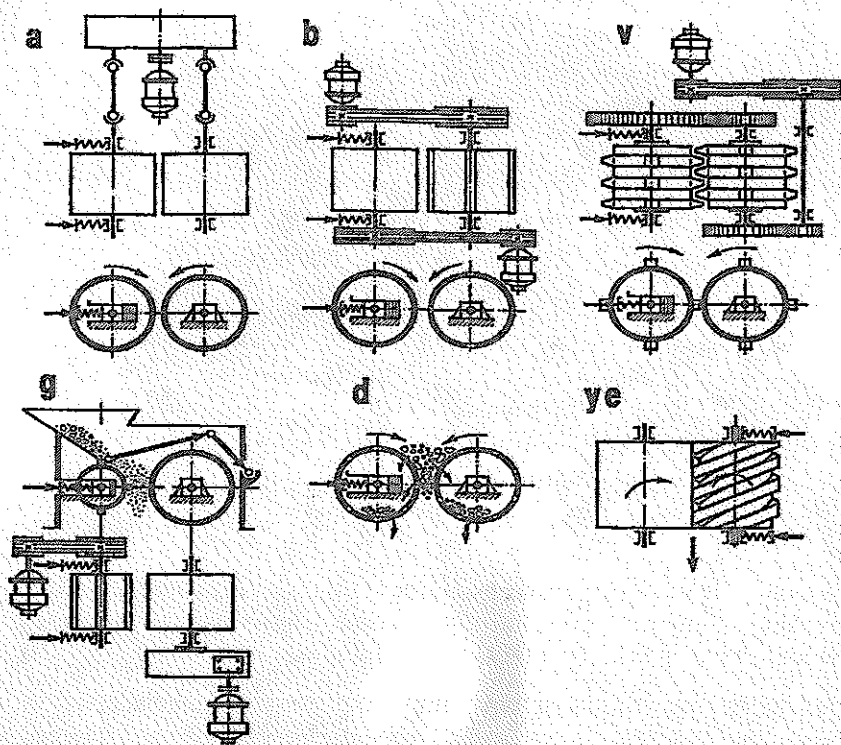
6-rasm. Valli maydalagich: a-yuzasi tekis valli, b-yuzasi notekis valli, v- yuzasi tish bilan qoplangan valli, g - tekis-notekis valli, d - teshik valli, ye - vint yuzaga ega valli.
