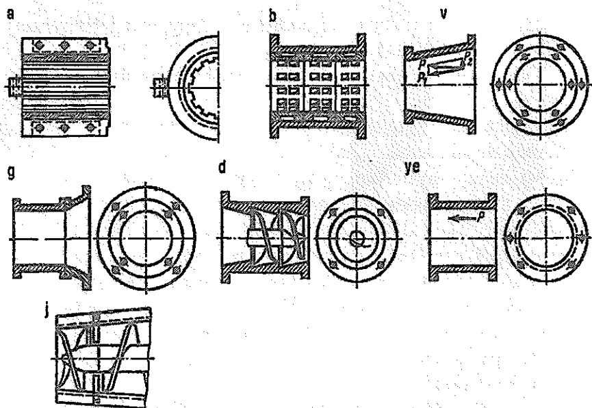
24- rasm. Lentasimon pressning qismlari: a - shtirli tana, b - rifli tana, v - konussimon tana, v - konussimon tana, g-kombinatsiyalashgan tana, d-ponasimon tana, j-silindrsimon tana.
