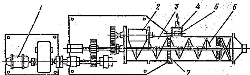
28-rasm. Vakuumli pressning chizmasi: 1- elektruyuritgich, 2 - oziqllovchi val, 3 - dastlabki siqish kamerasi, 4- vakuum-quti, 5 - valcha, 6 - shnek, 7- g'alvirsimon panjara.
