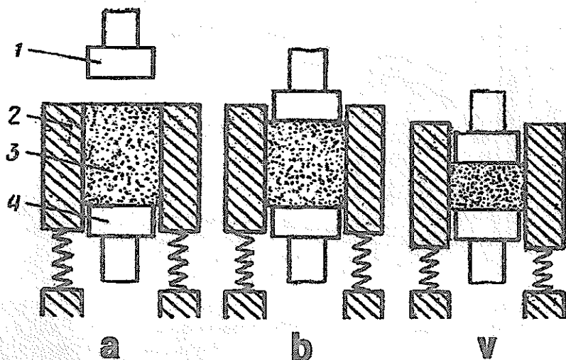
36-rasm. Qo'zg'aluvchi shtamp bilan shakllantirish sxemasi:
