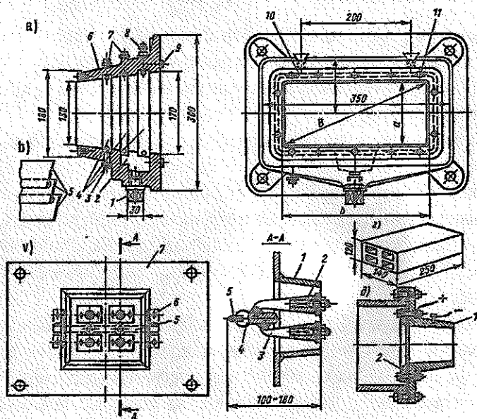
27-rasm. Lentasimon presslarning mundahtuklari: a-normal konstruksiyali mundahtuk, b-ichki qoplama, v-to'rt teshikli mundahtuk, g-4 ta teshikli g'isht, d-bug' bilan isitiladigan mundahtuk, 1-po'lat list, 2-nasadka, 3-kernlar, 4-kern tutech.
