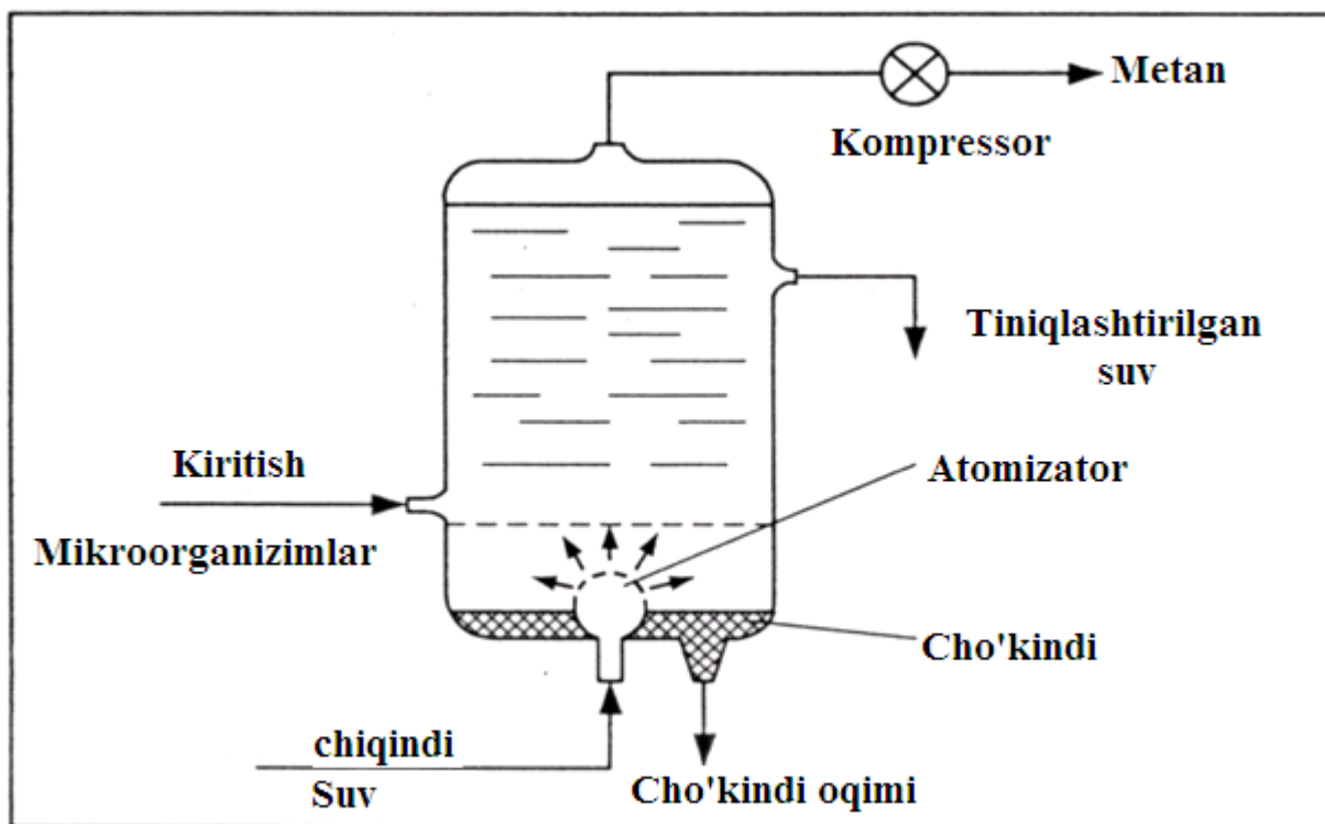
1- rasm Anaerob reaktorini prinsipial sxemasi
