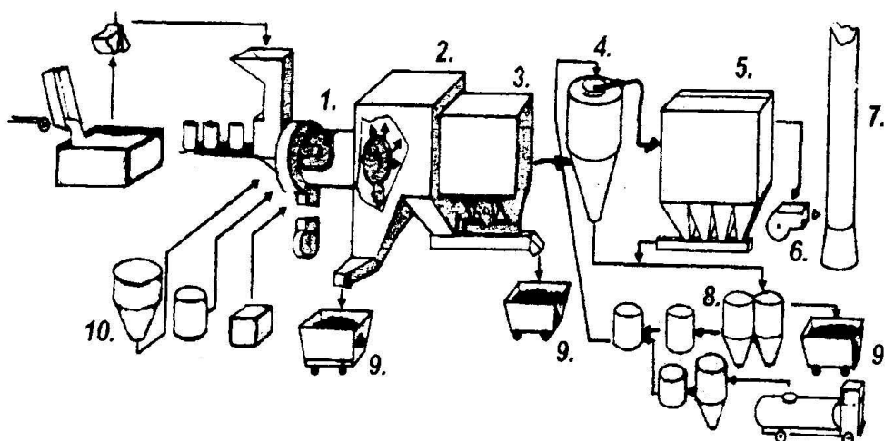
14- rasm. Ecokem (Finlyandiya) poligonidagi zahar chiqindilarni yeqish qurilmasi sxemasi
