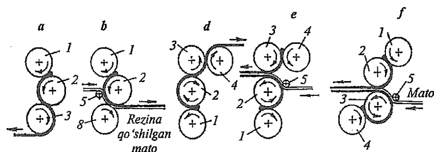
22-rasm. Rezina buyumlarni vulkanlash.
