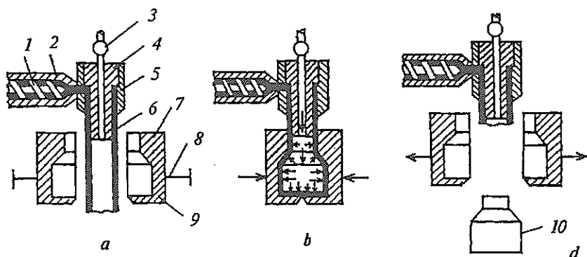
20-rasm. Ekstruziya usulida puflab ichi havol idishlar olish sxemasi:
