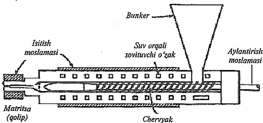
3-rasm. Ekstruder sxemasi.
