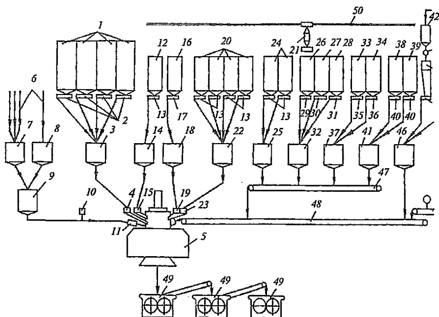
21- rasm. Rezina aralashmasini tayyorlash texnologik sxemasi:
