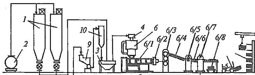
11-rasm. Termoplastlardan ekstruziya usuli bilan list ishlab chiqarish texnologik sxemasi:
