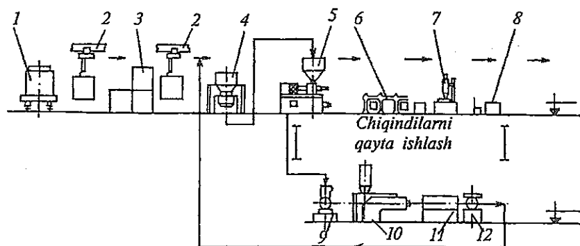
13-rasm. Termoplastlardan quyish usuli bilan buyum olish texnologik sxemasi:
