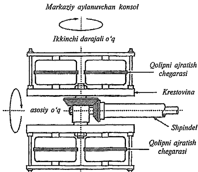
18- rasm. Ikki o'qli rotatsion shakllash moslamasi.
