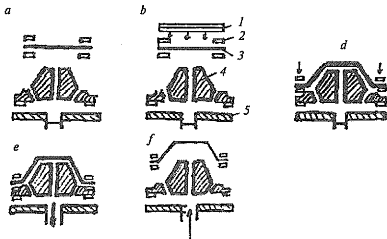
17-rasm. Termoplast listlardan buyum shakllash operatsiyalari:
