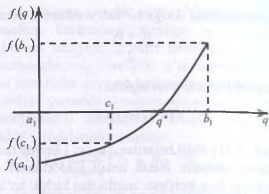
5.8-rasm. Oraliqni teng ikkiga bo'lish usulining grafik tasviri.
