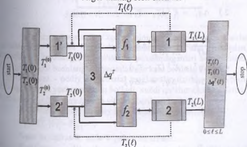
Algoritmnng blok-sxemasi
