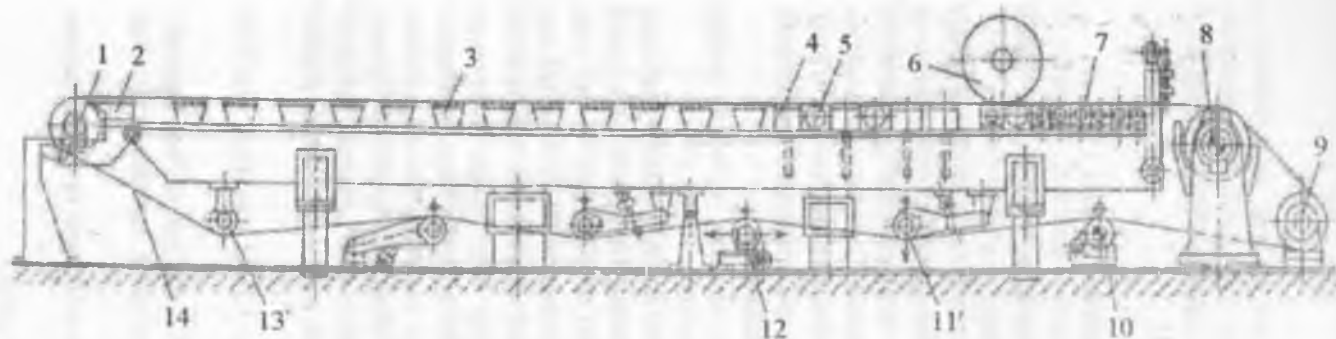
8.1-rasm. «Ho'l» vakuum va so'ruvchi qutilar bilan jihozlangan to'rli stol:
