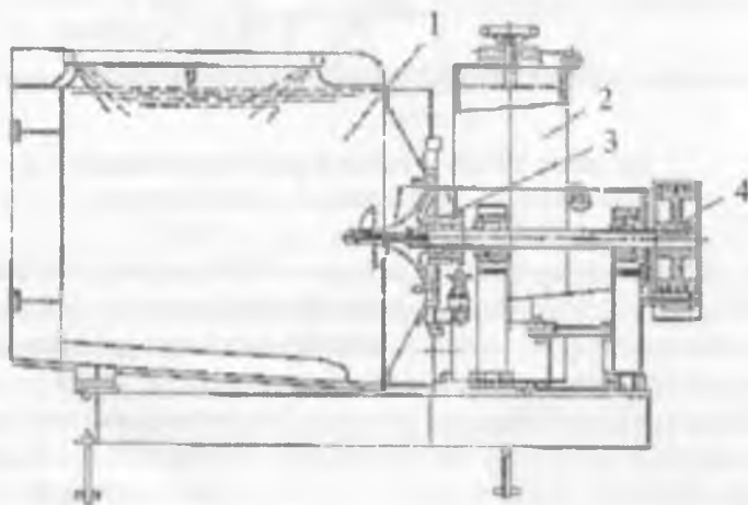
2.7-rasm. ГРГ-02-1 rusumli gorizontal gidromaydalagich:
