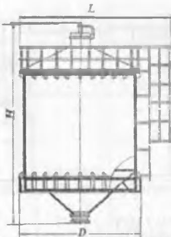
3.3-rasm. Suyultirilgan kimyoviy eritmalar saqlaydigan bak.
