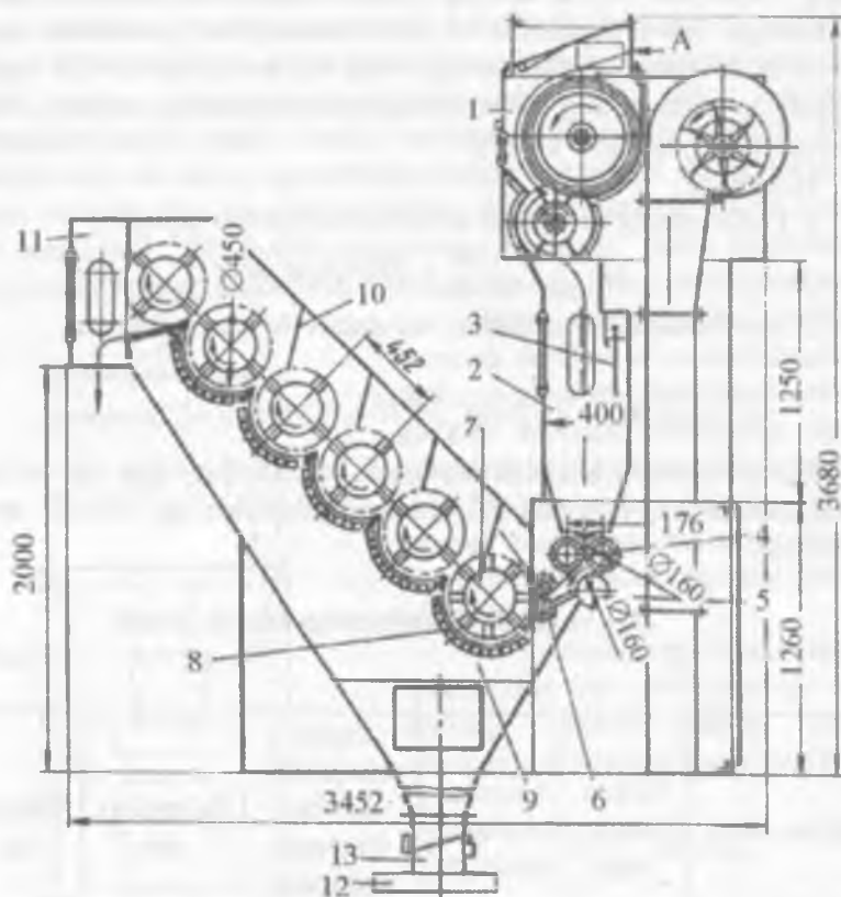
1.4-rasm. OH-6-4M rusumli tozalagichning bo'ylama kesimi.
