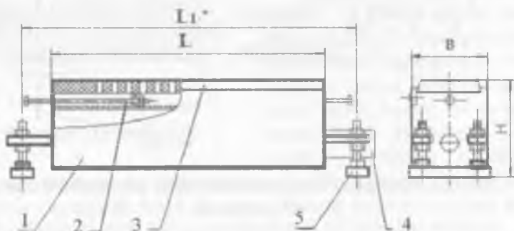
8.3-rasm. Namlikni so'ruvchi quti:
