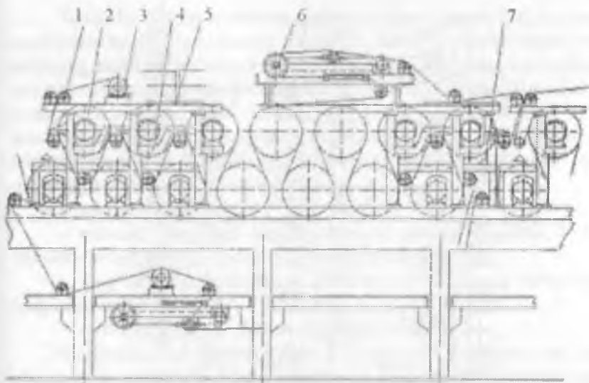
8.7-rasm. Ikki yarusda joylashgan quritish silindrlari:
