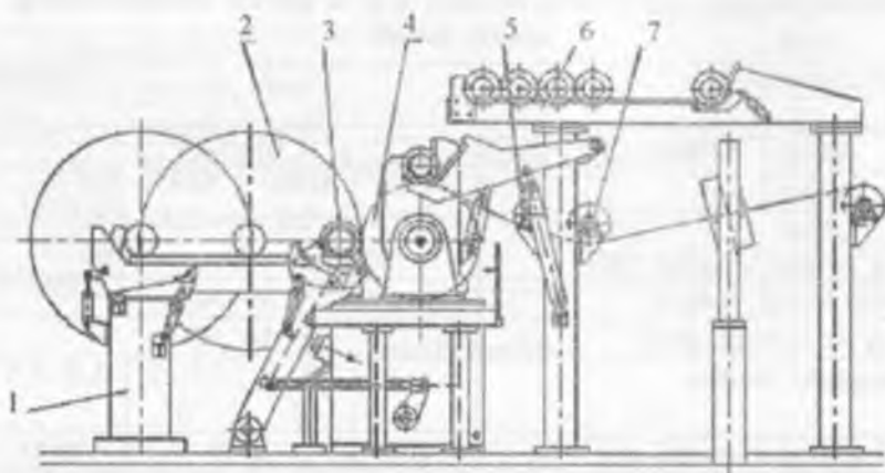
9.2-rasm. Magazinli tambur vali bor nakat (qog'oz o'rash): 1 – stanina; 2 – qog'oz o'ralgan val; 3 – yordamchi val; 4 – silindr; 5 – rulon qog'ozni to'g'rilovchi val; 6 – vallar magazini; 7 – qog'oz yetaklovchi val.
