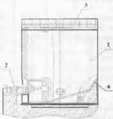
3.7-rasm. Gorizontaal aralashtirgichli havza (b): 1 – korpus; 2 – aralashtiruvchi qurilma; 3 – qopqog; 4 – silindr tubi.
