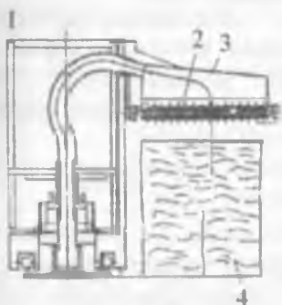
1.1-rasm. AP-18 rusumli mashinaning texnologik sxemasi:
