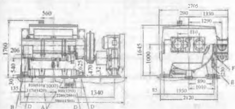
5.4-rasm. C2Б-07-35 va C2Б-10 rusumli ikki barabanli quyultirgichlarning gabarit chizmasi (qavs ichida-S2Б-10 o'lchamlari).
