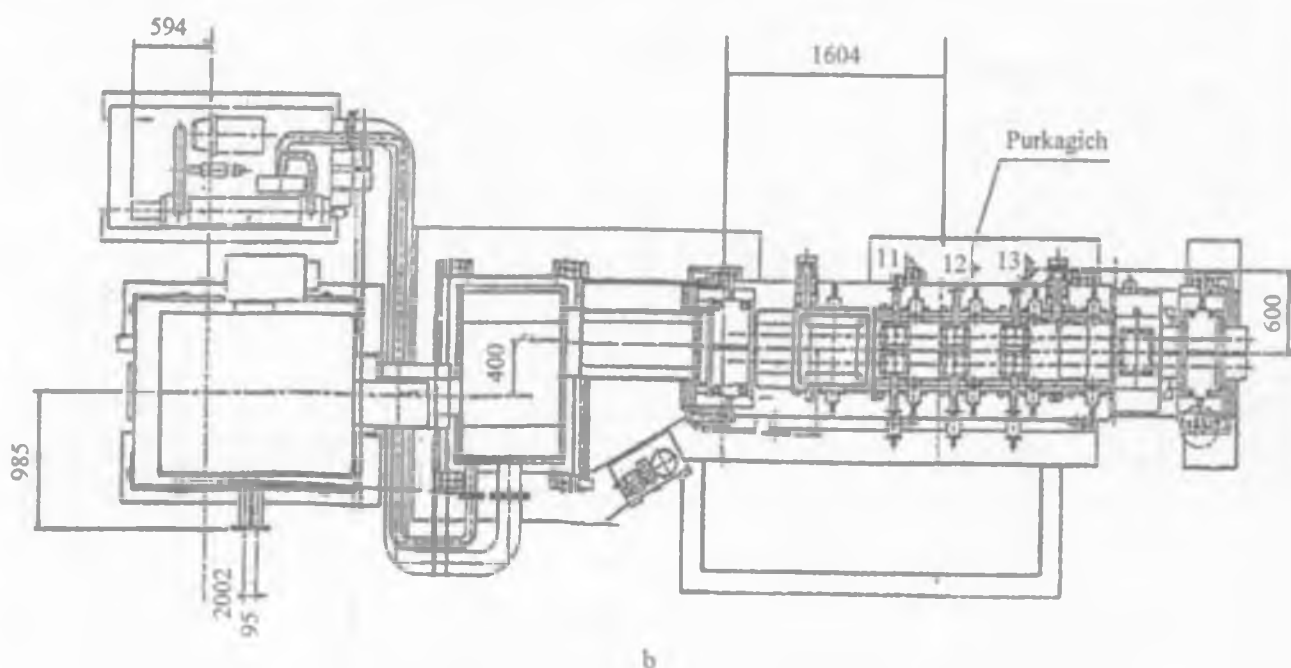
2.1-rasm. Bi-ViS mashinasining asosiy ko'rinishi va uning o'lchamlari: a – yonidan ko'rinishi; b – tepasidan ko'rinishi.
