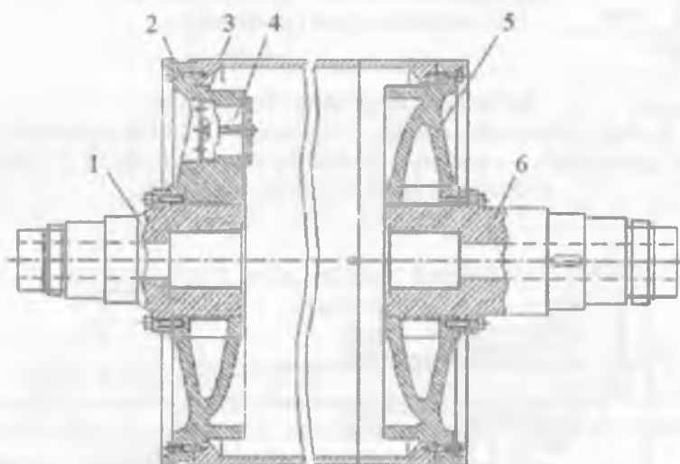
8.18-rasm. Qopqog'i alohida tayyorlangan quritish silindri: 1 – sapfaning yuza tomoni; 2 – qopqog'ning yuza tomoni; 3 – korpus; 4 – tuynuk; 5 – qopqog uzatmasi; 6 – uzatma tomonidagi sapfa.
