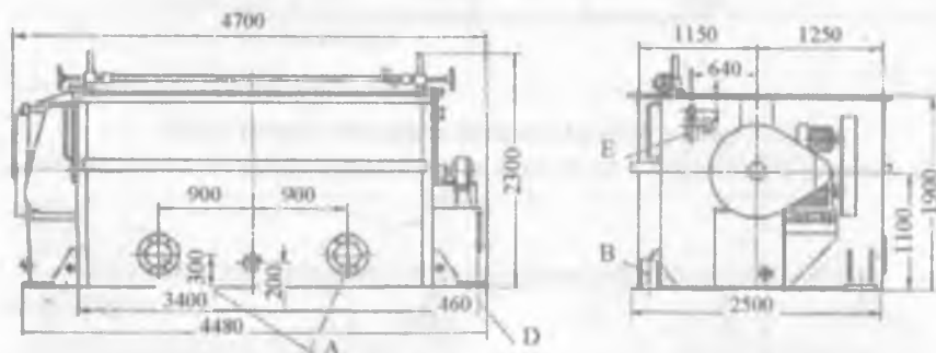
5.7-rasm. CQB-04 quyultirgichning chizmasi va gabarit o'lchamlari.
