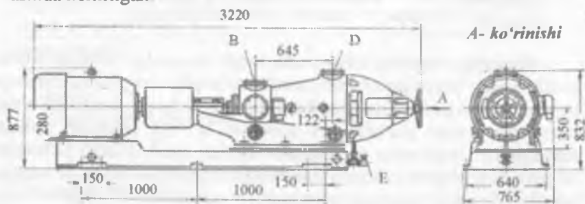
2.16-rasm. MKI-01M rusumli konussimon tegirmon va uning gabarit o'lchamlari.
