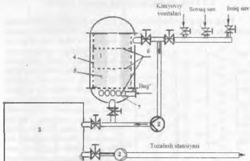
1.7-rasm. Paxta momig'ini pishirish qurilmasi sxemasi:
