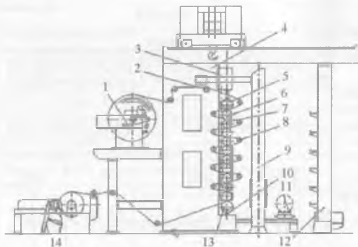
10.7-rasm. Superkalandr sxemasi:
