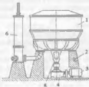
2.5-rasm. ГРБ-04 va ГРБ-05 rusumli gidromaydalagichlar:
