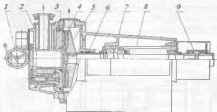
2.11-rasm. MD-14-1 rusumli diskli tegirmonning kesimli chizmasi:
