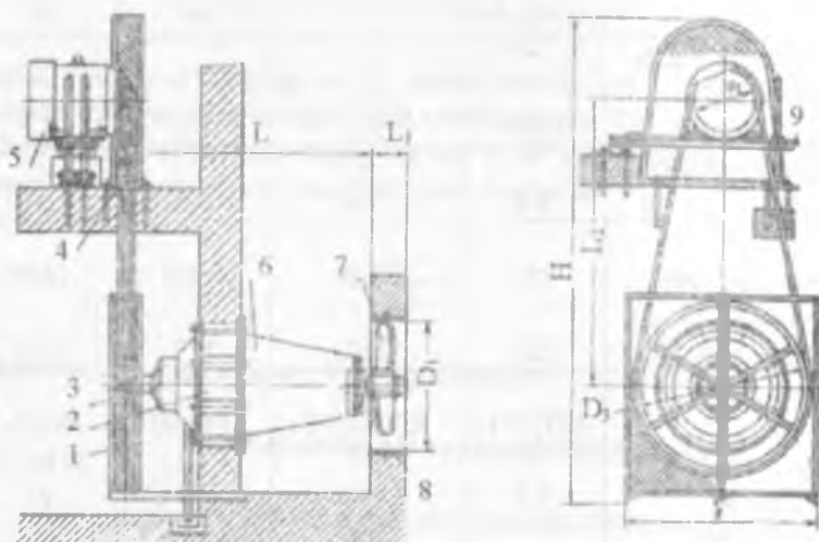
3.10-rasm. ЦУ-750-13, ЦУ-909-17, ЦУ-1500-40, ЦУ-1800-75 rusumli sirkulatsiyalovchi qurilma:
