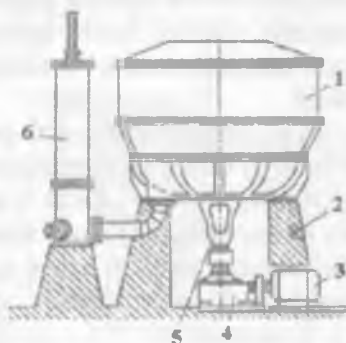
2.5-rasm. ГРБ-04 va ГРБ-05 rusumli gidromaydalagichlar: 1 – vanna; 2 – tayanch; 3 – dvigatel; 4 – reduktor; 5 – rotor; 6 – quti.
