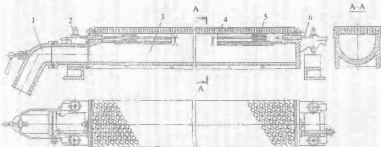
8.2-rasm. Namlikni so'ruvchi quti:
