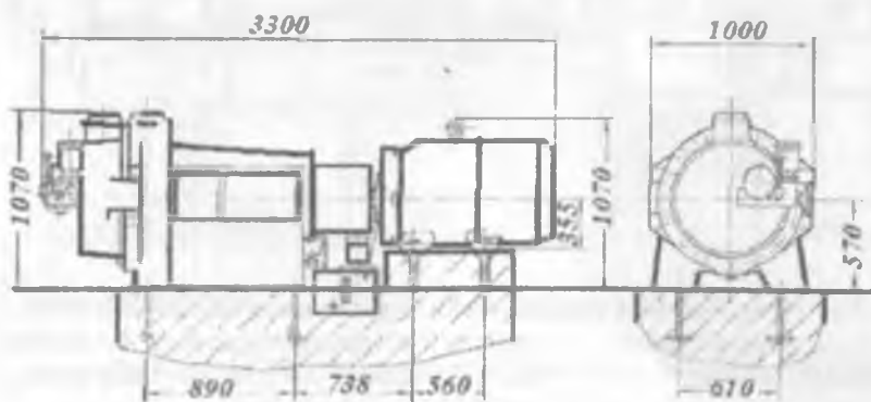
2.12-rasm. MД-14-1 rusumli diskli tegirmonning umumiy ko'rinishi va o'lchamlari chizmasi.
