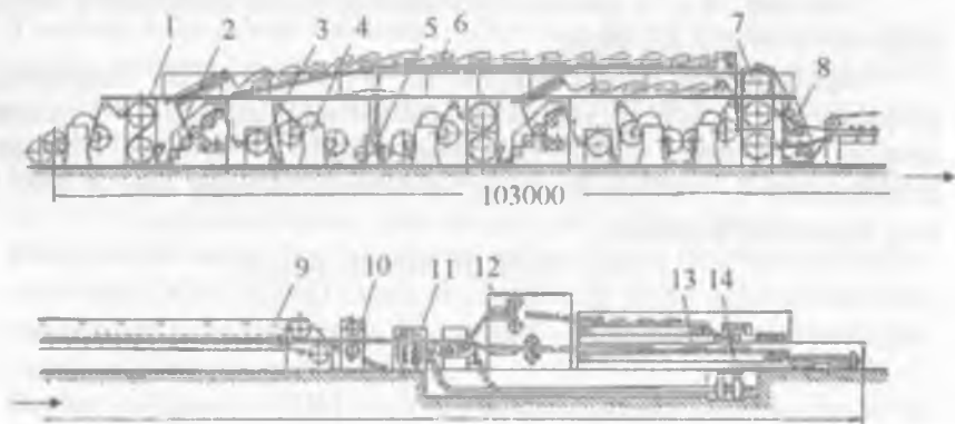
11.1-rasm. АГП2с-3Б rusumli gofrlash agregatining sxemasi:
