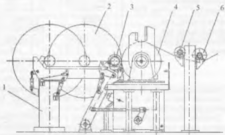
9.3-rasm. Magazinsiz tambur vali bor nakat (qog'oz o'rash): 1 – stanina; 2 – tamburli val (rulon qog'oz bilan); 3 – yordamchi val; 4 – silindr; 5 – rulon qog'ozni to'g'rilash val; 6 – qog'ozni yetaklovchi val.
