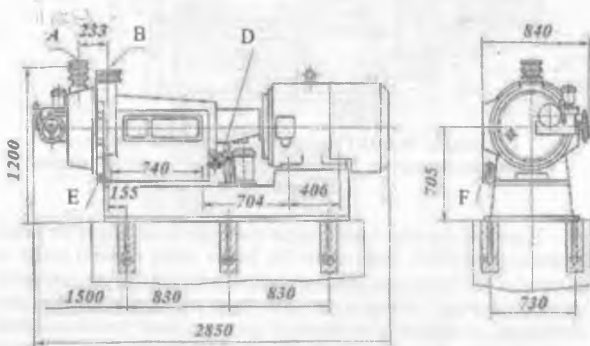
2.10-rasm. МД-02-1 rusumli diskli tegirmonning umumiy koʻrinishi va gabarit oʻlchashlari.
