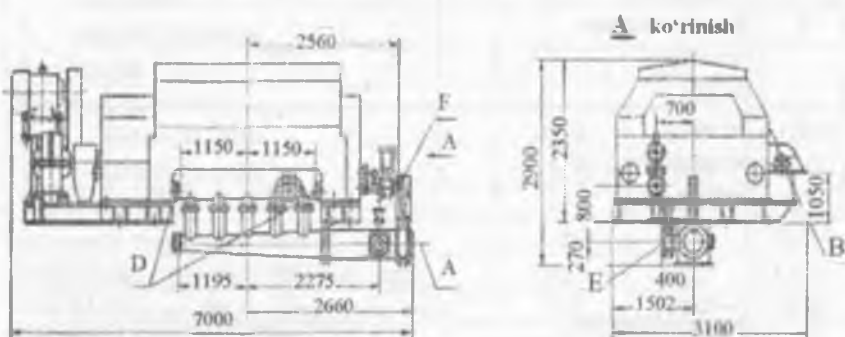
5.5-rasm. C2B-16 ikki barabanli quyultirgichning gaharit chizmasi.
