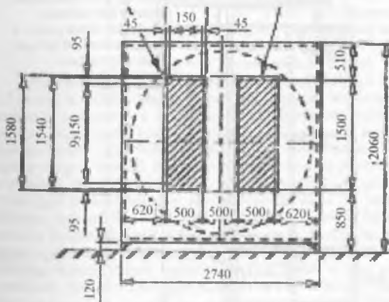
1.5-rasm. Chang-havo filtrining B kesimi ko'rinishi.
