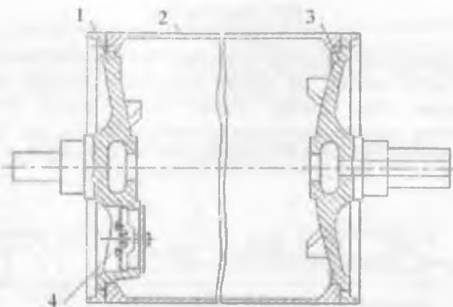
8.17-rasm. Qopqog'i quyib ishlangan quritish silindri. 1 – old tomonidagi qopqog; 2 – korpus; 3 – uzatma (orqa) tomonidagi qopqog; 4 – tuynuk
