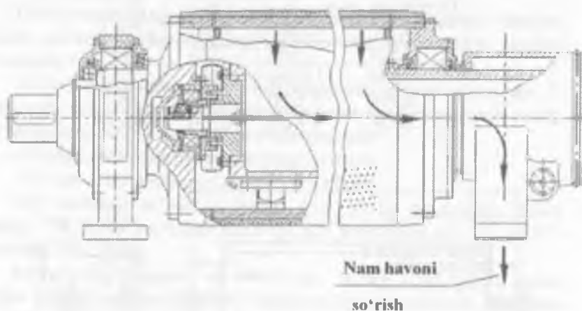
8.4-rasm. Old qismi ichiga joylashtirilgan podshipnikli nam so‘ruvchi val.
