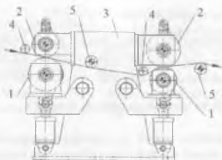
10.6-rasm. 2-tur «yumshoq» kalandr: 1 – kalandrli val; 2 – qizdiriladigan val; 3 – stanina; 4 – rulonni to'g'rilovchi val; 5 – qog'ozni yetaklovchi val.
