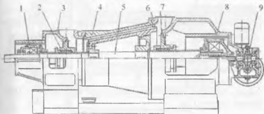
2.17. MK.I-03M rusumli konusli tegirmon:
