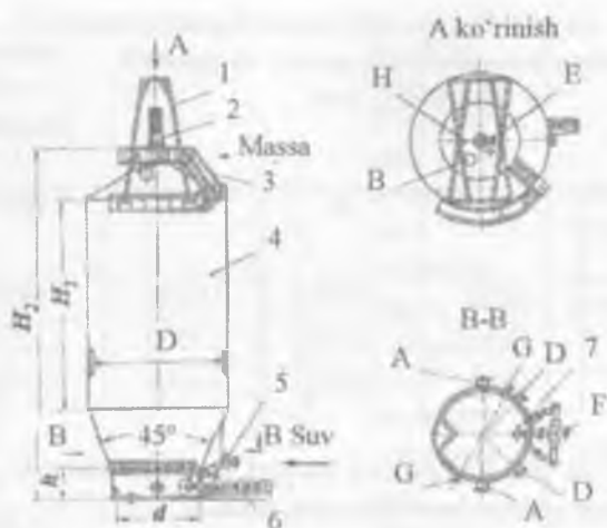
3.5-rasm. 204-49A, 204-51 va 204-62 rusumli yuqori konsentratsiyali massa uchun havzalar: 1 – rama; 2 – massani yuklash; 3 – ish may don-chasi; 4 – korpus; 5 – suyultirish qurilmasi; 6 – ha-rakatlantirgich; 7 – aralashtiruvchi qurilma.
