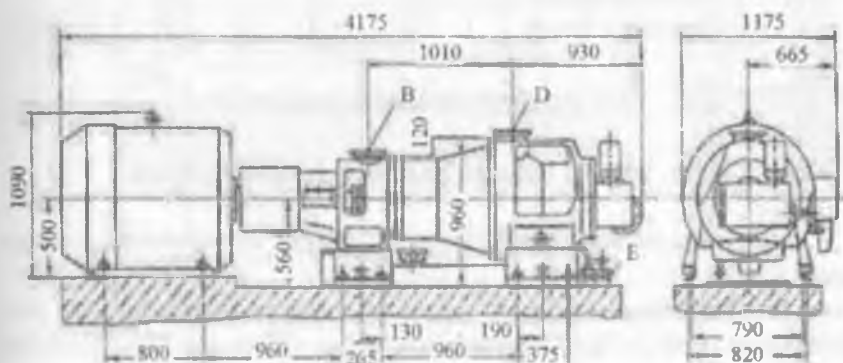
2.18-rasm. MK.I-03M rusumli konussimon tegirmon gabarit o'lchamlari.
