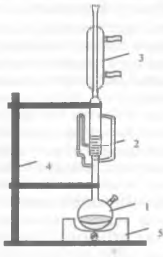
1-rasm. Ekstraksiya qurilmasi:
