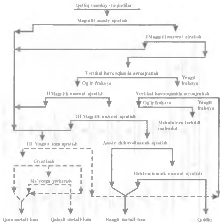
21.8-rasm. «Polimer» MIB da metallar va yengil fraksiyani ajratuvchi qattiq maishiy chiqindilarni boyitish prinsiplal texnologik sxemasi.
