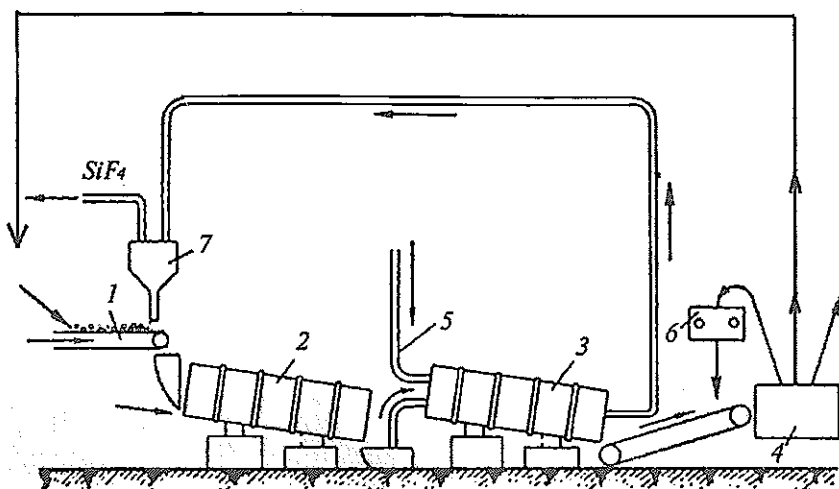
76- rasm. Superfosfatni donadorlash qurilmasining sxemasi.
