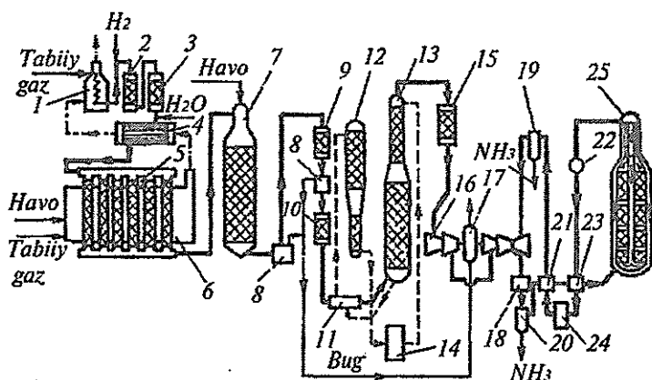
64- rasm. Ammiak ishlab chiqarish sxemasi.
