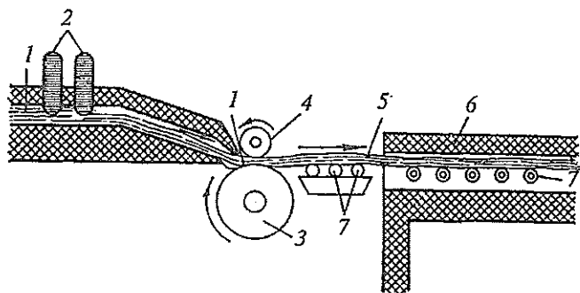
82- rasm. Uzlüksiz prokatlash orqali sayqallangan shisha listini tayyorlash sxemasi.
