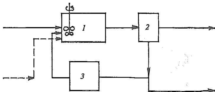
17- rasm. Oqova suvlarni biologik tozalash qurilmasining sxemasi. 1 — aerotenk; 2 — ikkilamchi tindirgich; 3 — balchiq regeneratori.
