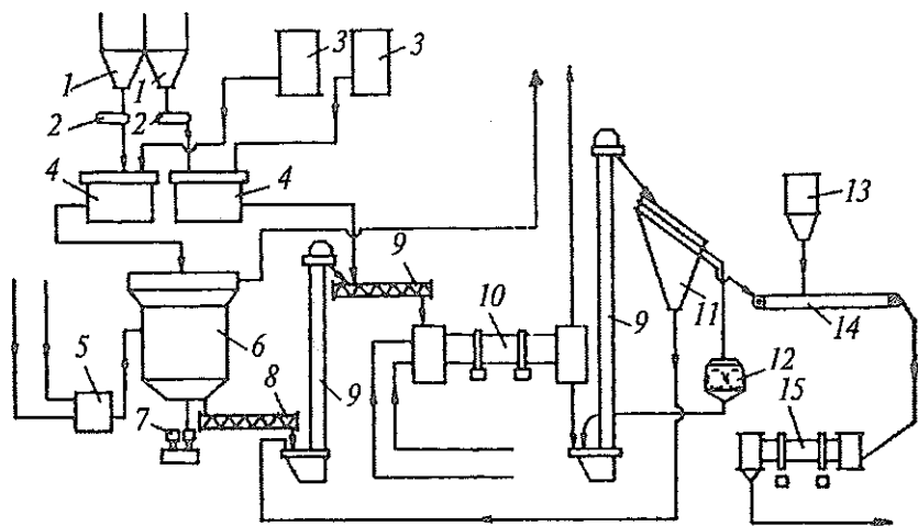
78- rasm. Fosforit uni va ekstraksion fosfat kislotasidan donador qo'sh superfosfatni uzluksiz ishlab chiqarish sxemasi.
