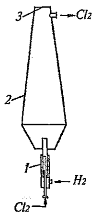
43- rasm. Vodorod xloridni sintezlash pechi. 1 — gorelka; 2 — pech korpusi; 3 — asbestli qopqoq.
