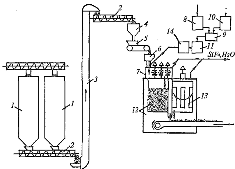
74- rasm. Uzlüksiz usulda superfosfat ishlab chiqarish sxemasi.
