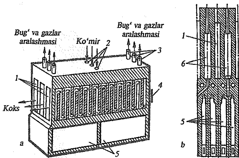
90- rasm. Koks batareyasi.
