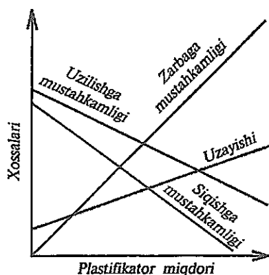
120- rasmi. Tarkibidagi plastifikator miqdoriga qarab polimer mexanik xossalari o'zgarishi.
