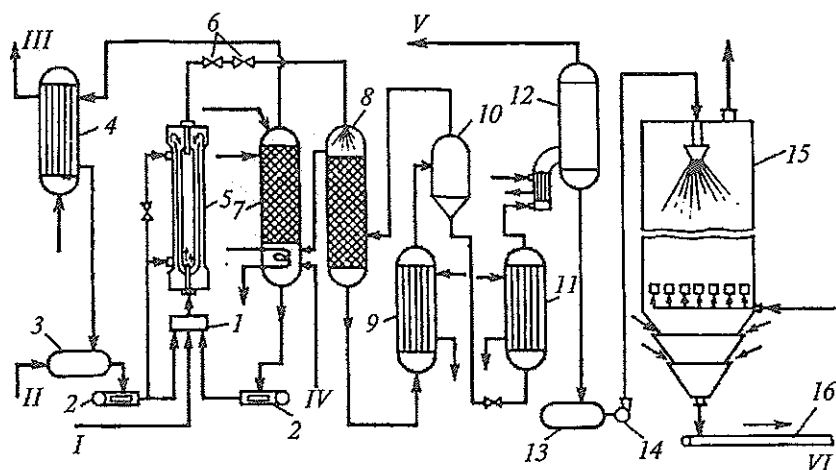
72- rasmi. Karbamid ishlab chiqarishning sxemasi.
