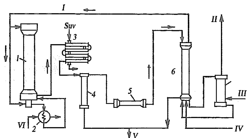
62- rasm. O'rta bosimda ammiak ishlab chiqarish sxemasi.
