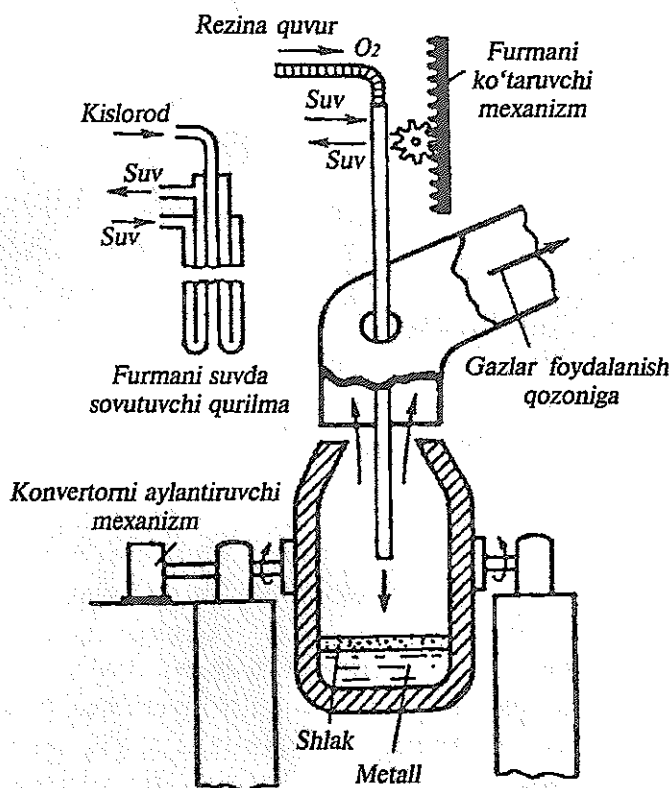
87- rasm. Po'lat eritish uchun kislorod konvertori.
