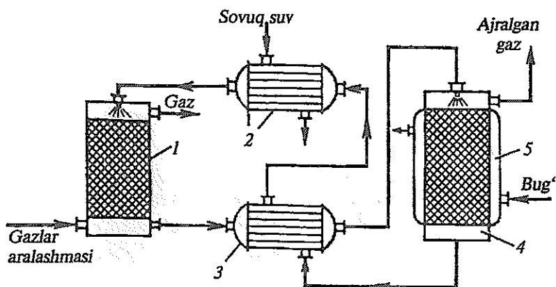
9- rasm. Adsorbsiya — desorbsiya usulida gazlarni ajratish qurilmasining sxemasi.
