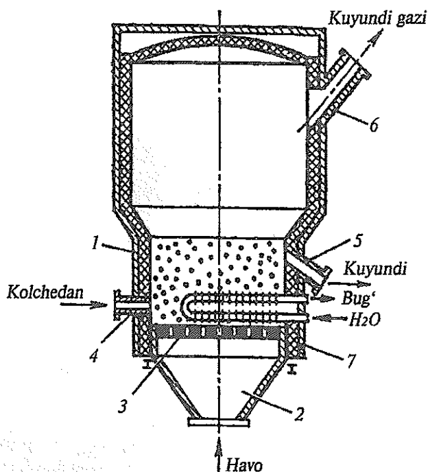
49- rasm Qaynovchi qavatda kuydirish pechi (kolchedan kuydirish pechi).
