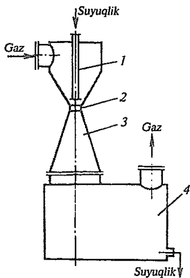
45- rasm. Venturi apparati.
