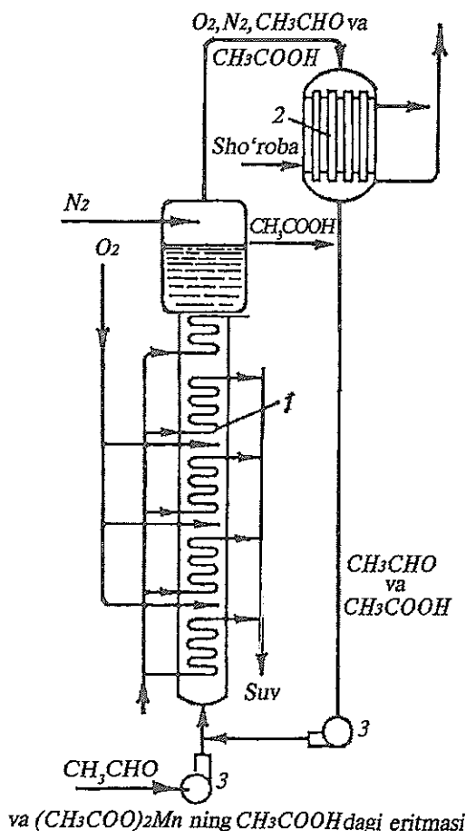
109- rasm. Sirka aldegidni oksidlab sirka kislotasi olish sxemasi. 1 — oksidlash minorasi(kolonnasi) 2 — kondensator; 3 — nasoslar.
