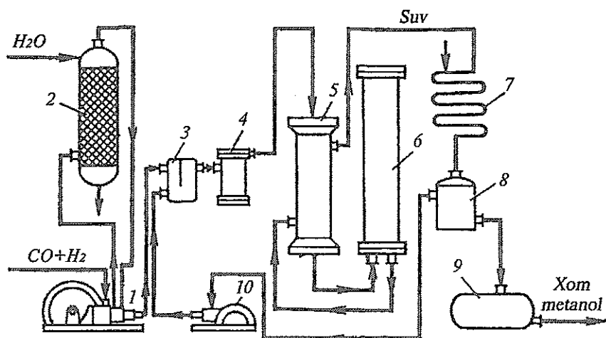
103- rasm. Uglarod (II) oksidi va vodoroddan metanol sintezi qurilmasining sxemasi.
