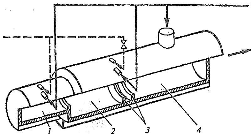
57- rasm. Oltingugurtni yoqish uchun ishlatiladigan siklon pechi. 1 — oltingugurtni berish uchun va havoni tangensial kiritish uchun forsunkali forkamera; 2,4 — yoqish bo'limi; 3 — gazni girdobli harakatga keltiruvchi halqalar.
