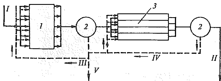
18- rasm. Aerotenklarda oqova suvlarning ikki bosqichli tozalash sxemasi. 1 — aerotenk — aralashtirgich; 2 — tindirgich; 3 — aerotenk reaktorlar; I — oqava suvlari tozalashga; II — oqava suvining tozalangani; III — birinchi bosqich aktiv balchig'i; IV — ikkinchi bosqich aktiv balchig'i; V — ortiqcha aktiv balchiq.
