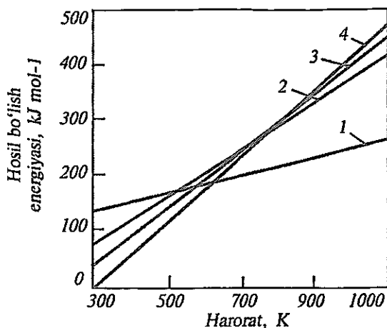
96- rasm. Uglevodorodlarning oddiy moddalaridan hosil bo'lish energiyasining haroratga bog'liqligi.
