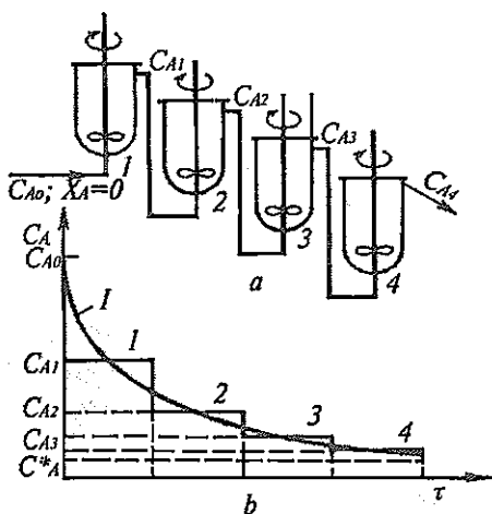
35 a, b- rasm. Ketma-ket ulangan to'liq aralashtirish reaktorlari. a — ketma-ket ulanish sxemasi; b — dastlabki asosiy modda konsentratsiyasining o'zgarishi; A — ketma-ketlik pog'onasi (1—4 pog'ona).
