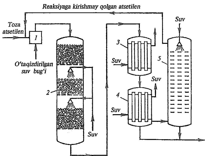
108- rasm. Atsetilenni bug' fazali gidratlash yo'li bilan sirka aldegid olish sxemasi.
