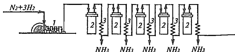
41 - rasm. Ochik zanjirli(batareyali) apparatlarda to'g'ri oqimli sistemada ammiak sintezi. 1 — yuqori bosimli kompressor; 2 — katalizatorli ammiak sintez ustuni(kolonnasi); 3 — ammiak kondensatori, sovutgichi.
