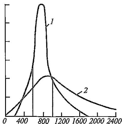
110- rasm. Polimerlarda molekularning molekular massalari bo'yicha taqsimlanishi. 1 — nitrosellyuloza; 2 — polistirol.
