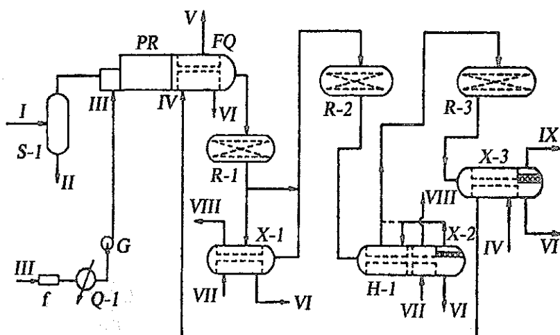
54- rasm. Muborak gazni qayta ishlash zavodining (GQIZ) oltingugurt ishlab chiqarish qurilmasining sxemasi.
