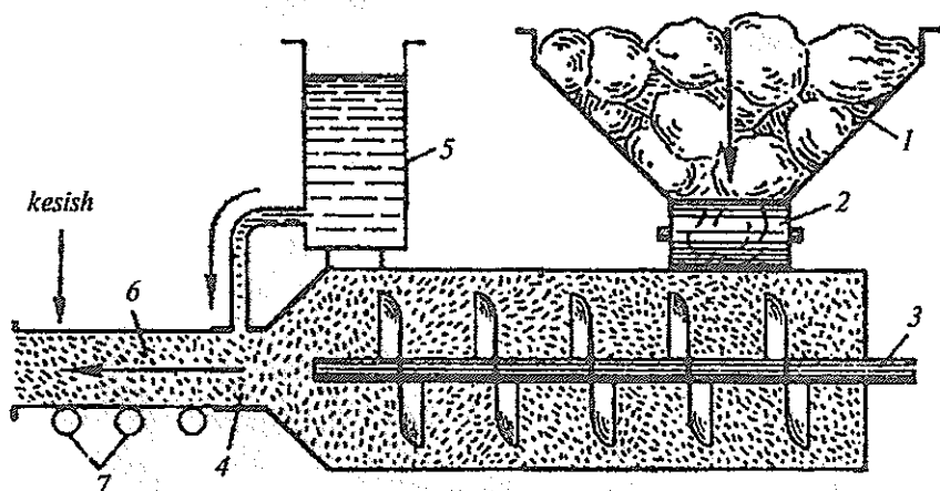
79- rasm. Lentali press apparati.
