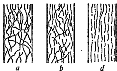
115- rasm. Tolaga shakl berishda chiziqli molekulalarning oriyentatsiyalanishi.
