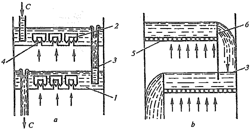
37- rasm. Barbatajli apparat tokchalarining(tarelka) sxemasi. a — gazni qalpoqchalar orqali taqsimlovchi apparat; b — panjarali(to‘rsimon tarelkali) apparat; 1 — qalpoqchali tarelka; 2 — qalpoqcha; 3 — suyuqlik oshib tushuvchi quvurcha; 4 — gaz o‘tuvchi quvurcha; 5 — to‘rsimon tarelka; 6 — quyuvchi ostonasi.
