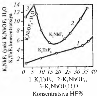
2- grafik. Turli konsentratsiyali plavik kislotalarda tantal va niobiyning fiortli komplekslarining (25°C da) erishi.
