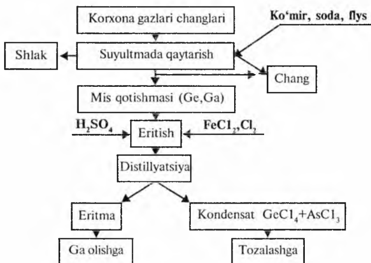
9- chizma. Korxona gazlari va changidan germaniyni olish texnologik sxemasi.
