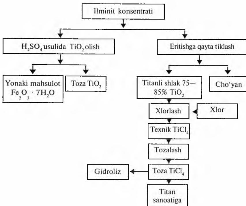
5-chizma. Ilminiti konsentratidan TiCl 4 yoki TiO 2 ni olish.
