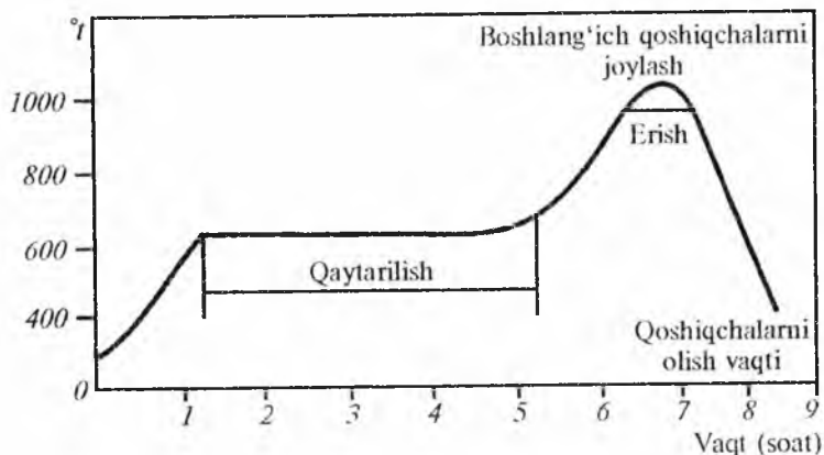
3- grafik. \text{GeO}_2 ni qaytarish sharoiti va undagi germaniyli qoshiqchaning o'choqda harakatlanishi.
