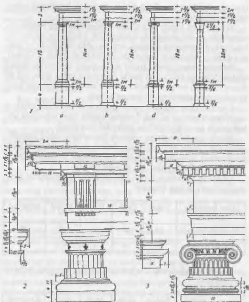
15-rasm. Rim orderlari (Vinola bo'yicha):
