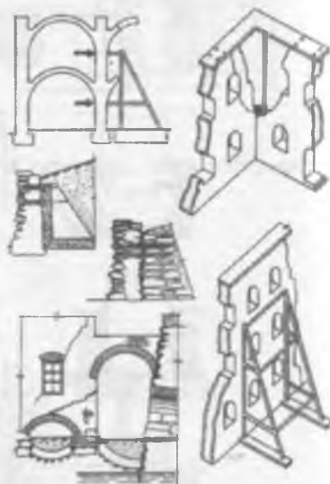
3.7.11-rasm. Nuragan konstruksiyalarni mustahkamlash.
