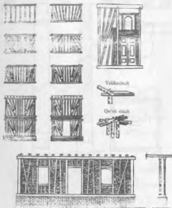
1-rasm. Sinchli devorlar.
