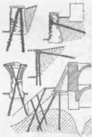
3.7.8-rasm. Burg'ulab inyeksiyalangan qoziqlar.
