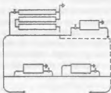
4.4.1-rasm. Pastdan issiqlik uzatuvchi gorizontali ko'rinishli isitish tarmog'i: a-ikki quvurli; b-bir quvurli.
