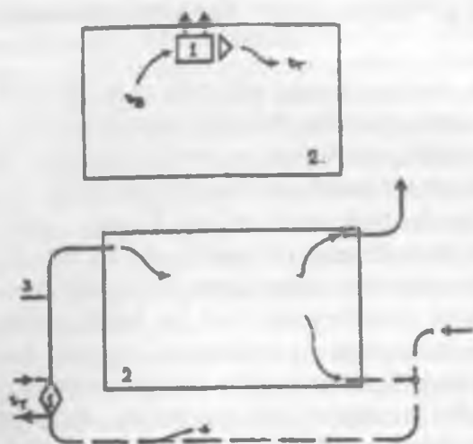
4.4.3-rasm. Havo bilan isitish tarmog'ining shartli sxemasi: a-mahalliy tarmoq; b-markazlashgan tarmoq; 1-kalorifer; 2-xona; 3-va 4-tarqatuvchi va qaytaruvchi havo tarmoqlari.
