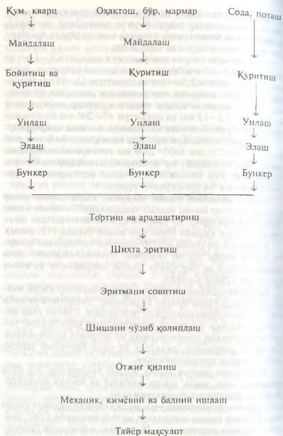
12- расм. Дераза ойнаси ишлаб чиқаришнинг соддалаштирилган схемаси.
