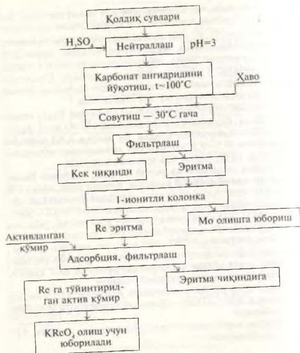
43-расм. Ренийни эритмалардан сорбциялаб ажратиш олишнинг технологик схемаси.
