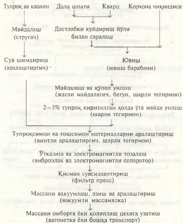
4- расм. Пластик чинни массасини сувли унлаш ва аралаштириш йули билан тайёрлаш схемаси.
