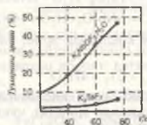
27-расм. Калий фтортанталат ва фтороксиниобат тузларининг 1% ли плавик кислотаси ва температура узгариши билан эриши.
