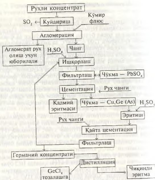
31-рasm. Германий олишнинг технологик схемаси.
