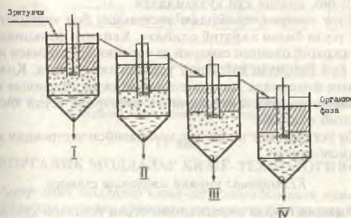
49-расм. Ярим тескари оқимда экстракциялаш. I, II, III, IV-сувли эритма фракциялари: I — аралаштириш камераси; 2 — тиндириш камераси.
