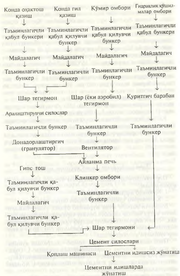
20- расм. Қуруқ усулда портландцемент ишлаб чиқариш технологияси схемаси.
