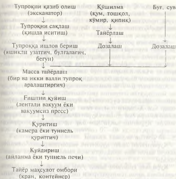
1- расм. Қурилиш гишти ишлаб чиқаришнинг технологик тизими.
