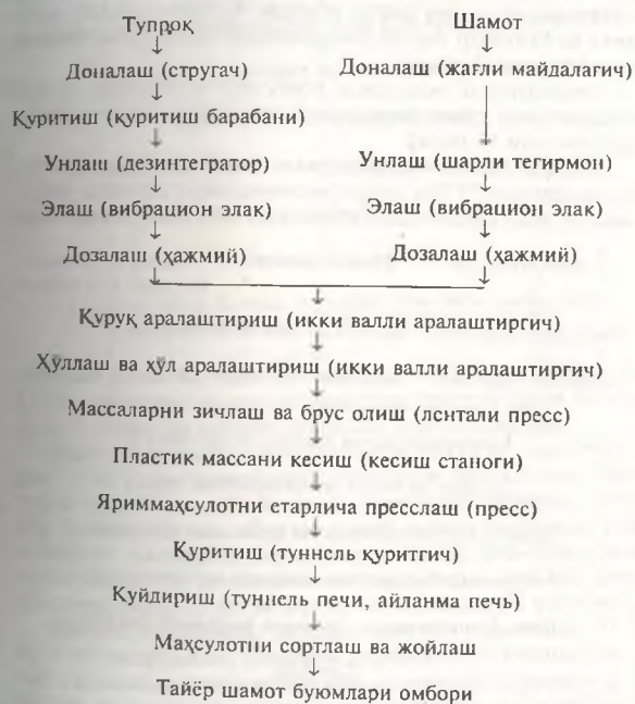
6-рису. Пластик пресслаш усулида шамот ғишти олишнинг технологик схемаси.
