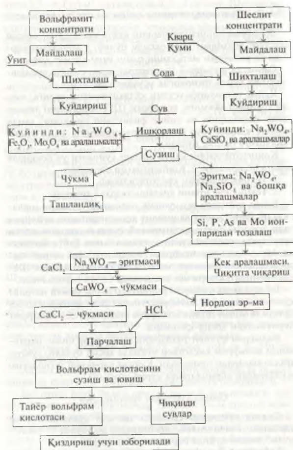
21-расм. Вольфрамит ёки шеелитнинг содали куйдириш технологияси.
