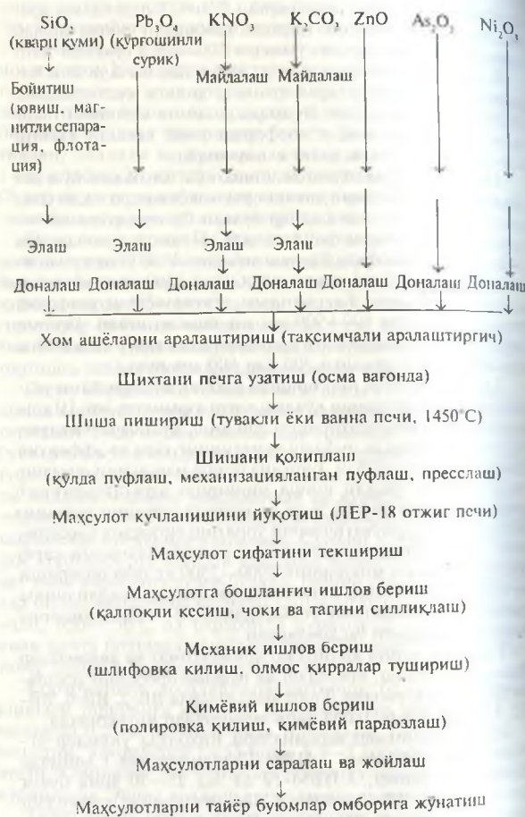
16-расм. Қурғошинли биллур маҳсулотлар ишлаб чиқаришнинг технологик схемаси.
