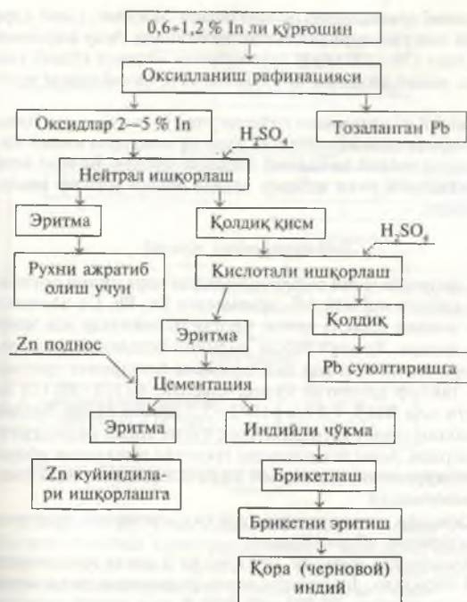
38-расм. Рух қорасини рафинациялашда ҳосил булган қўғошин таркибидаги индийни ажратиб олиш технологияси.
