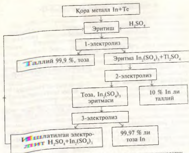
39-расм. Электрохимёвий усулда индий олишнинг технологик схемаси.
