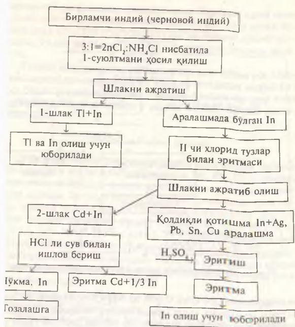
40-расм. Клемвий усулда индий олишнинг технологик схемаси.
