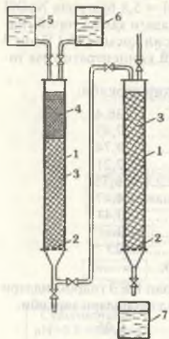
47-расм. Ион алмашиниш усулида элементларни ажратиш олиш асбобининг схемаси:
