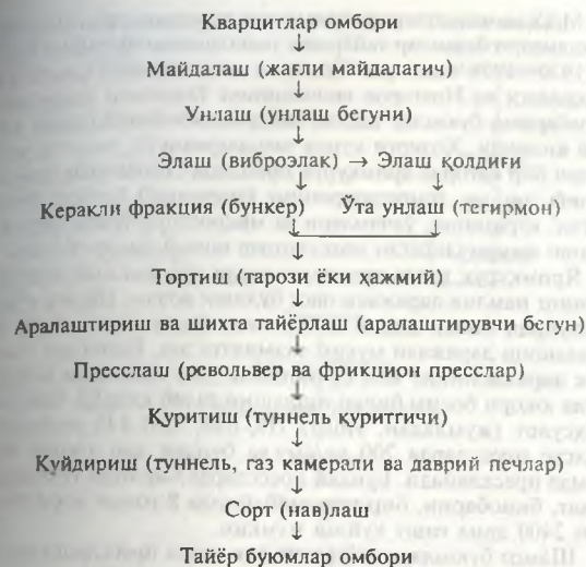
8-расм. 150 \text{ кг/см}^2 босимда пресслаш йўли билан динас ғишти ишлаб чиқаришнинг технологик схемаси.
