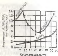
28-расм. Турли концентрацияда плавик кислоталарда тантал ва ниобийнинг фторли комплексларини (25°Cда) эриши.
