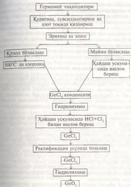
35-расм. Германий чиқиндиларининг қайта ишлаш технологик схемаси.
