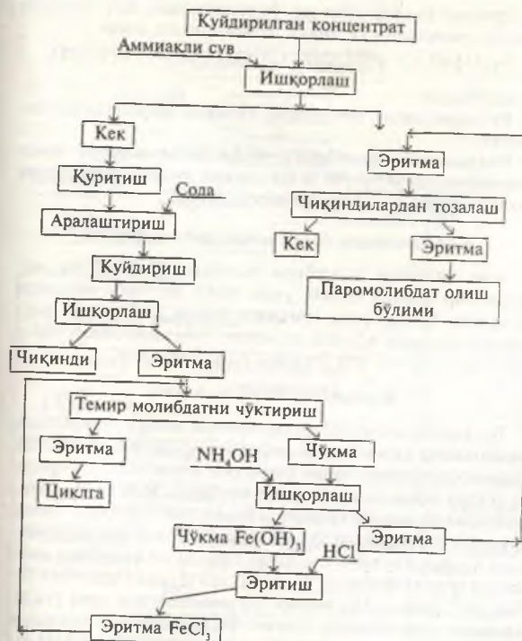
24- расм. Чиқиндилардан молибден олиш технологик схемаси.
