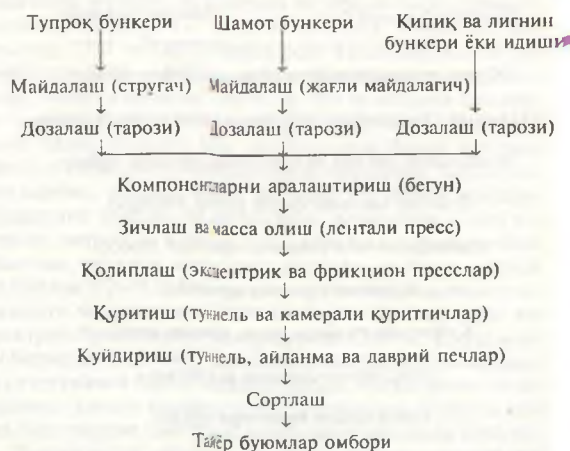
7-расм. Энгил вазли шамот ғишти тайёрлашнинг технологик тизими.
