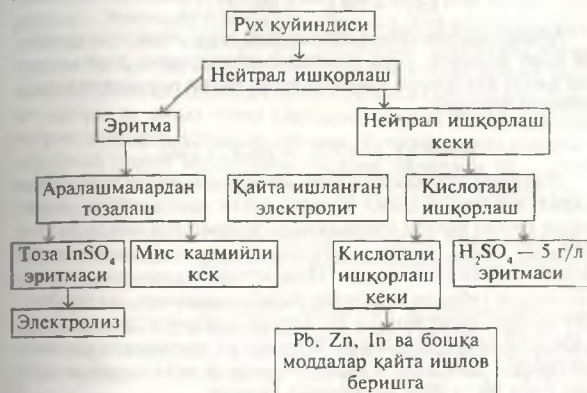
36-расм. Рух ишлаб чиқаришнинг гидрометаллургик схемаси.
