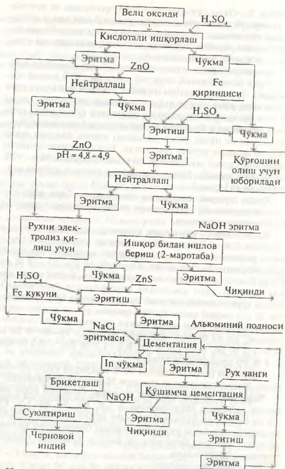
37-рasm. Вcльц оксидларидан индийни олиш технологик схемаси.
