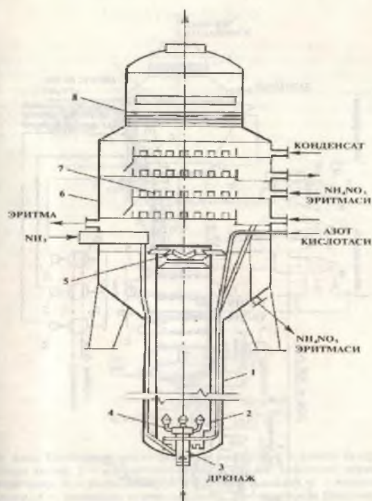
54- расм. ИТН ускунаси: 1 — реакция қисми қобиғи, 2 — реакция стакани, 3 — аммиак қўпиклагичи, 4 — нитрат кислотаси қўпиклагичи, 5 — гидроблагич, 6 — сепаратор қобиғи, 7 — қалпоқсимон ликобча, 8 — элаксимон томчи қайтаргич.
