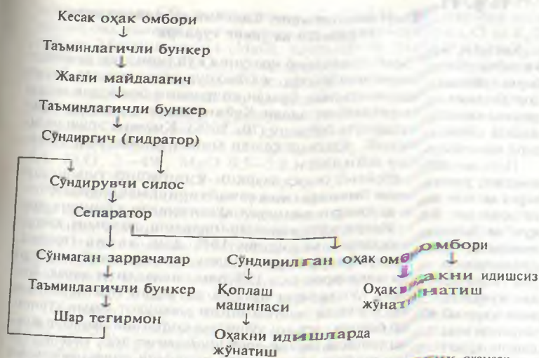
19-расм. Кукунсимон оҳак тайёрлашнинг технологик схемаси.
