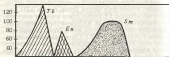
48-расм. Смолда ютилган тербий, европий ва самарий элементларини \text{pH} = 3,62 да 0,26 молярли ЭДТС эритмаси билан ажратиш (ювиб) олиш эгри чизиқлари.
