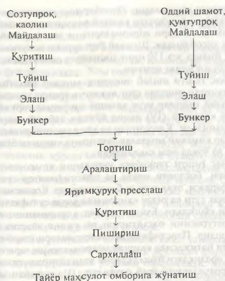
9-расм. Яримкуруқ усулда пресслаш орқали шамот буюмларни ишлаб чиқариш технологик схемаси.
