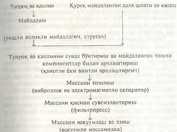
5- расм. Пластик массани қуқунланган тошсимон материаллардан фойдаланган ҳолда тайёрлаш схемаси.
