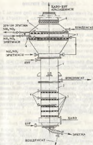
56- расм. Комбинацияланган буғлатиш ускунаси: 1 — қобиғи қувурсимон қисми, 2 — концентрациялаш қисми, 3 — элаксимон чўкма ликобчалар, 4 — иссиқлик берувчи илонсимон найлар, 5 — тозалаш қисми, 6 — элаксимон томчи қайтаргич, 7 — элаксимон ўтказувчи ликобчалар.
