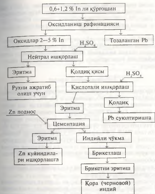
38-расм. Рух қорасини рафинациялашда ҳосил бўлган қўرғошин таркибидаги индийни ажратиб олиш технологияси.
