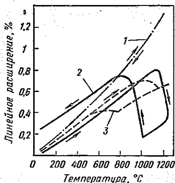
Рис. 34. Термическое расширение диоксида циркония
