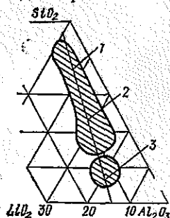
Рис. 46. Области составов системы \text{LiO}_2\text{—Al}_2\text{O}_3\text{—SiO}_2 с отрицательным термическим расширением 1 — петалит; 2 — сподумен; 3 — эвкрипит
