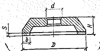
Рис. 28. Шлифовальный (алмазный чашечный) круг АЧК
