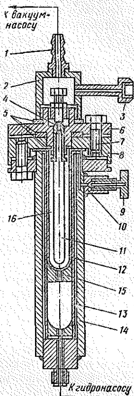
Рис. 15. Форма для гидростатического прессования чехлов к термopам 1 — штуцер для подвода вакуума; 2 — колпак; 3 — штуцер для подключения вакуумметра; 4 — втулка поглотителя; 5 — прокладка; 6 — крышка; 7 — болт; 8 — зажимное кольцо; 9 — вентиль; 10 — втулка; 11 — рол; 12 — рубашка; 13 — ограничитель; 14 — камера прессования; 15 — перемещаемый поддон; 16 — прессуемый порошок
