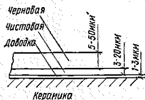
Рис. 27. Стадии механической обработки керамики
