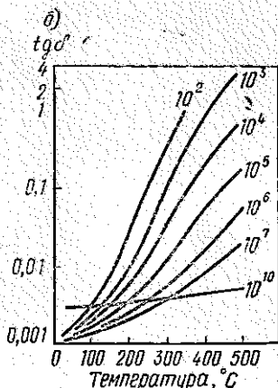
Рис. 11. Температурная зависимость \operatorname{tg} \delta керамики — титановой (а) и стеатита (б) — при различных частотах (цифры на кривых даны в Гц)
