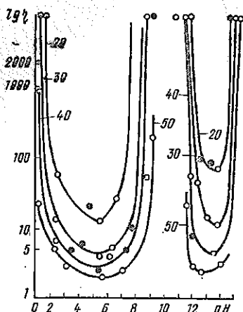
Рис. 29. Зависимость вязкости шликера из глинозема от его рН и влажности (цифры на кривых — влажность шликера, %)
