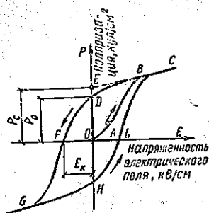
Рис. 49. Схематическое изображение сегнетоэлектрической петли гистерезиса
