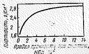
Рис. 38. Зависимость предела прочности BeO при сжатии от плотности
