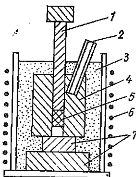
Рис. 20. Принципиальная схема установки для горячего прессования керамики
