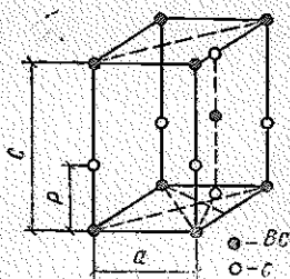
Рис. 37. Кристаллическая решетка \text{BeO} (типа вюрцита)
