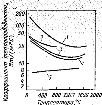
Рис. 4. Теплопроводность некоторых видов керамики
