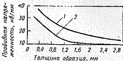
Рис. 13. Изменение пробивной напряженности при различной температуре
