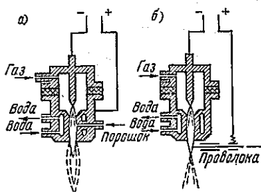
Рис. 64. Схемы плазменного напыления покрытий
