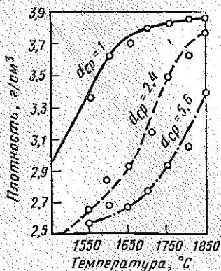
Рис. 30. Спекание корунда в зависимости от дисперсности исходного глинозема ( d_{ср} , мкм)
