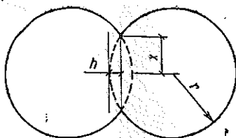
Рис. 23. Модель жидкостного спекания без взаимодействия между твердой и жидкой фазами
