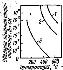
Рис. 42. Температурная зависимость удельного объемного сопротивления высокоглиноземистой керамики
