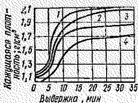
Рис. 61. Зависимость плотности BN от продолжительности горячего прессования при 1800 °С и различных давлениях, МПа
