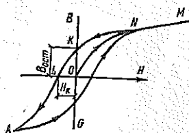
Рис. 57. Схематическое изображение петли магнитного гистерезиса
