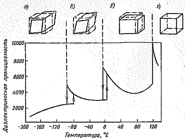
Рис. 51. Температурная зависимость диэлектрической проницаемости различных форм \text{BaTiO}_3 и области их стабильности
