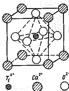
Рис. 50. Кристаллическая решетка типа перовскита
