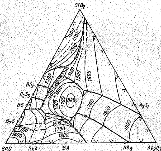
Рис. 45. Диаграмма состояния \text{BaO}-\text{Al}_2\text{O}_3-\text{SiO}_2
