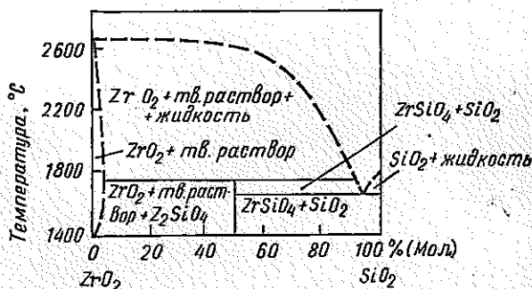
Рис. 44. Диаграмма состояния системы ZrO_2 — SiO_2
