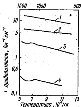
Рис. 59. Изменение проводимости твердого раствора хромита лантана состава \text{La}_{1-x}\text{Ca}_x\text{CrO}_{3-(x/2)} в зависимости от содержания Са
