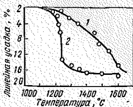
Рис. 31. Спекание корунда
