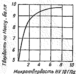
Рис. 26. Корреляция между микротвердостью и твердостью по Моосу
