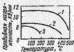
Рис. 13. Изменение пробивной напряженности при различной температуре
