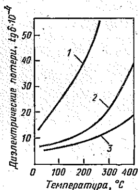
Рис. 43. Зависимость диэлектрических потерь \text{tg}\delta стеатитовой керамики из массы пластичной (1), малопластичной (2), непластичной (3) от температуры при частоте 1 МГц
