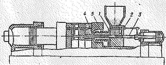
Рис. 16. Схема литейной машины для керамических масс
