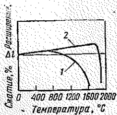
Рис. 2. Типичные кривые деформации под нагрузкой 1 — керамики со значительным содержанием стекловидной фазы; 2 — оксидной керамики кристаллического строения
