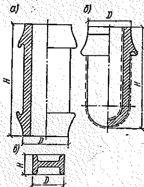
Рис. 48. Высоковольтные конденсаторы
