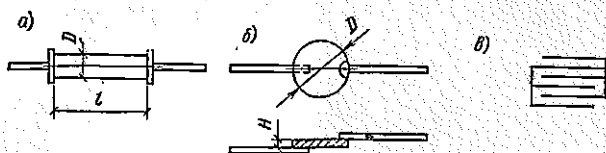
Рис. 47. Высокочастотные конденсаторы
