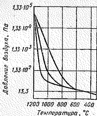
Рис. 58. Типовые программы давления воздуха в печи в зависимости от температуры при охлаждении изделий из Mn-Zn ферритов
