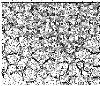
Рис. 39. Прозрачная керамика состава \text{Y}_2\text{O}_3 (90%) и \text{ZrO}_2 (10%). Преобладающий размер кристаллов 30—40 мкм
