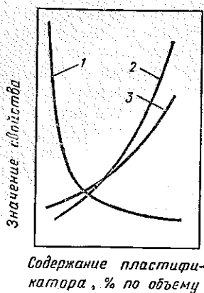
Рис. 17. Изменение свойств шликера — вязкости (1), литейной способности (2), расслаивания (3) — в зависимости от содержания пластификатора
