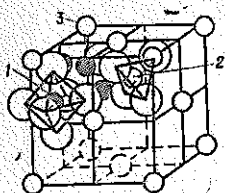
Рис. 54. Элементарная ячейка структуры шпинели
