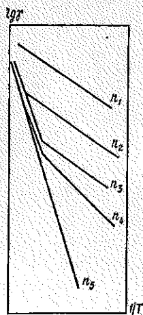
Рис. 9. Температурная зависимость собственной и примесной электропроводности керамики ( n — концентрация примесей, причем n_1 > n_2 > n_3 \dots )
