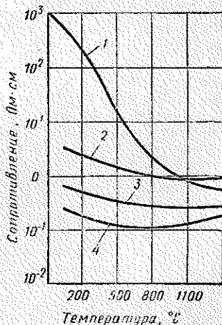
Рис. 60. Температурная зависимость сопротивления различных видов карбида кремния и нагревателей
