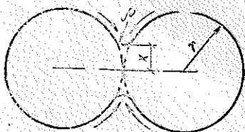
Рис. 25. Модель спекания по механизму «испарение — конденсация»
