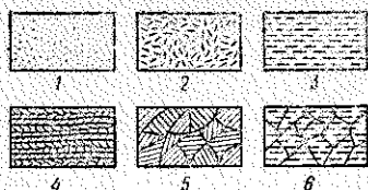
Рис. 62. Типичные структуры композиционных материалов (КМ)
