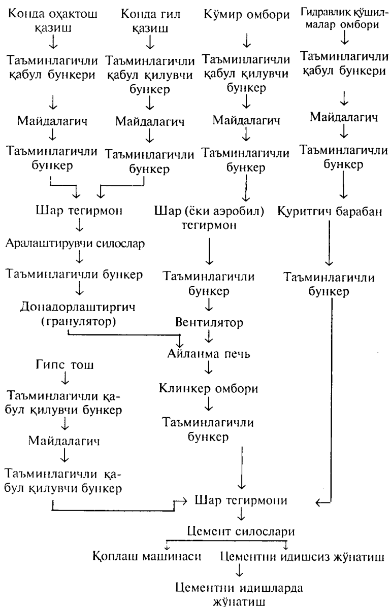
20- расм. Қуруқ усулда портландцемент ишлаб чиқариш технологияси схемаси.
