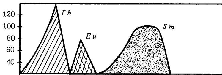
48-расм. Смолада ютилган тербий, европий ва самарий элементларини \text{pH} = 3,62 да 0,26 молярли ЭДТС эритмаси билан ажратиб (ювиб) олиш эгри чизиклари.
