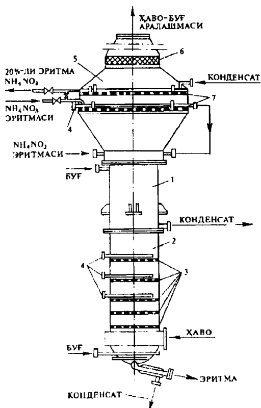
56- расм. Комбинацияланган буғлатиш ускунаси: 1 — қобиғи қувур-симон қисми, 2 — концентрациялаш қисми, 3 — элаксимон чўкма ликобчалар, 4 — иссиқлик берувчи илонсимон найлар, 5 — тозалаш қисми, 6 — элаксимон томчи қайтаргич, 7 — элаксимон ўтказувчи ликобчалар.
