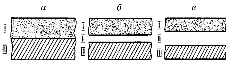
30- расм. Энергия зоналари: а — ўтказгичлар, б — яримўтказгичлар, в — изоляторлар. I — ўтказувчанлик зонаси, II — тақиқланган зона, III — валент (тўйинган) зона.
