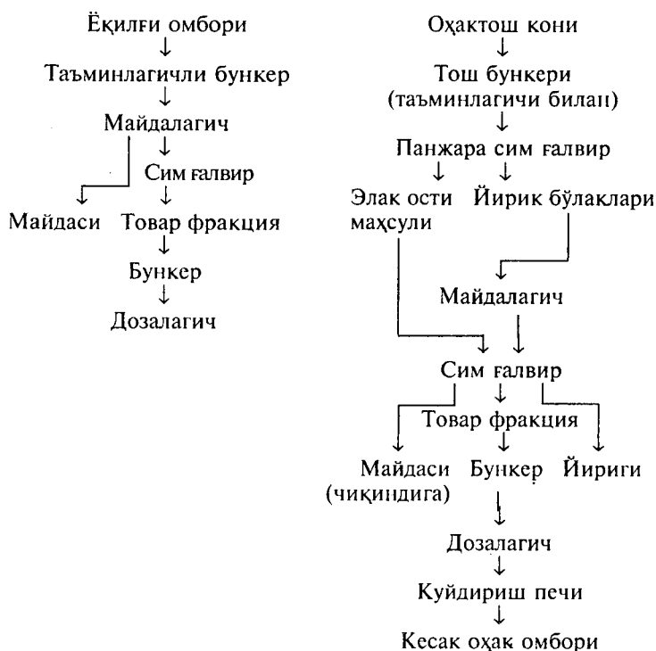
18-расм. Сўндирилмаган кесаксимон оҳак ишлаб чиқаришнинг технологик схемаси.
