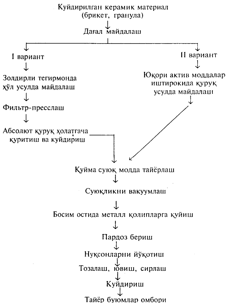
II- расм. Босим остида буюмларни қуйиш (технологик) жараёнининг принципиал тизими.
