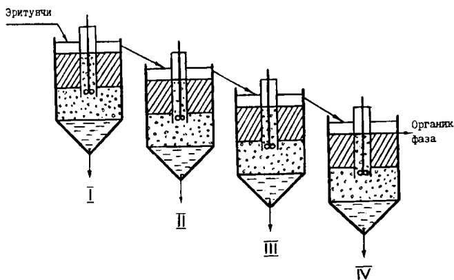
49-расм. Ярим тескари оқимда экстракциялаш. I, II, III, IV-сувли эритма фракциялари: I — аралаштириш камераси; 2 — тиндириш камераси.
