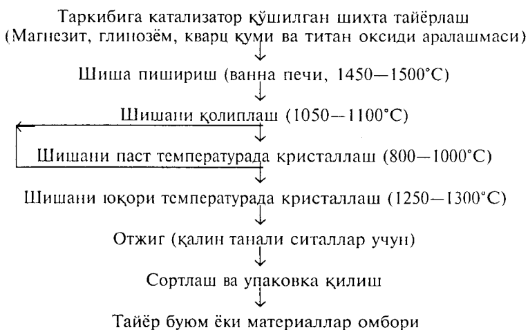
17- расм. Бир ва икки поғонали ситал буюмлар олишнинг содда схемаси.
