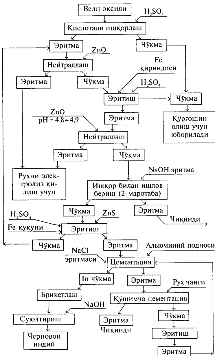
37-расм. Велц оксидларидан индийни олиш технологик схемаси.
