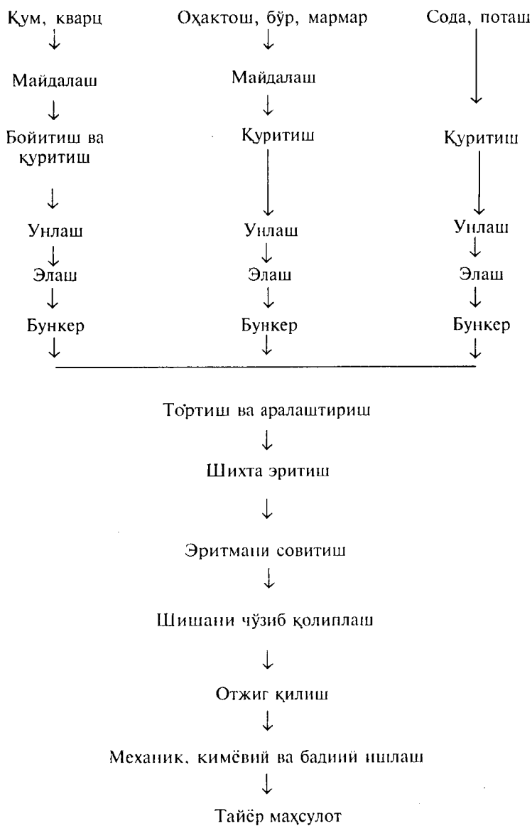
12- расм. Дераза ойнаси ишлаб чиқаришнинг соддалаштирилган схемаси.
