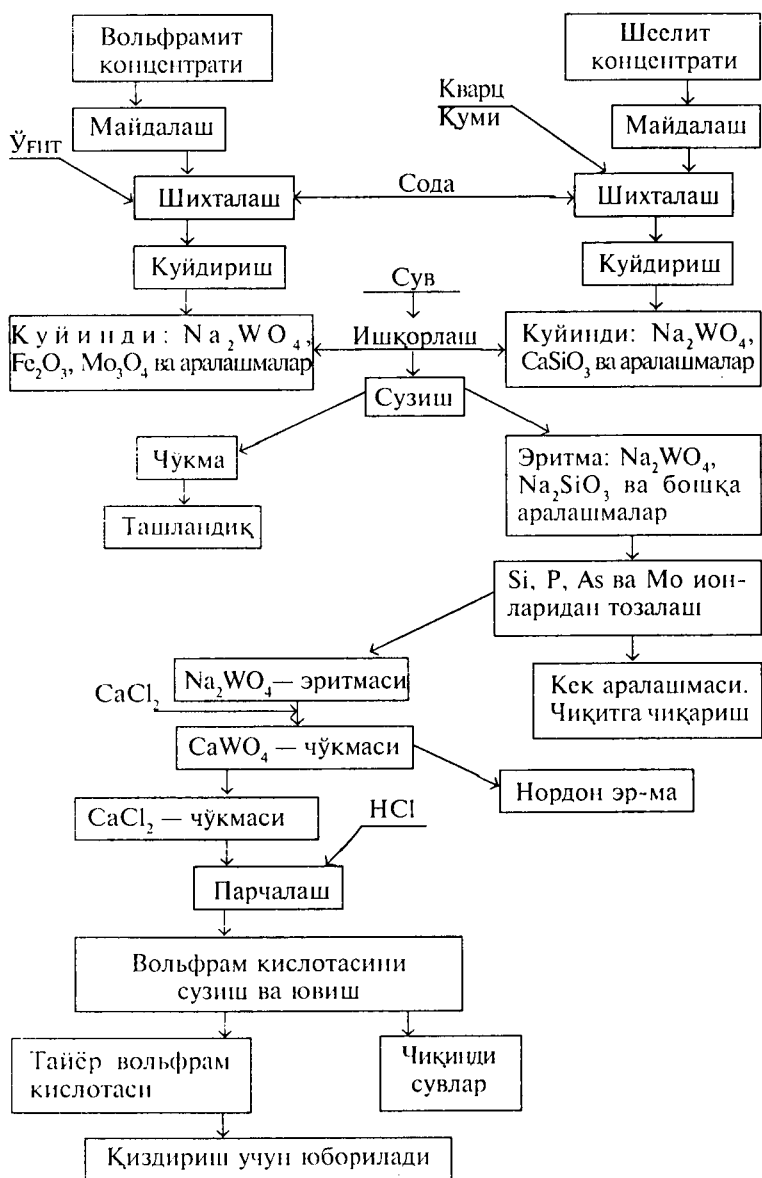
21-расм. Вольфрамит еки шеслитнинг содали куйдириш технологияси.
