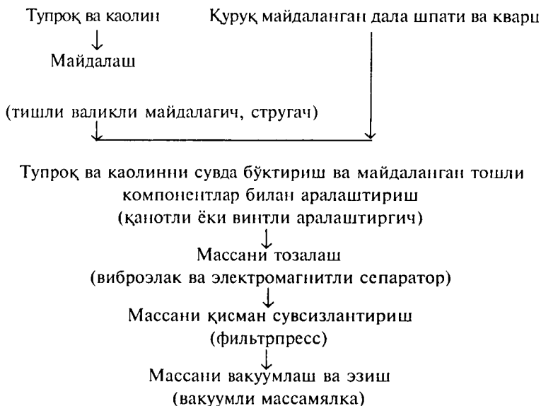
5- расм. Пластик массани қукунланган тошсимон материаллардан фойдаланган ҳолда тайёрлаш схемаси.
