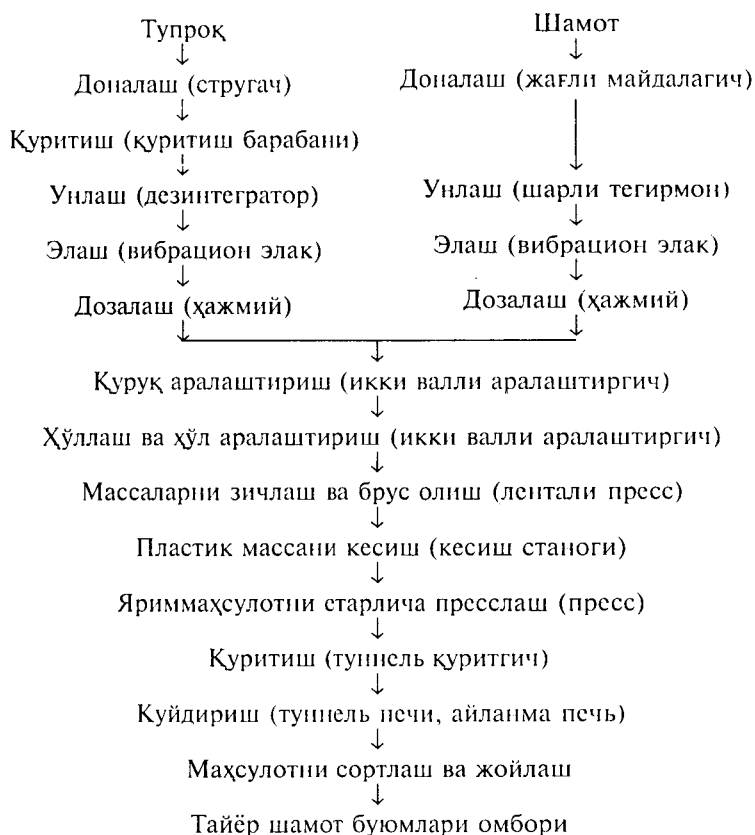
6- расм. Пластик прессилаш усулида шамот гишти олишнинг технологик схемаси.
