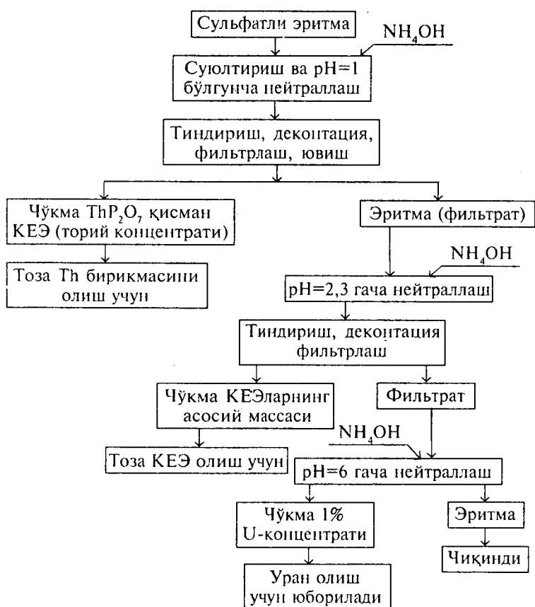
45-расм. Босқичли нейтраллаш усули билан сульфатли эритмаларни қайта ишлаш схемаси.
